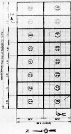
แปลนแผงเซลล์พลังงานแสงอาทิตย์ขนาดไม่น้อยกว่า 600 วัตต์ NOT TO SCALE
