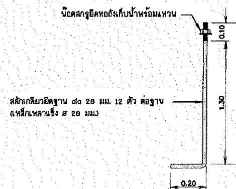
แบบขยายสลักเกลียวยึดฐาน
