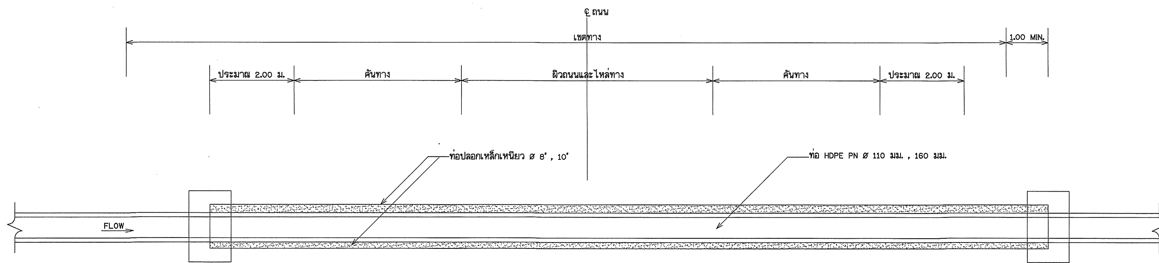
แปลนท่อลอดถนน มาตราส่วน 1:100
