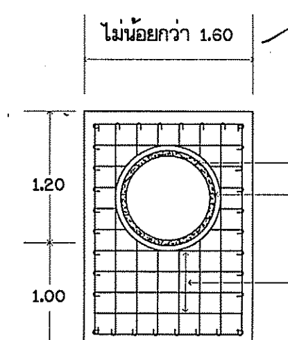
ขยายการเสริมเหล็กกำแพงปากท่อและท้ายท่อ (HEAD WALLS) ไม่แสดงมาตราส่วน
