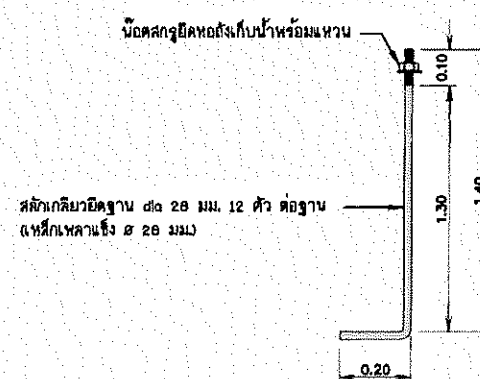
แบบขยายหลักเกิลียวียิตฐาน
