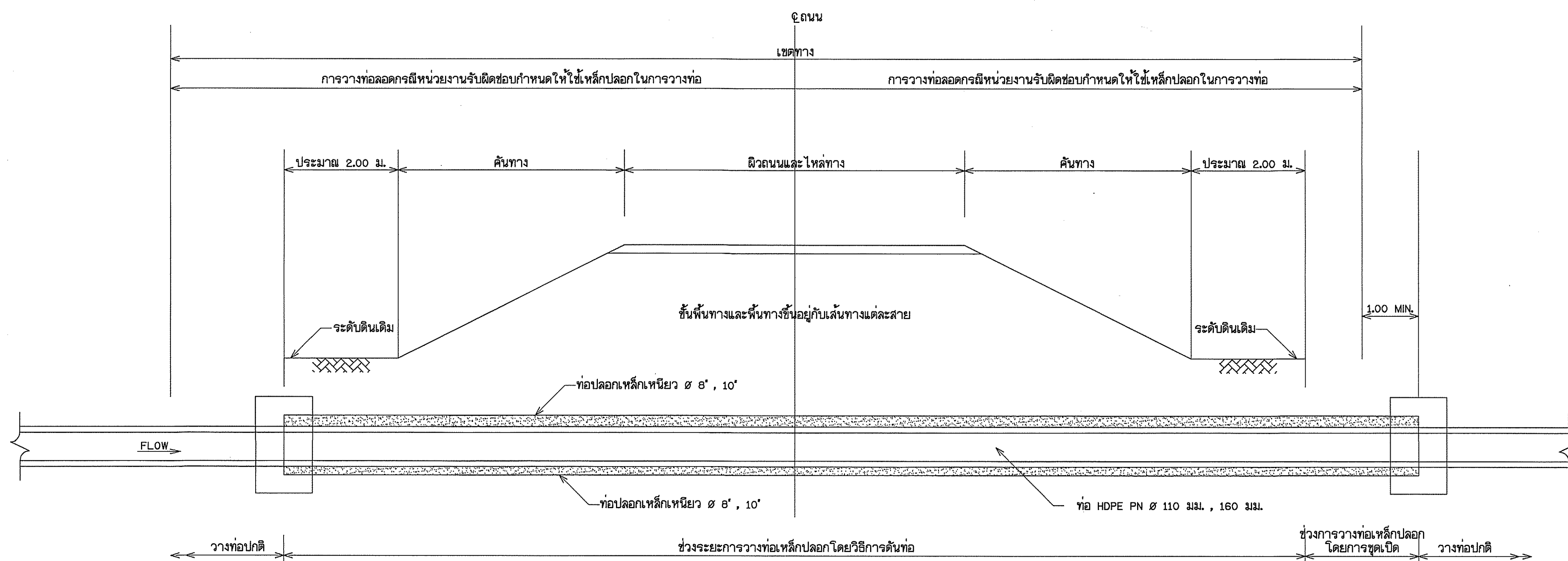
แสดงการวางท่อลอดใต้ผิวจราจร มาตราส่วน 1:100
