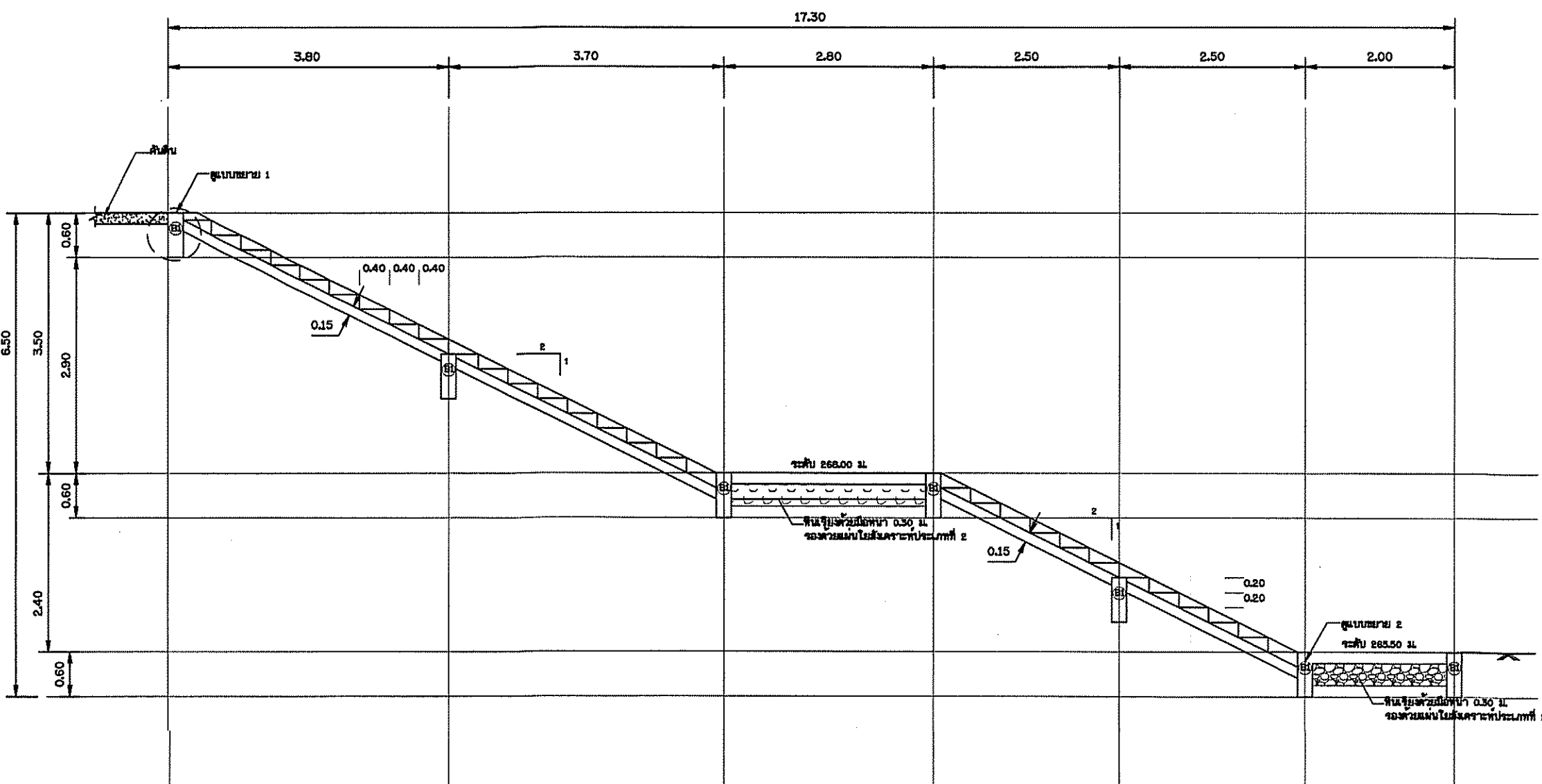
แนวตัด A-A มาตราส่วน 1 : 100
