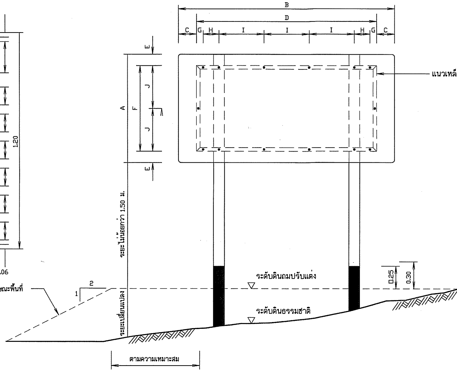
รูปแสดงการประกอบแผ่นป้าย มาตรฐาน 1120
