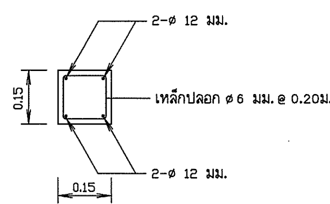
รูปตัด ก - ก มาตรฐาน 1110
