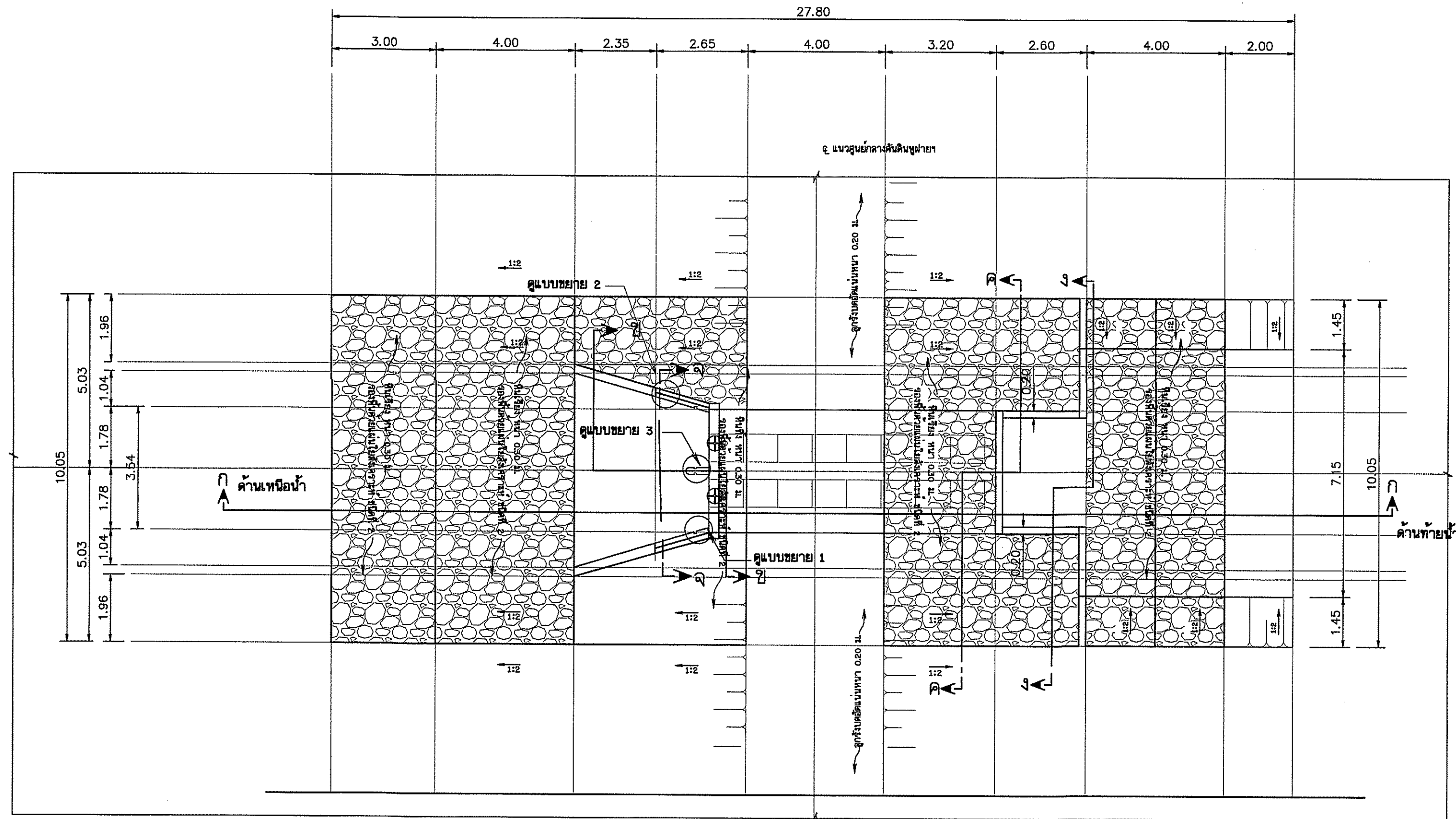
แปลนอาคารบังคับน้ำแบบทอกลม ท่อ 2 แถว (สำหรับฝายน้ำล้น) มาตราส่วน 1:100
