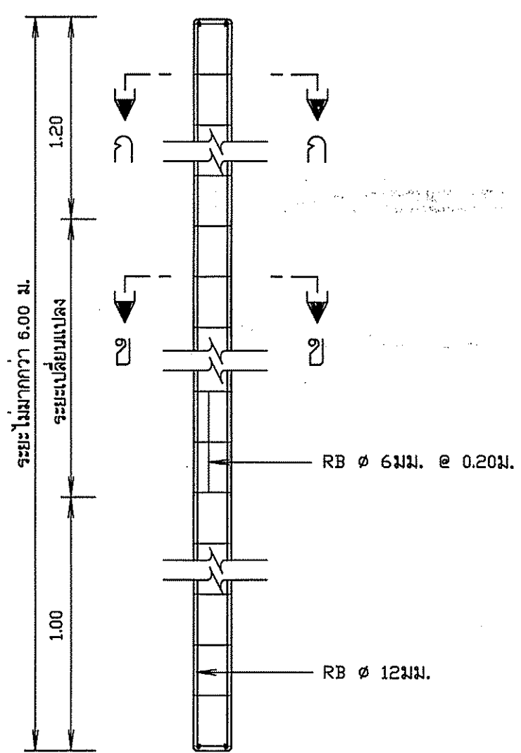
รายละเอียดเสาป้าย คสล. มาตรฐาน 1120
