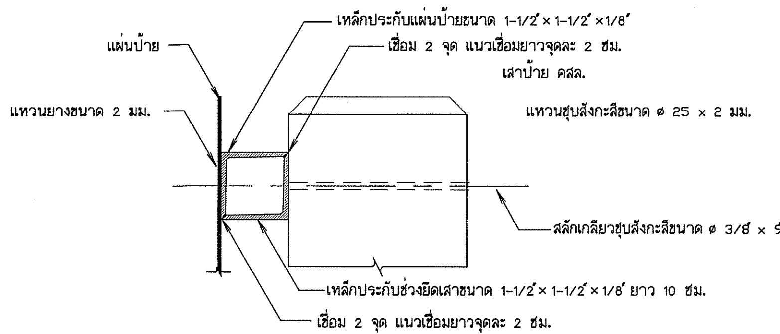
รูปตัดขยายการยึดแผ่นป้ายและเสา มาตรฐาน 1120
