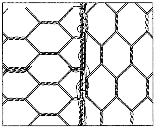
รูปที่ 2 วิธีการผูกยึดกล่องลาดตาข่าย
