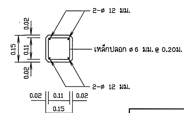
รูปตัด ข - ข มาตรฐาน 1110
