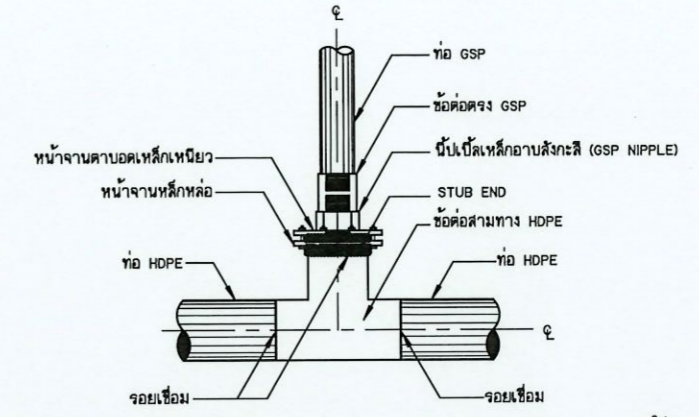
การบรรจุท่อสามทาง HDPE กับท่อ GSP แบบข้อต่อ (สำหรับอาคารจุดปล่อยน้ำ อาคารประจวบทยตะกอน อาคารท่อระบายอากาศ กรณีที่ท่อส่งน้ำขนาดเส้นผ่าศูนย์กลางมากกว่า 315 มม.)
