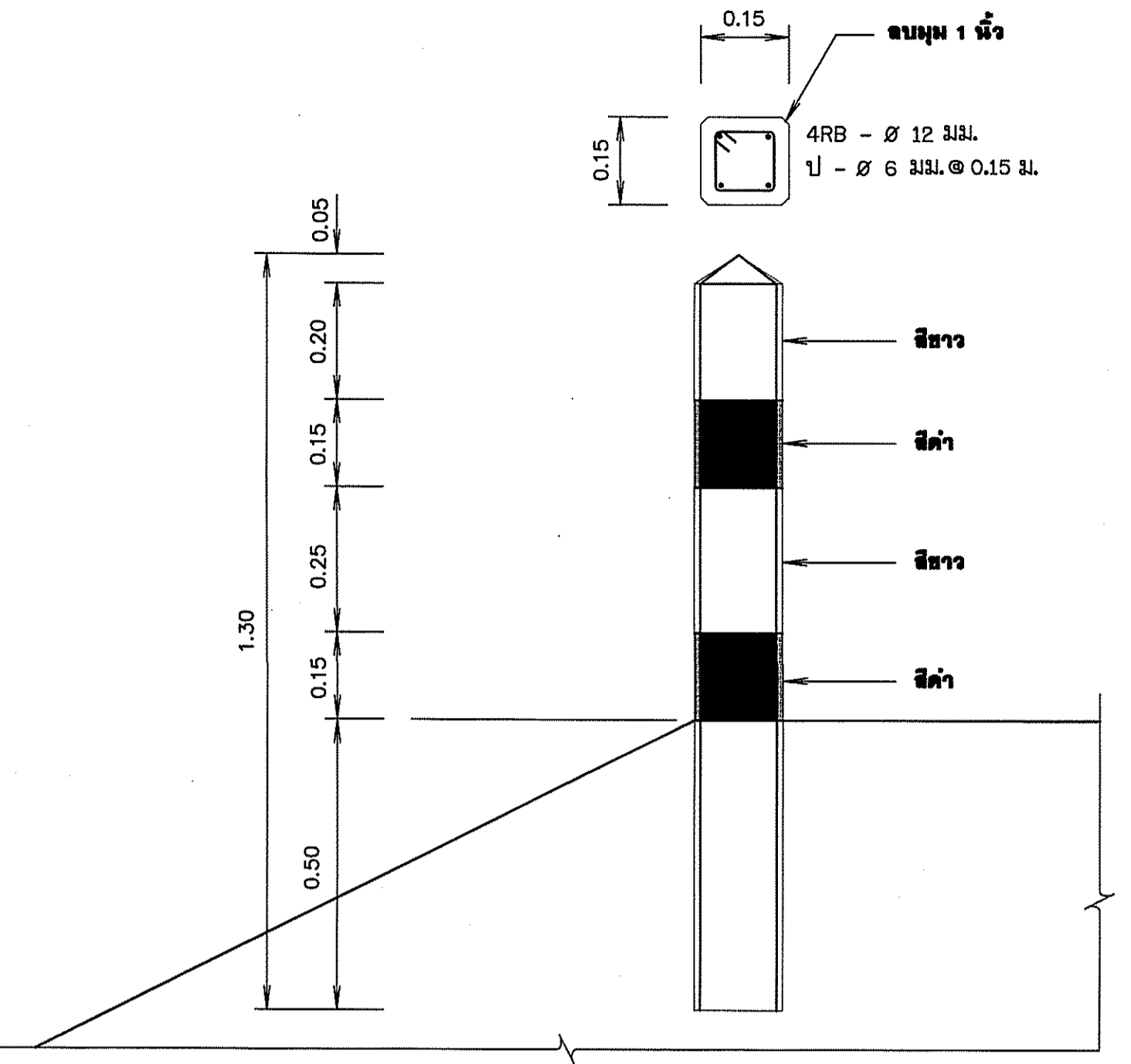
แบบขยายหลักirimคันดิน ไม่แสดงมาตราส่วน
