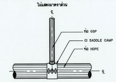
การบรรจุท่อสามทาง HDPE กับท่อ GSP แบบ CI SADDLE CLAMP (สำหรับอาคารจุดปล่อยน้ำ อาคารประจวบทยตะกอน อาคารท่อระบายอากาศ กรณีที่ท่อส่งน้ำขนาดเส้นผ่าศูนย์กลางน้อยกว่าหรือเท่ากับ 315 มม.)
