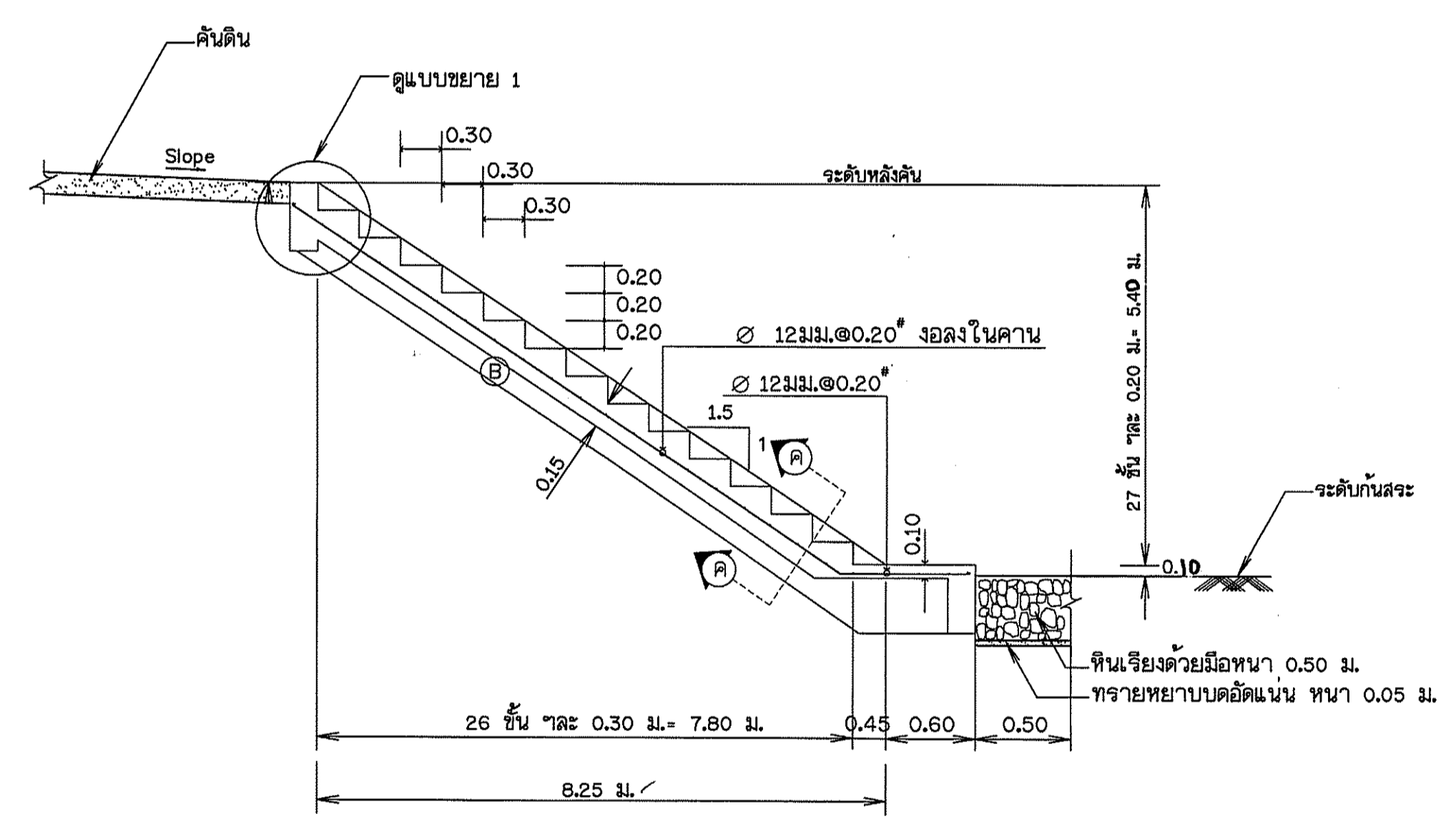
แปลนบันได คสส. แบบไม่มีชันพิก
