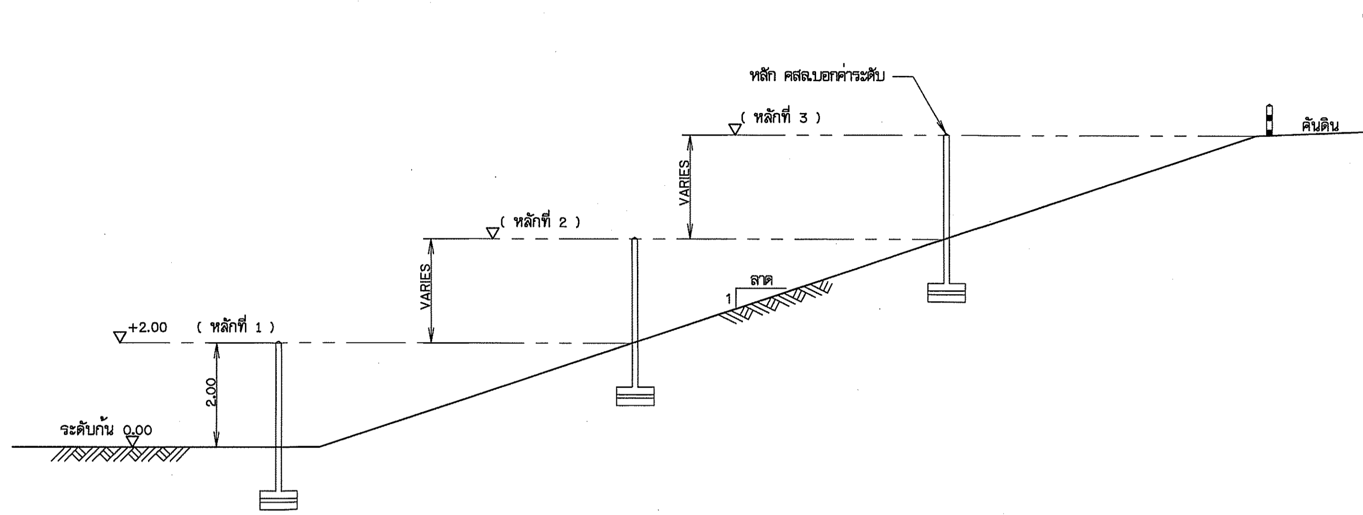
รูปตัดทั่วไปแสดงตำแหน่งหลักบอกค่าระดับน้ำ ไม่แสดงมาตราส่วน
