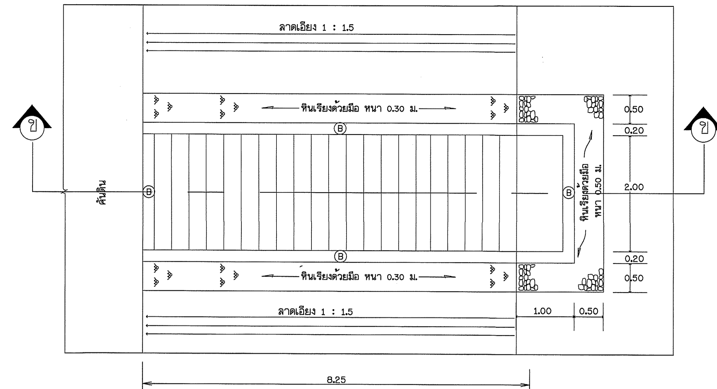
แปลนบันได คสส. แบบไม่มีชันพิก
