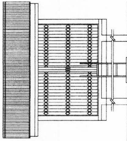
รูปด้านหน้า 1 : 50
