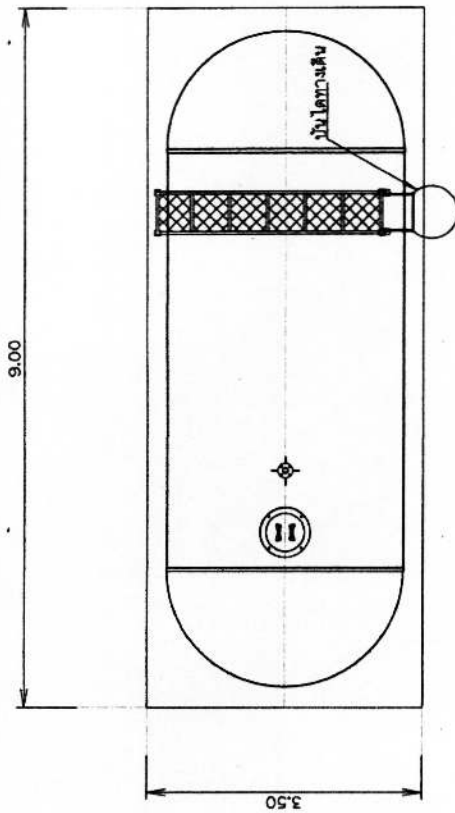
แปลนฐานราก ไม่ตอกเข็ม
