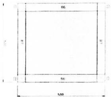
แปลนคานายึด ขนาด 87 x 95
