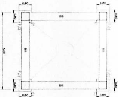
แปลนฐานรากคานคดขึ้น ขนาด 500 x 500
