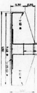
รูปตัด ก - ก มาตราส่วน 1:100
