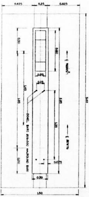
รูปตัด ข - ข มาตราส่วน 1:100
