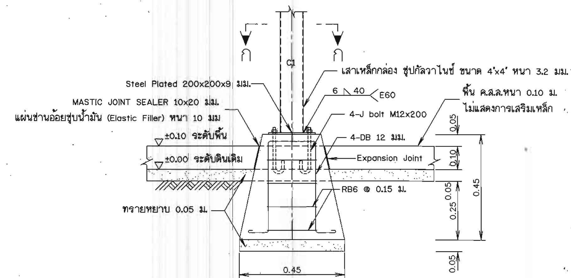
รูปขยายฐานรากโครงสร้างรับแผง F1 (ตาม คสล. ท่อสำเร็จรูปพร้อมติดตั้ง) ไม่แสดงมาตราส่วน
