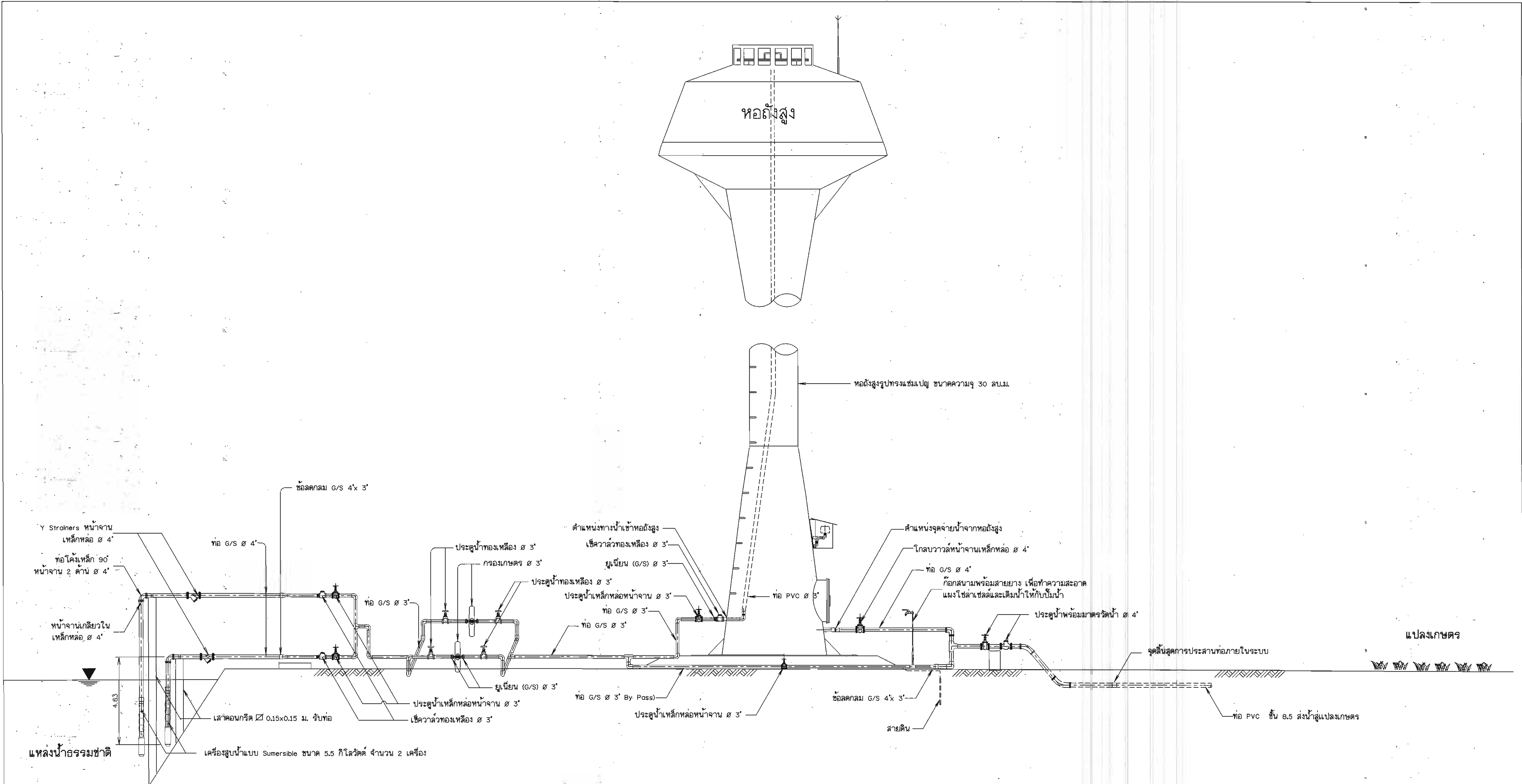
รูปแสดงรายละเอียดท่อและอุปกรณ์ระบบส่งจ่ายน้ำพลังงานแสงอาทิตย์ ไม่แสดงขนาดบางส่วน
