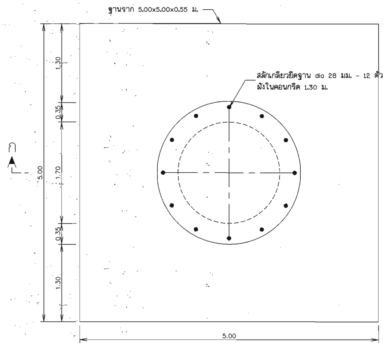
แปลน ฐานรากหochtงสูง (แบบฐานแผ่)
