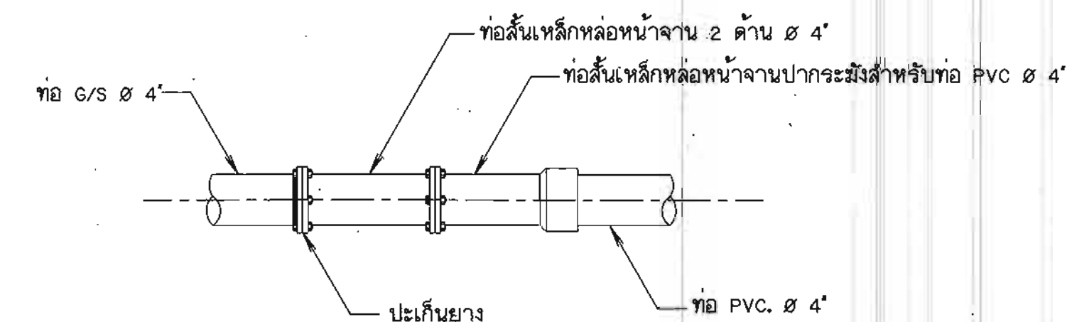
8. การบรจพบท่อเหล็กอาบสังกะสี G/S กับท่อ PVC. ไม่แสดงมาตราส่วน
