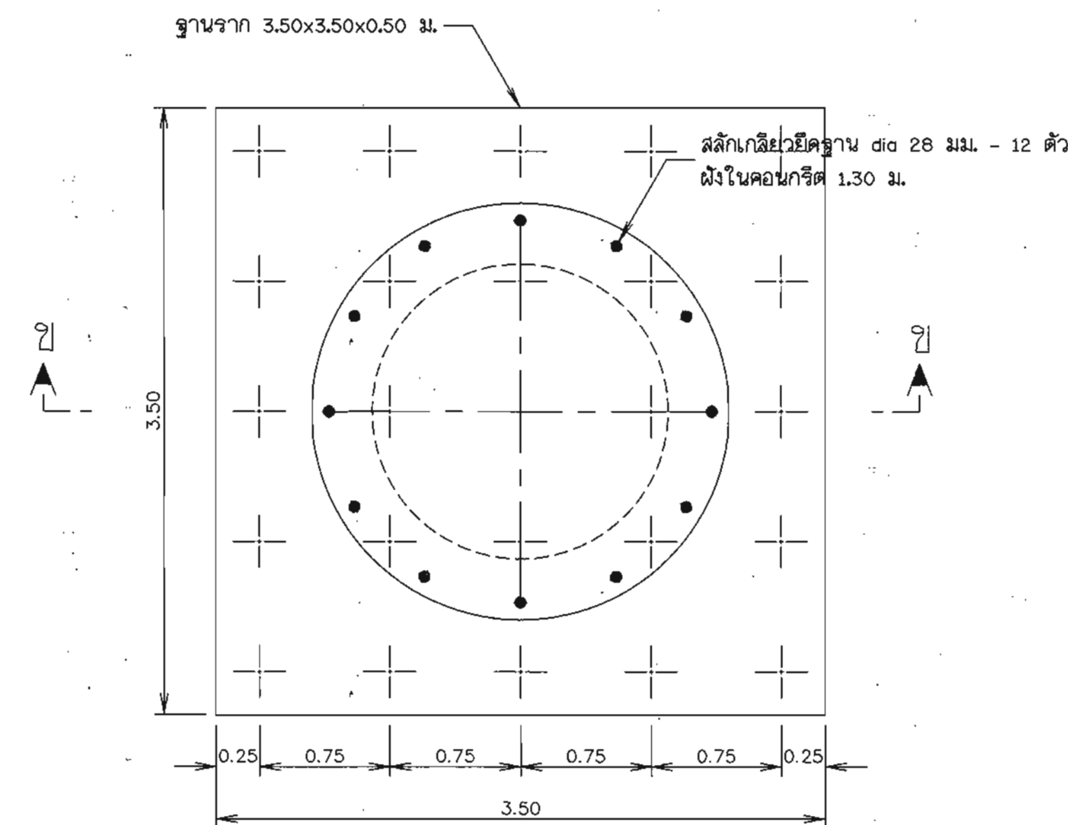
แปลน ฐานรากหochtงสูง (แบบเสาเข็ม)
