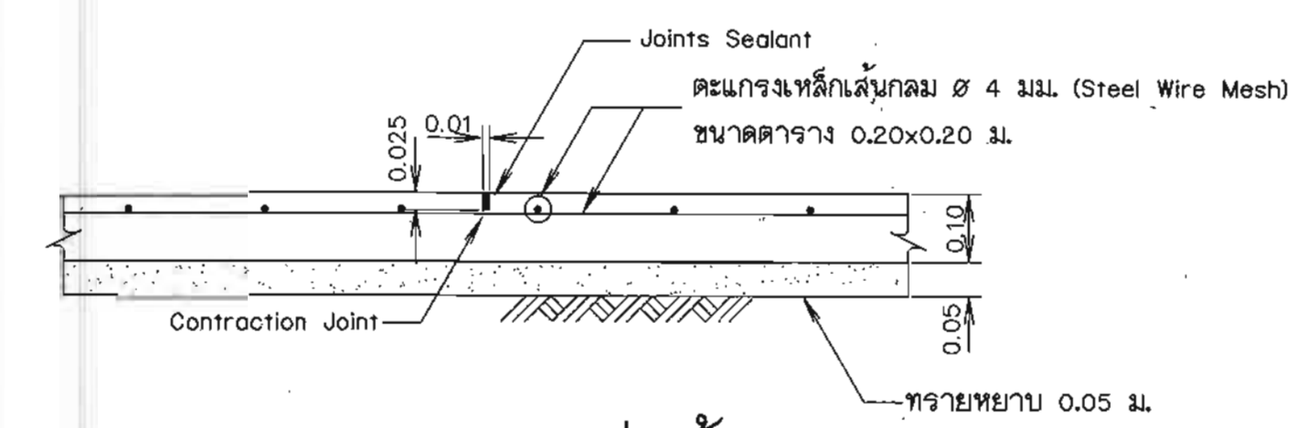
แบบขยายรอยต่อพื้น (Contraction Joint) ไม่แสดงขนาดราวล้วน
