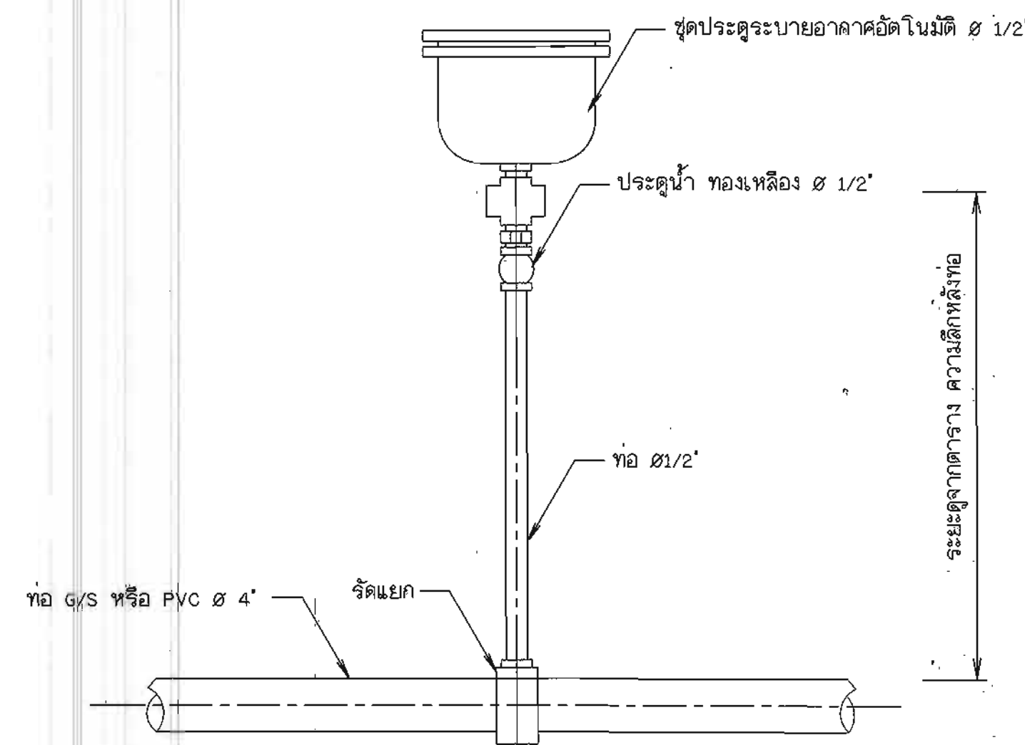
12. การติดตั้งประตูปะบายอากาศอัดไนเมติ ไม่แสดงมาตราส่วน
