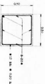
เสา C1
