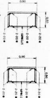
รูปตัด 5-5
