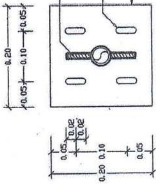
แผ่นเหล็กบนเสาด้าน FREE 1:5
