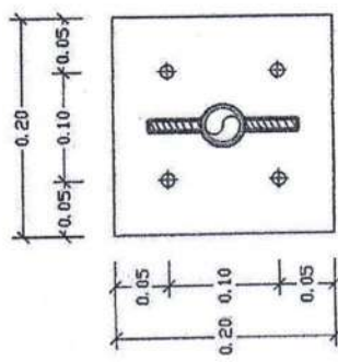
แผ่นเหล็กบนเสาด้าน FIXED 1:5
