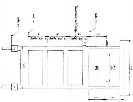
รูปตัด (3) ขนาดหน้าตัด 1175
