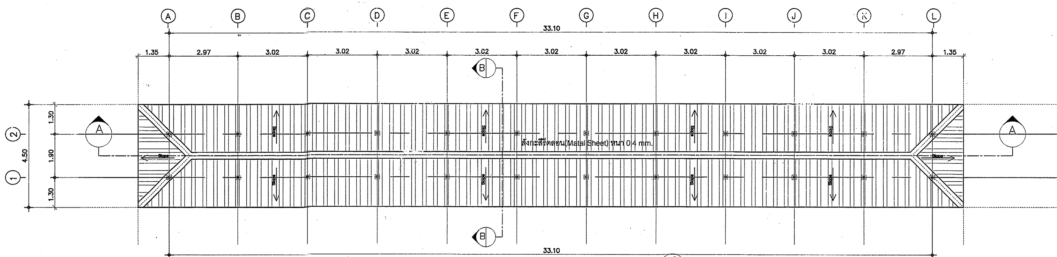
แปลนหลังคา
