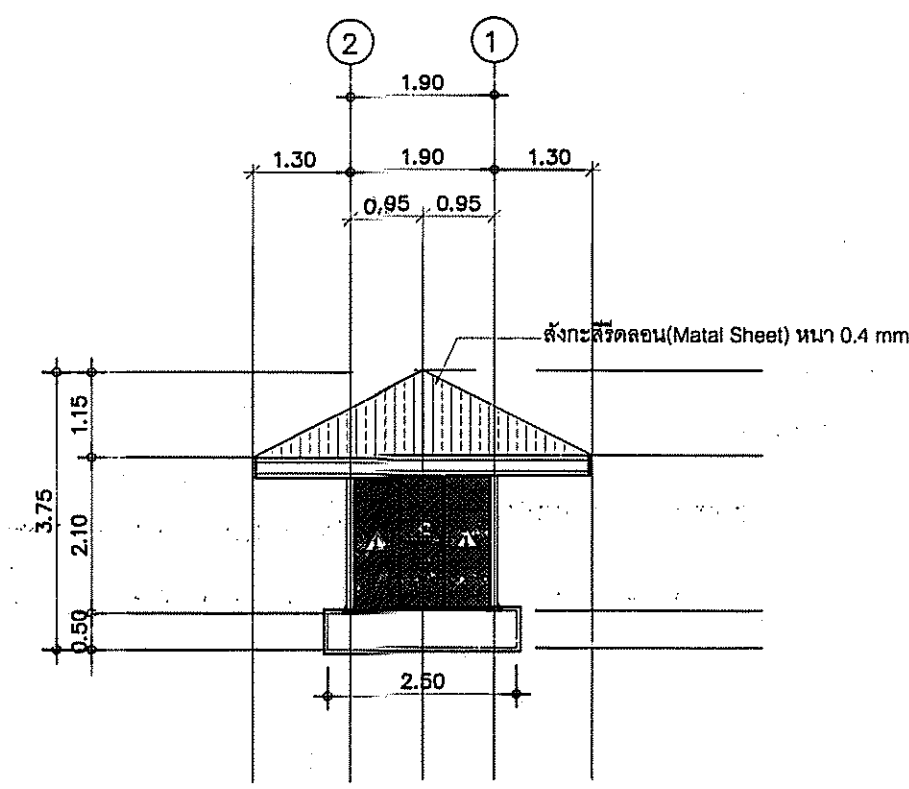
รูปด้านขวา
