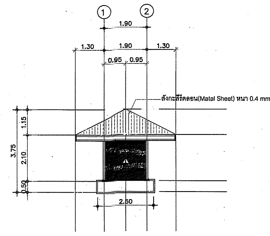
รูปด้านซ้าย
