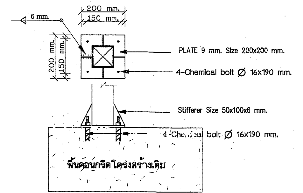
ขยาย Plate ยึดเสา
