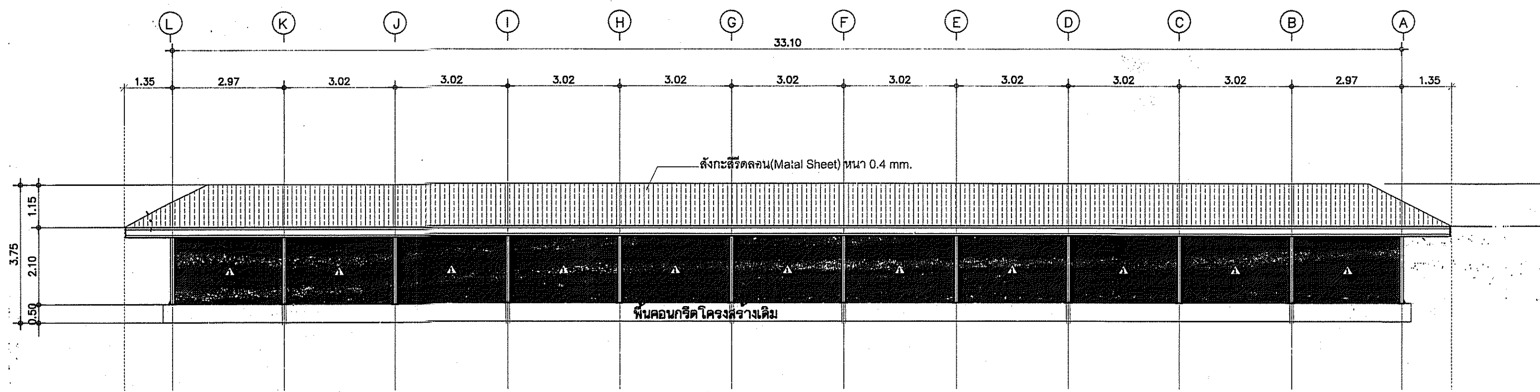
รูปด้านหลัง
