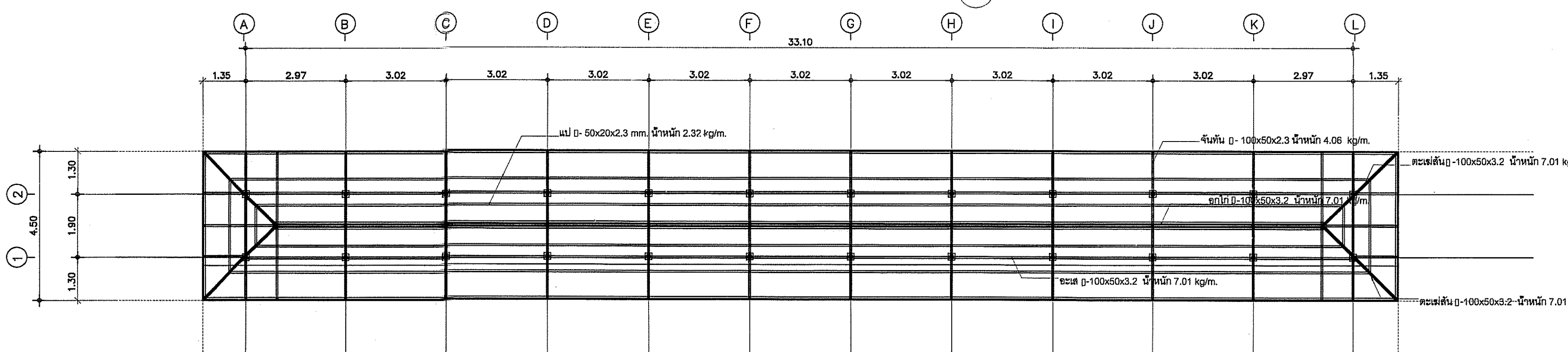
แปลนโครงสร้างหลังคา
