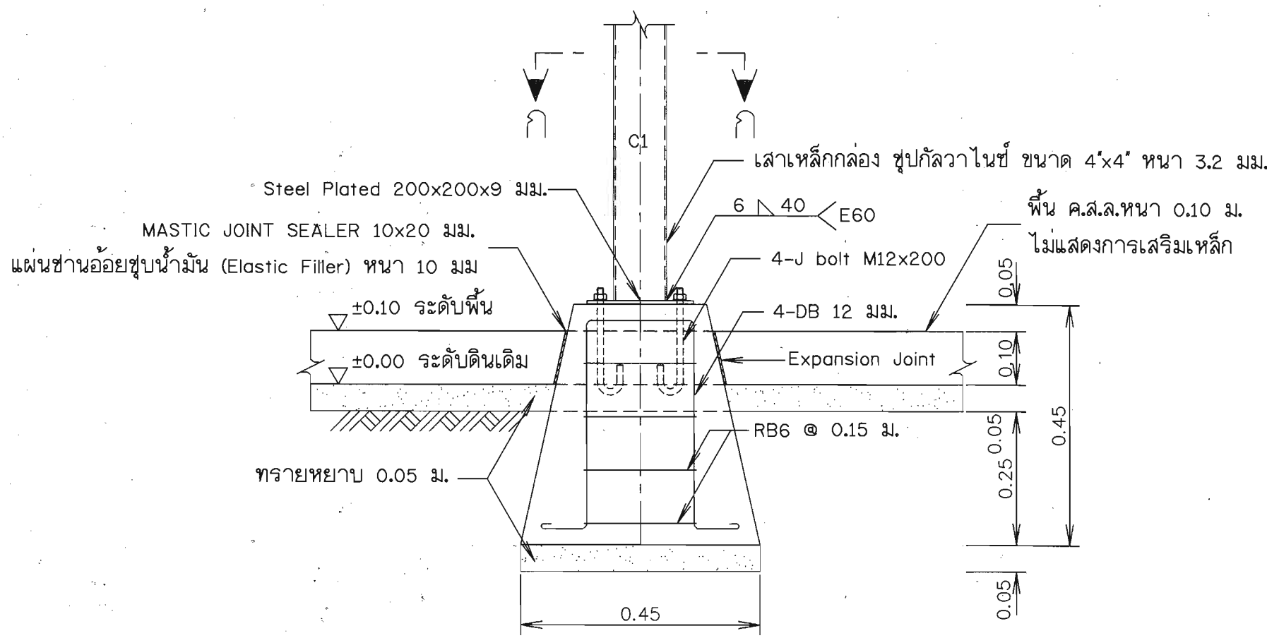
รูปขยายฐานจากโครงสร้างรับแผง F1
