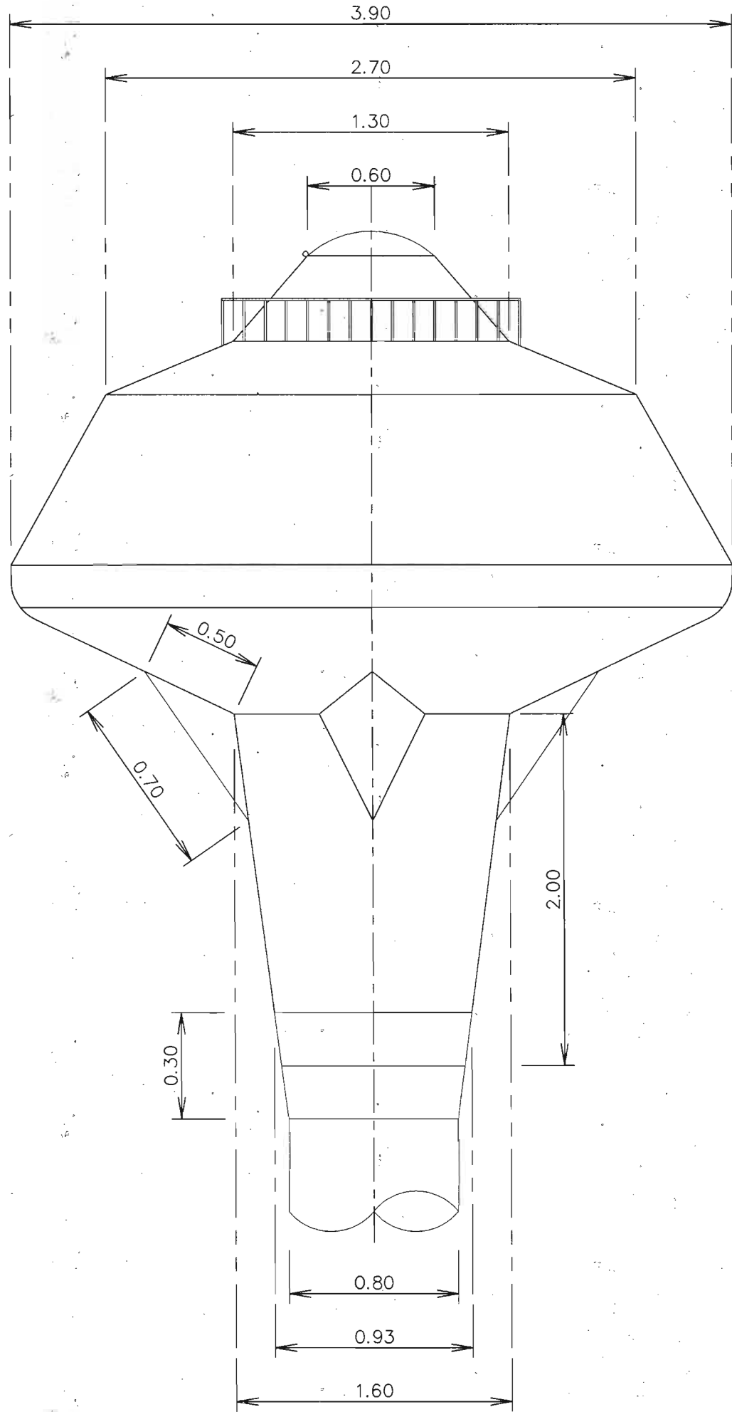
แบบขยายแมนโฮลบนหอลังสูง
