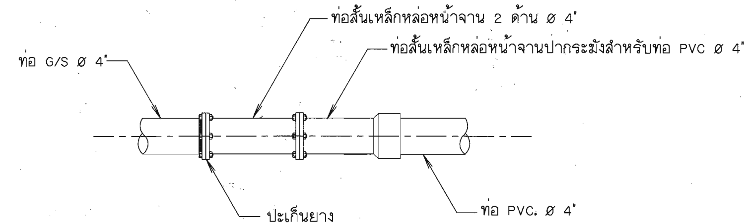
8. การบรรจบท่อเหล็กอบสังกะสี G/S กับท่อ PVC. ไม่แสดงมาตราส่วน
