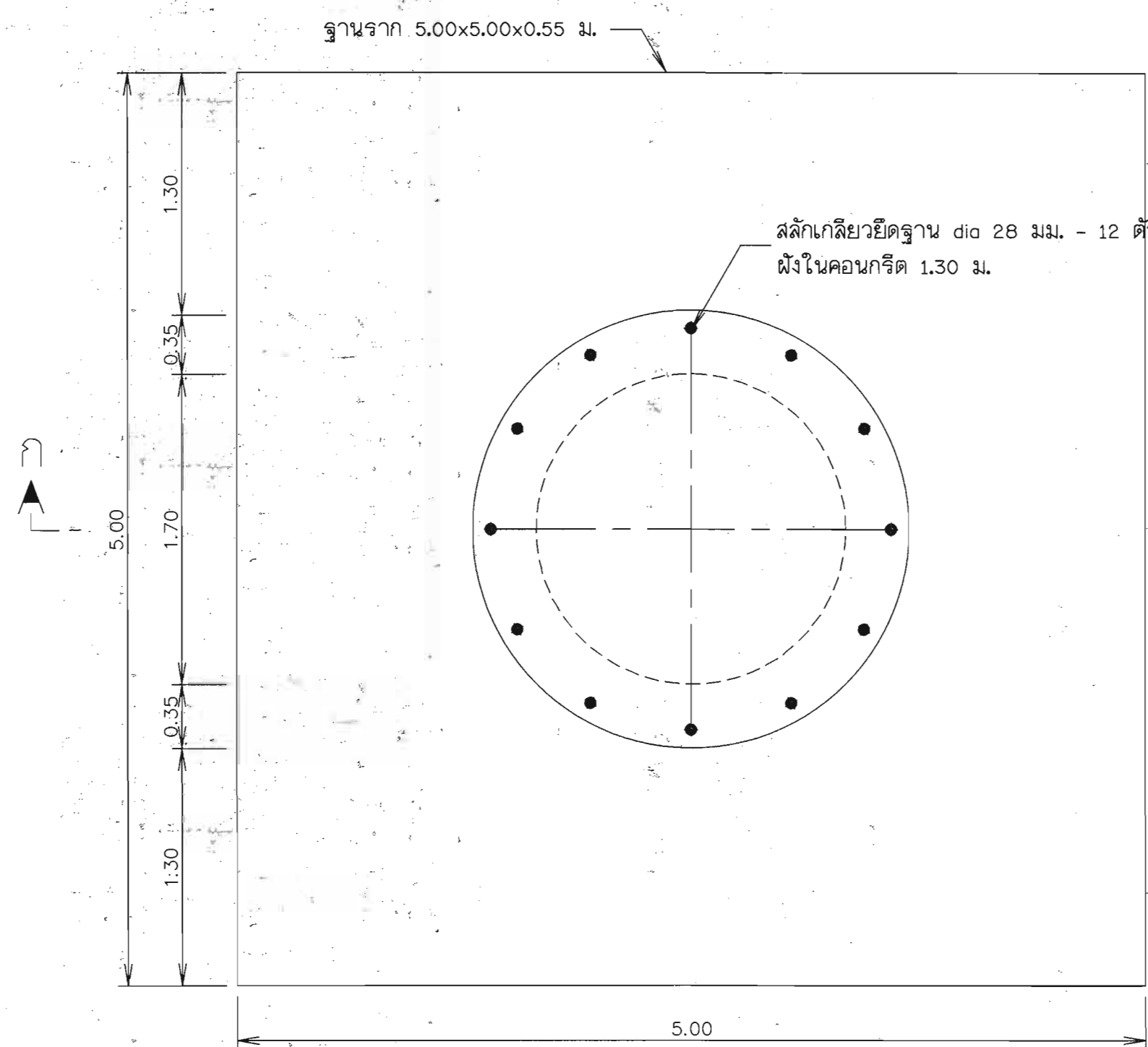
แปลน ฐานรากหอดึงสูง (แบบฐานแฉ่ง)
