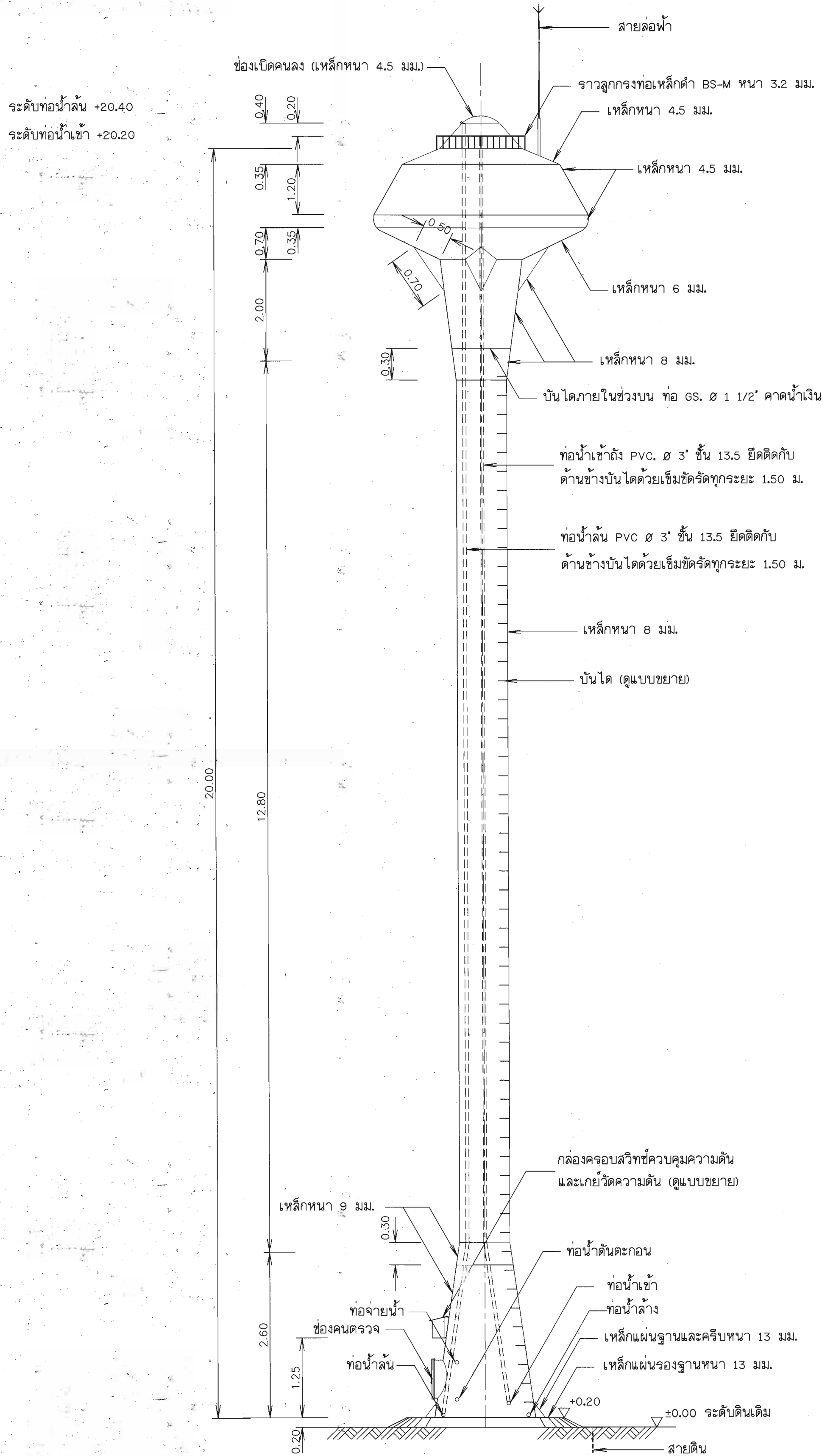
รูปด้านข้างหอลังสูง แบบถังเหล็กรูปทรงแปมแปญ
