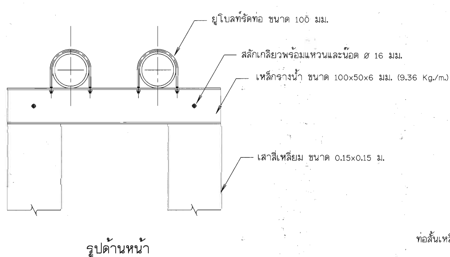
13. เสาดมอรับท่อชุด และแบบขยายอุปกรณ์รัดท่อ ไม่แสดงมาตราส่วน
