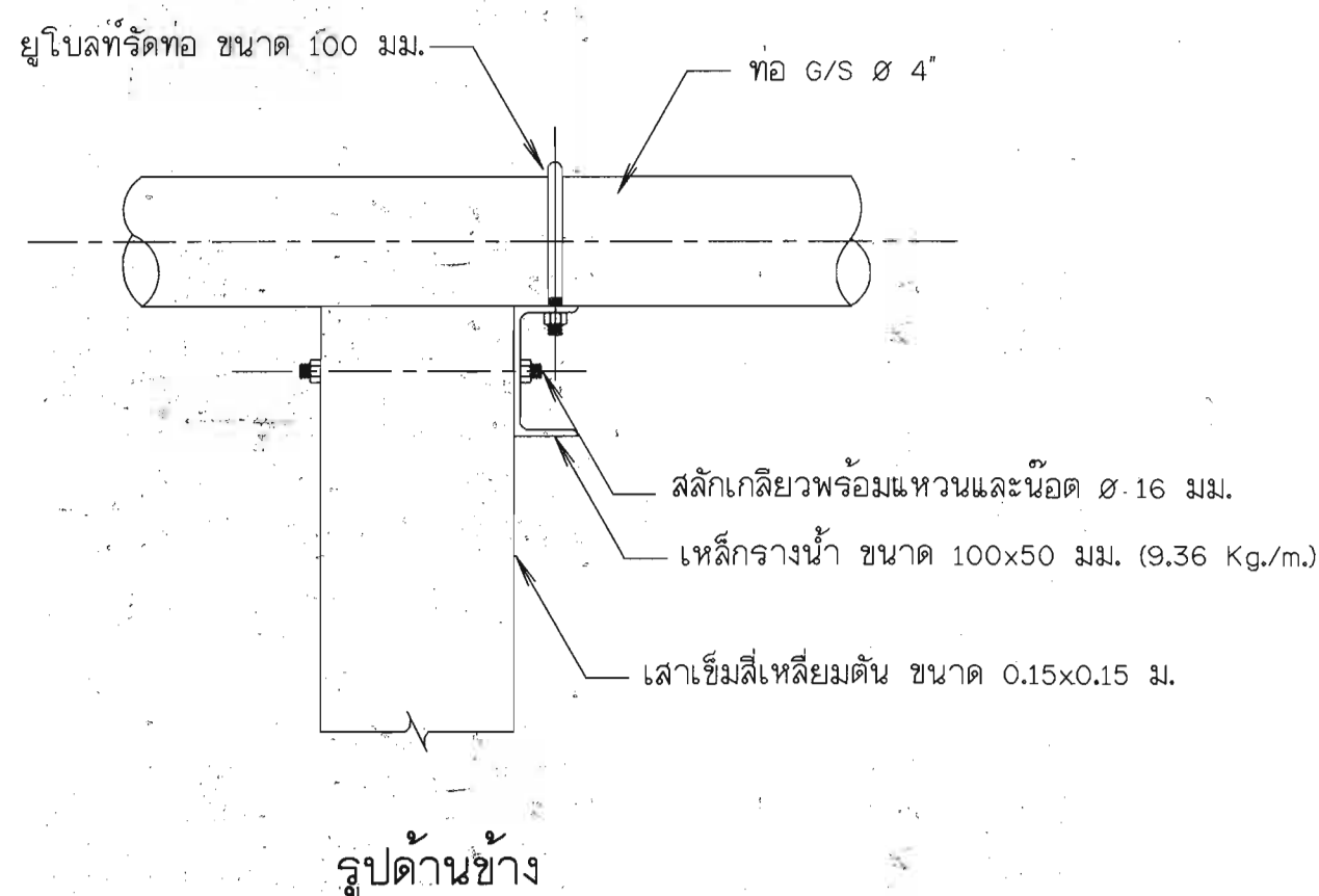
13. เสาดมอรับท่อชุด และแบบขยายอุปกรณ์รัดท่อ ไม่แสดงมาตราส่วน
