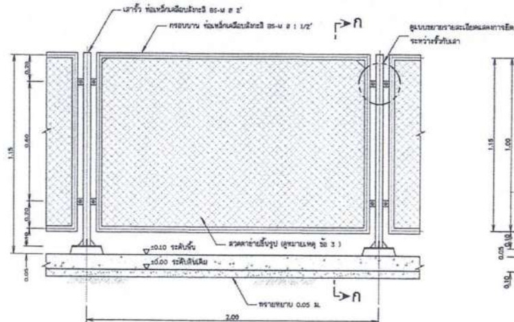
แบบขยายรู้ลวดตาข่าย ใบแสดงมาตรฐาน
