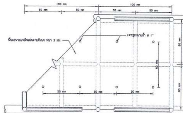
แบบขยายโครง พื้นสะพาน
