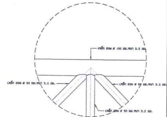
รูปขยาย 2
