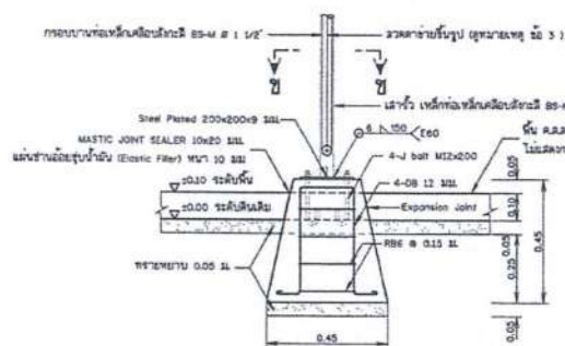
รูปขยายฐานรากโครงสร้างรับแผง F1 (ตาม A-11 ทิศใต้รูปหน้าตัดจริง) โมดูลมาตรฐาน
