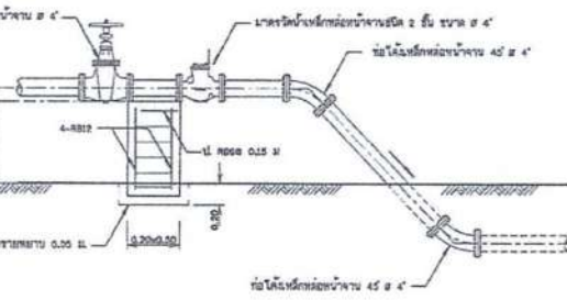
14. การติดตั้งมาตรวัดน้ำบนพื้นดิน ๔" ไม่แสดงมาตราส่วน
