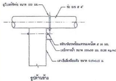
13. เสาคอมม่อรับท่อตัด และแบบขยายอุปกรณ์รัดท่อ ไม่แสดงมาตราส่วน
