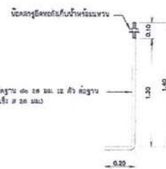
แบบขยายหลักเกลียวยึดฐาน
