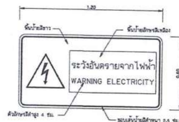
ป้ายเตือนกระแสไฟฟ้า
