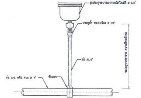
12. การติดตั้งประตูละบายอากาศอัด โนมิต ไม่แสดงมาตราส่วน
