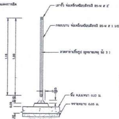
รูปตัด ก-ก โดยสมมาตรด้าน
