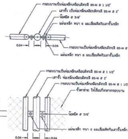
แบบขยายรายละเอียดแสดงการยึดระหว่างรั้วกับเสา
