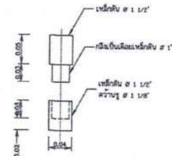
แบบขยายบานพับนุ้หลัก
