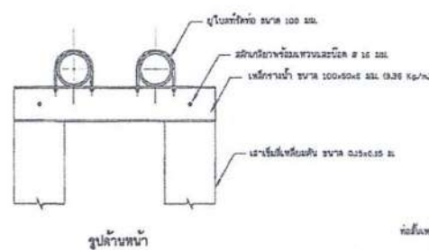
13. เสาคอมม่อรับท่อตัด และแบบขยายอุปกรณ์รัดท่อ ไม่แสดงมาตราส่วน
