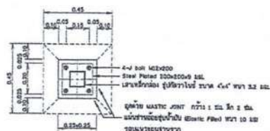
รูปตัด ก-ก
