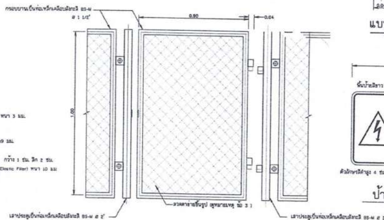
แบบขยายรายละเอียดประตู
