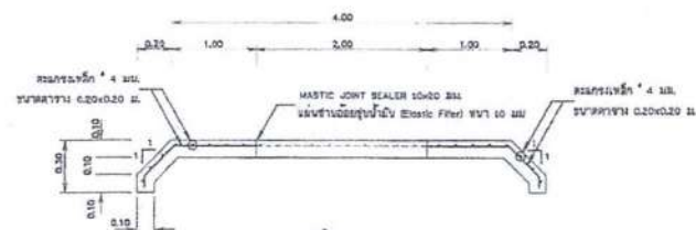
รูปตัด ค-ค
