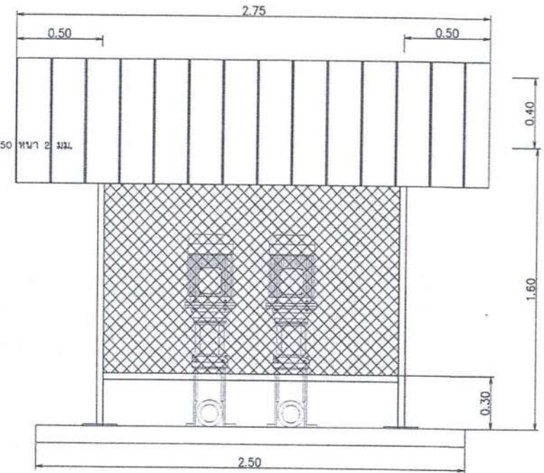
รูปด้านข้าง 2
