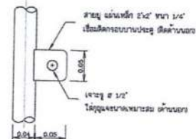
แบบขยายสายขุม โมดูลมาตรฐาน
