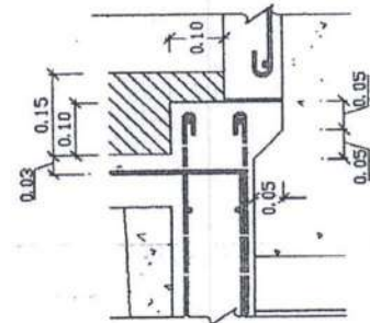
ขยายขอบพื้น 1:10
