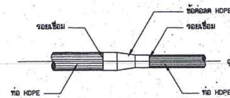
การบรรจุท่อ HDPE กับข้อต่อท่อ HDPE ไม่แสดงขนาดราส่วน
