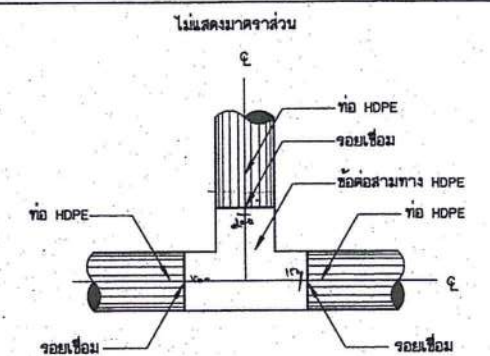
การบรรจุท่อสามทาง HDPE กับท่อ HDPE ไม่แสดงขนาดราส่วน
