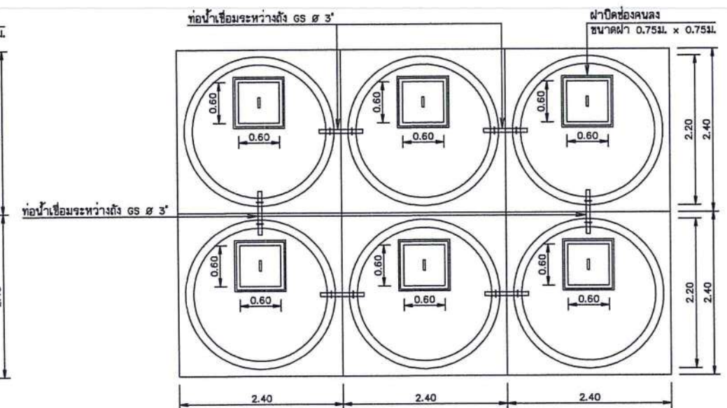
แปลนแบบ 6 ถึง มาตราส่วน 1:40
