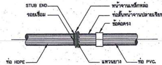
การบรรจุท่อ HDPE กับท่อ PVC. ไม่แสดงขนาดราส่วน
