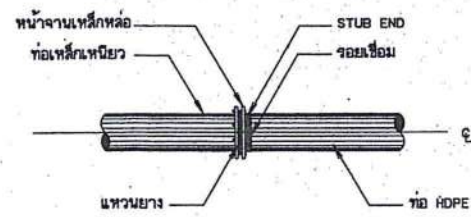
การบรรจุท่อเหล็กเหนียวกับท่อ HDPE ไม่แสดงขนาดราส่วน
