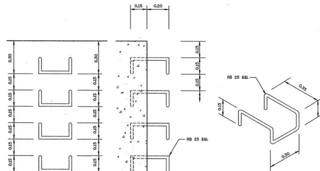
รูปขยายบันไดลิง
