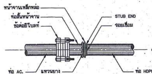
การบรรจุท่อ AC กับท่อ HDPE ไม่แสดงขนาดราส่วน
