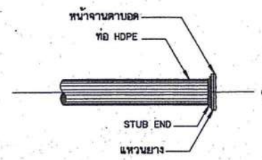
การปิดปลายท่อ ไม่แสดงขนาดราส่วน
