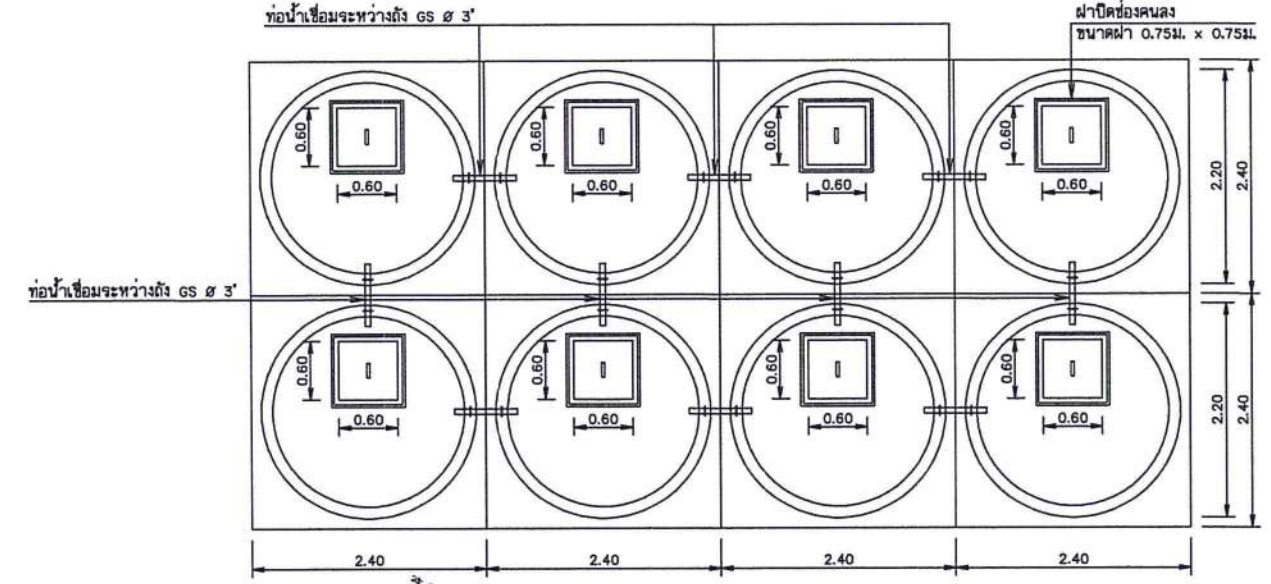
แปลนแบบ 8 ถัง มาตราส่วน 1:40
