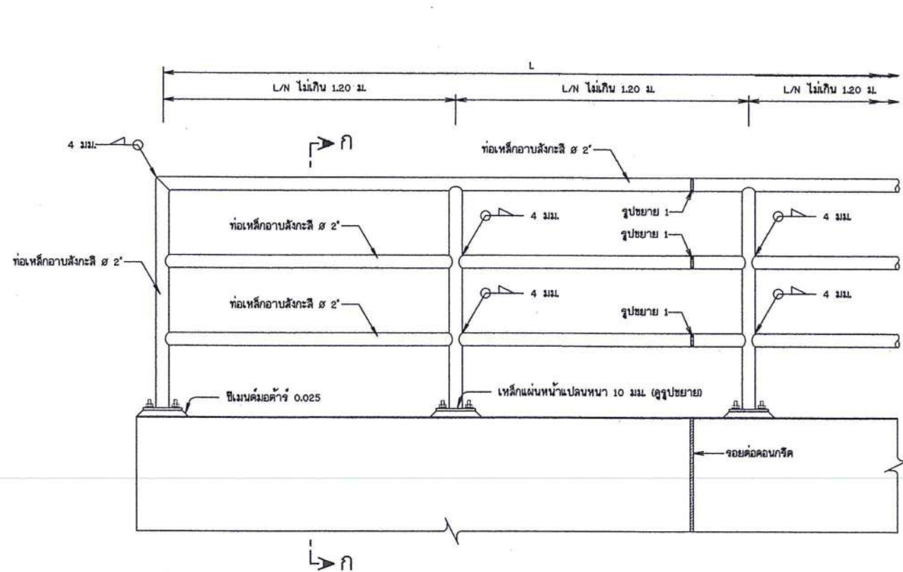
รูปขยายราบเหล็กกันคก
