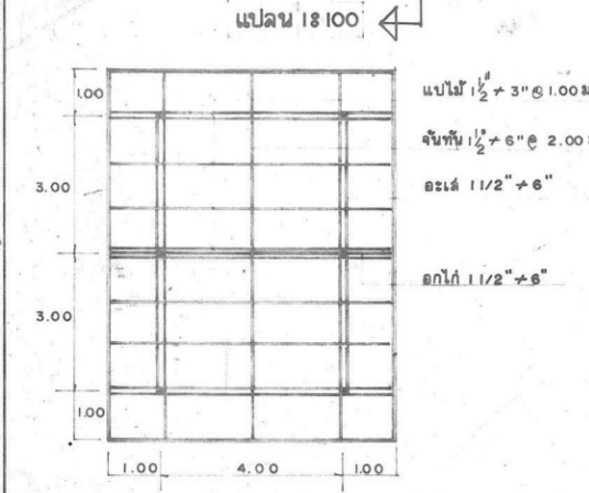
แปลนโครงหลังคา 18100
