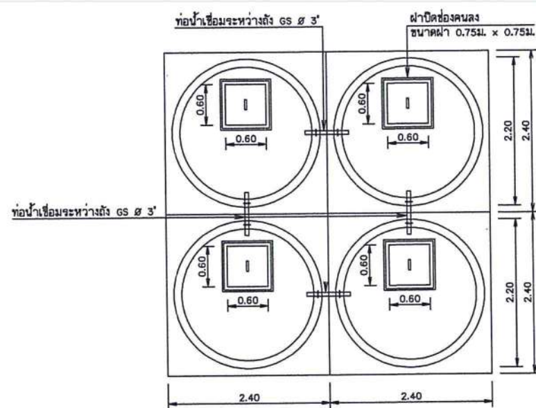
แปลนแบบ 4 ถึง มาตราส่วน 1:40
