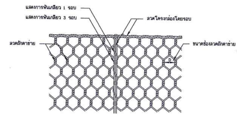
รูปแสดงการพันลวดระหว่างกล่องลวดตาข่ายและฟาปิด
