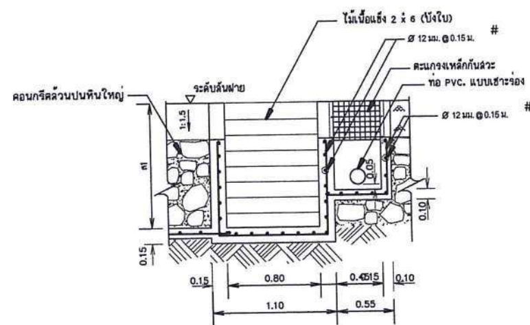
รูปตัด ฉ - ฉ ขนาดจั่ว 1:25
