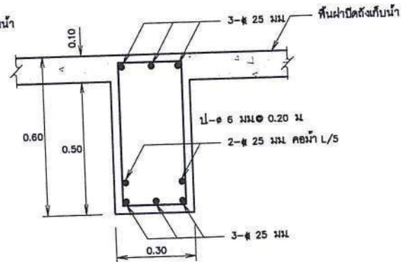
เสริมเหล็กคานแบบที่ ② มาตราส่วน 1:10
