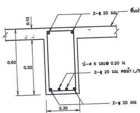
เสริมเหล็กคานแบบที่ ① มาตราส่วน 1:10
