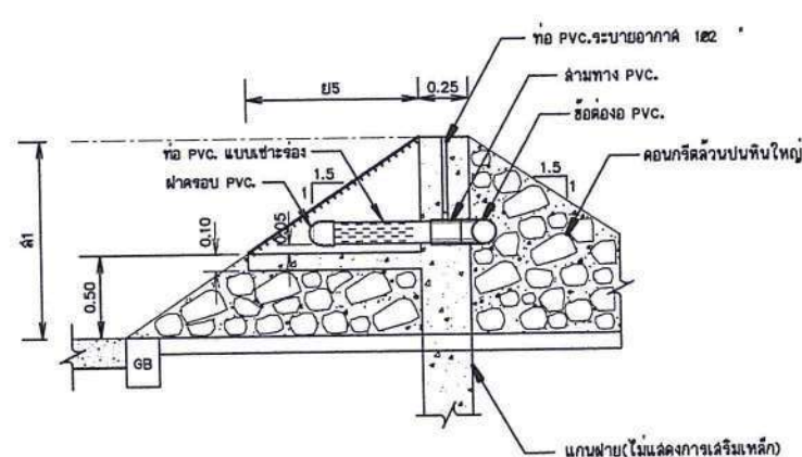
รูปตัด ช - ช ขนาดจั่ว 1:25
