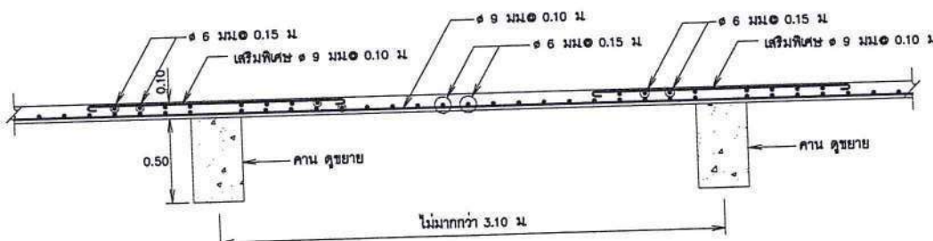
ขยายการเสริมเหล็กพื้นผิวดังเก็บน้ำ มาตราส่วน 1:20
