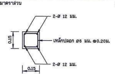
รายละเอียดเสาป้าย คสล. มาตราส่วน 1:20
