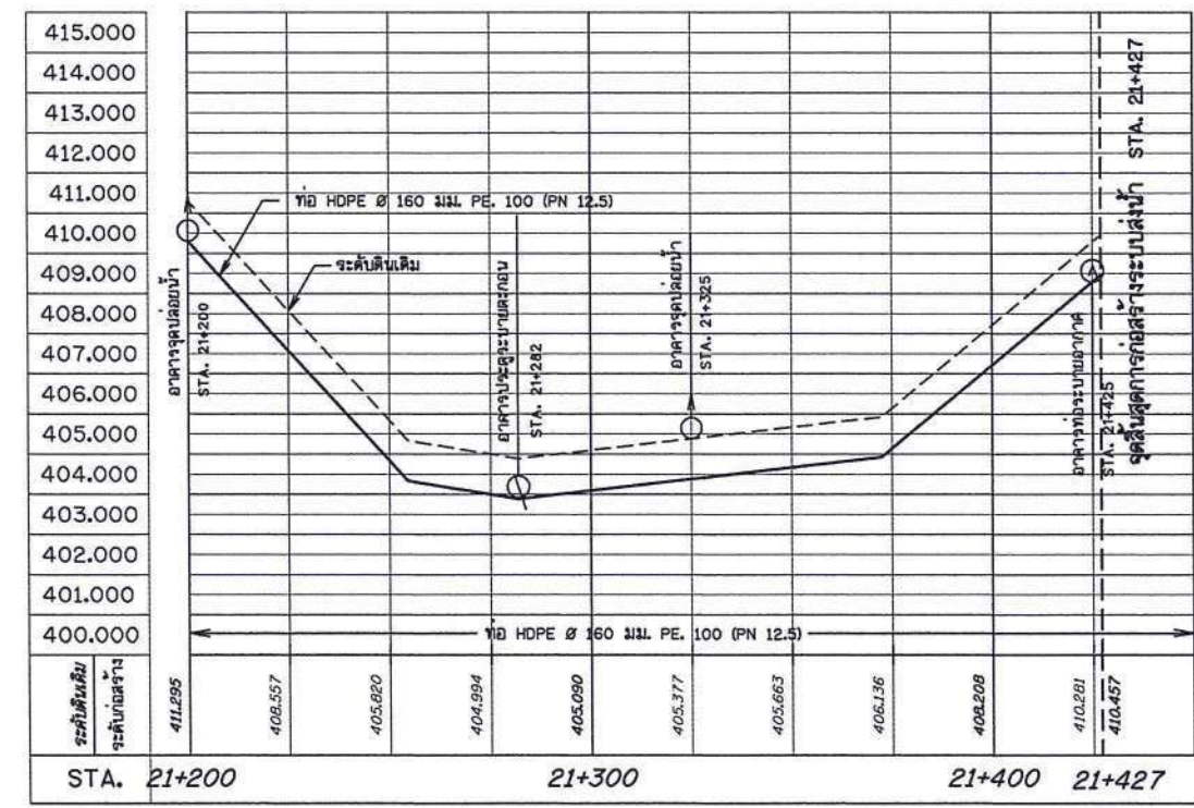
รูปตัดตามแนวยาว STA. 21+200 - 21+427 แนวตั้ง 1:200 แนวนอน 1:1,000
