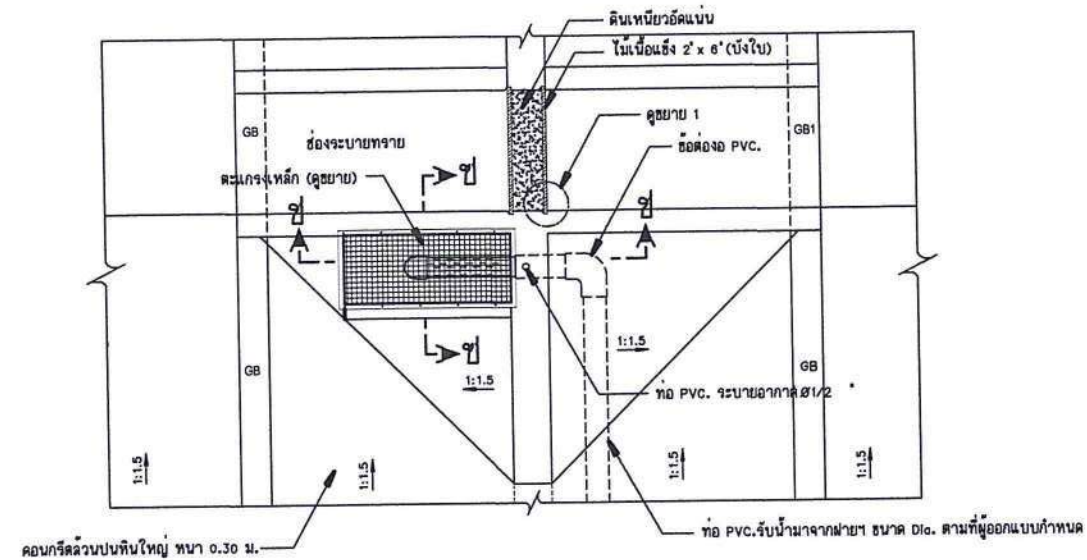
แปลนอาคารรับน้ำ ขนาดจั่ว 1:25
