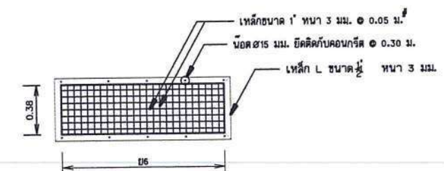
แปลนตะแกรงเหล็กกันล้น ขนาดจั่ว 1:20
