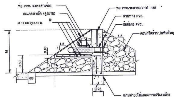
รูปตัด ช - ช (แสดงการเสริมเหล็ก) ขนาดจั่ว 1:25
