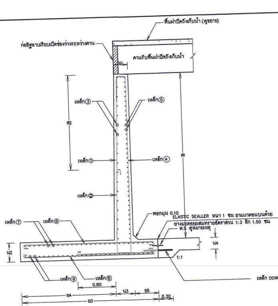
รูปตัดแนว ค - ค มาตราส่วน 1:25
