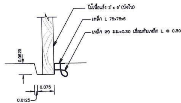
รูปขยาย 1 ขนาดจั่ว 1:5
