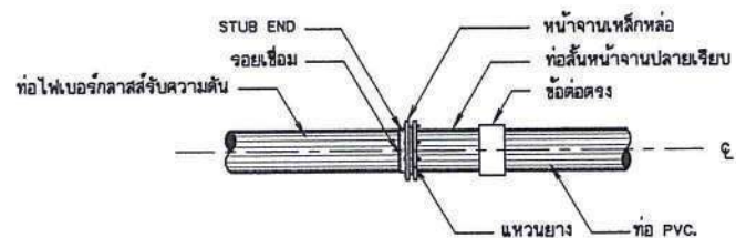
การบรรจบท่อไฟเบอร์กลาสส์ กับท่อ PVC.
