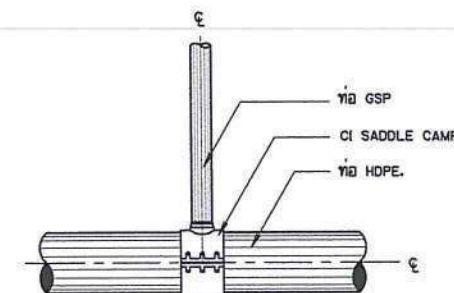
การบรรจบท่อสามทาง HDPE. กับท่อ GSP แบบ CI SADDLE CLAMP
