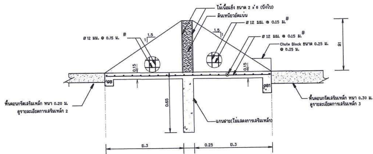
รูปตัด จ - จ ไม่แสดงขนาดจั่ว
