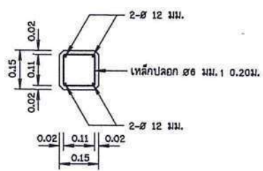
รูปตัด ข - ข ๙๑๙๙๑๐ 1:10
