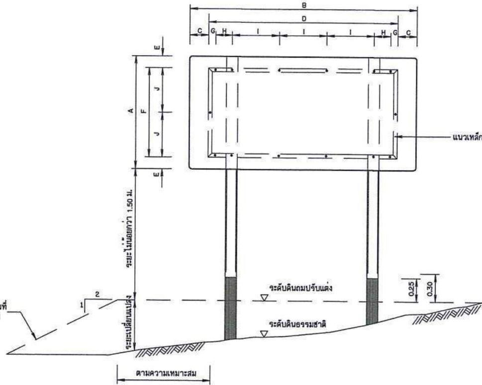
รูปแสดงการประกอบแผ่นป้าย ๙๑๙๙๑๐ 1:20
