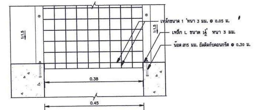
รูปตัด ช - ช ขนาดจั่ว 1:5
