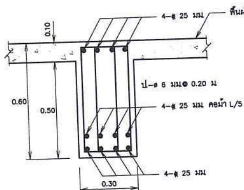
เสริมเหล็กคานแบบที่ ③ มาตราส่วน 1:10
