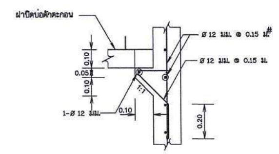
ขยาย 1 มาตราส่วน 1 : 10
