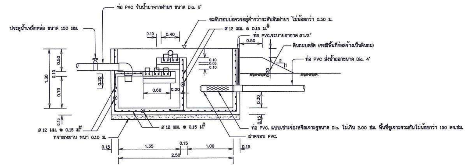
รูปตัด ข - ข มาตราส่วน 1 : 25
