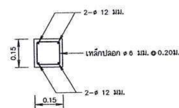
รูปตัด ก - ก มาตรฐาน 1:10
