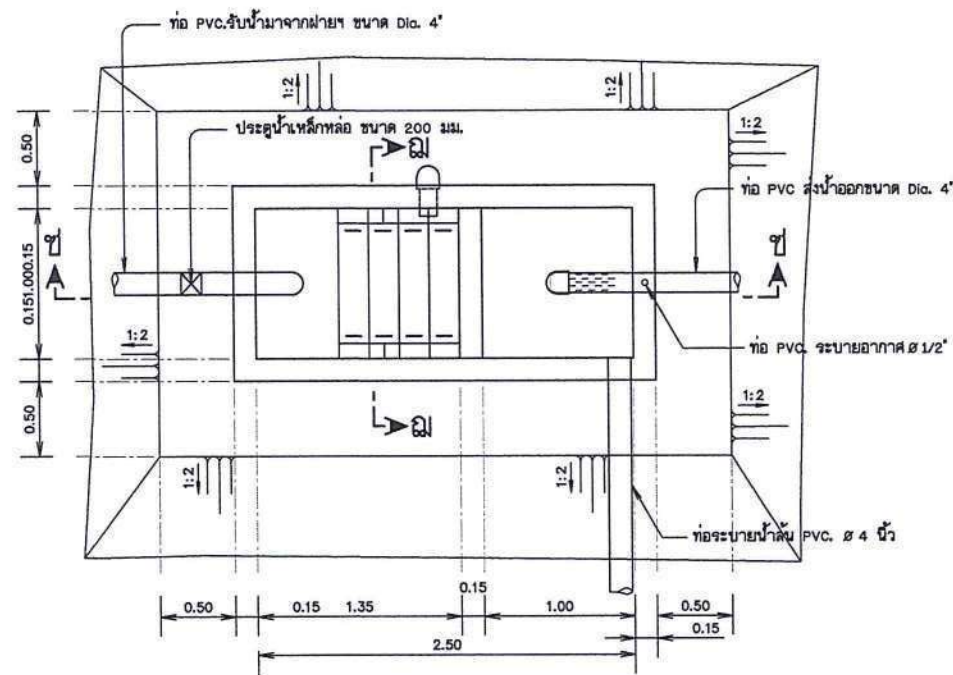
แปลนบ่อตกตะกอน มาตราส่วน 1 : 25
