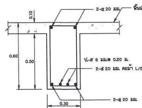
รูปตัดแสดงการเสริมเหล็กพื้นถึงเก็บน้ำ มาตราส่วน 1:20
