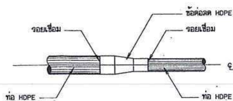
การบรรจุบ่อ HDPE กับข้อต่อลดท่อ HDPE
