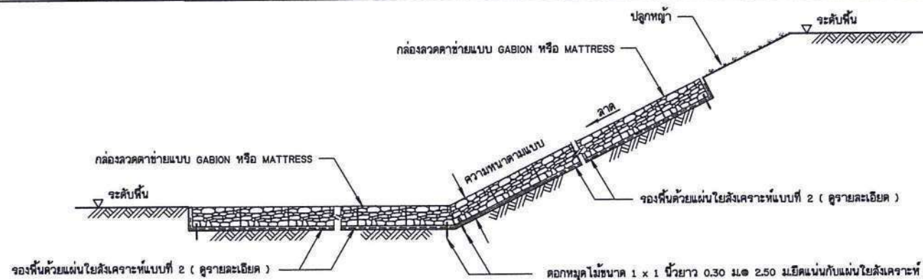
รูปตัดแสดงการวางกล่องลวดตาข่าย (แผ่นโพลีเอทิลีนรองพื้น)
