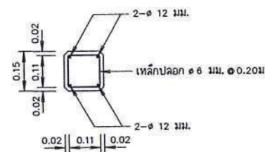
รูปตัด ข - ข มาตรฐาน 1:10
