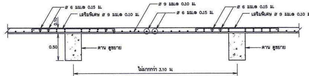
ขยายการเสริมเหล็กพื้นผิวดังเก็บน้ำ มาตราส่วน 1:20
