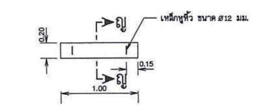
แปลนบ่อตกตะกอน มาตราส่วน 1 : 10
