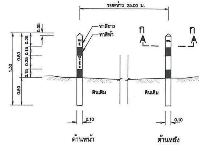
รูปขยายหลักแนวท่อ คลส.
