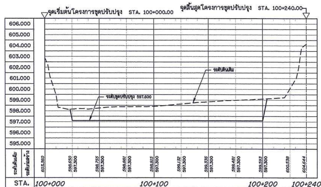
รูปตัดตามแนวขวางงานดินชุด มาตราส่วน 1:500 แนวตั้ง 1:500 แนวนอน 1:1,000
