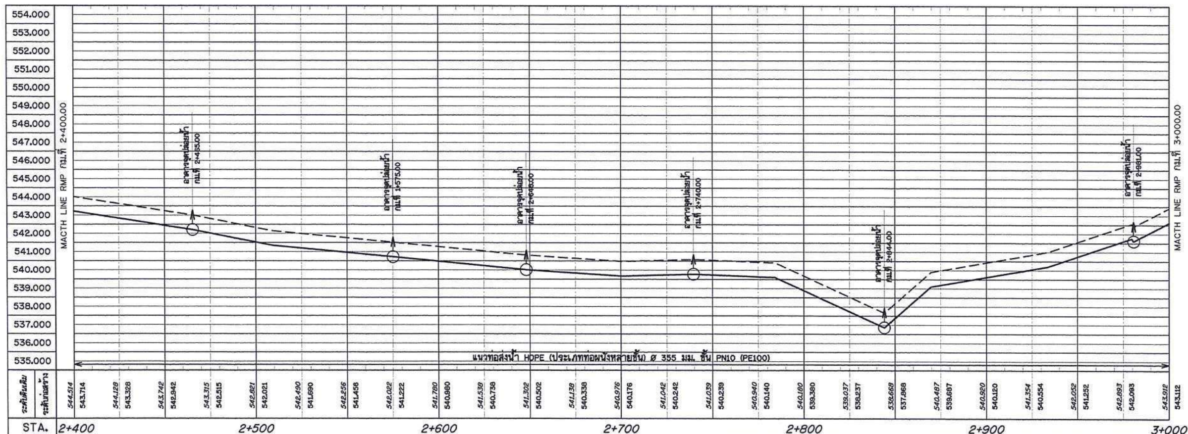
แปลนระบบส่งน้ำ สาย RMP. STA. 2+400 - 3+000 มาตรฐาน 1:1,000
