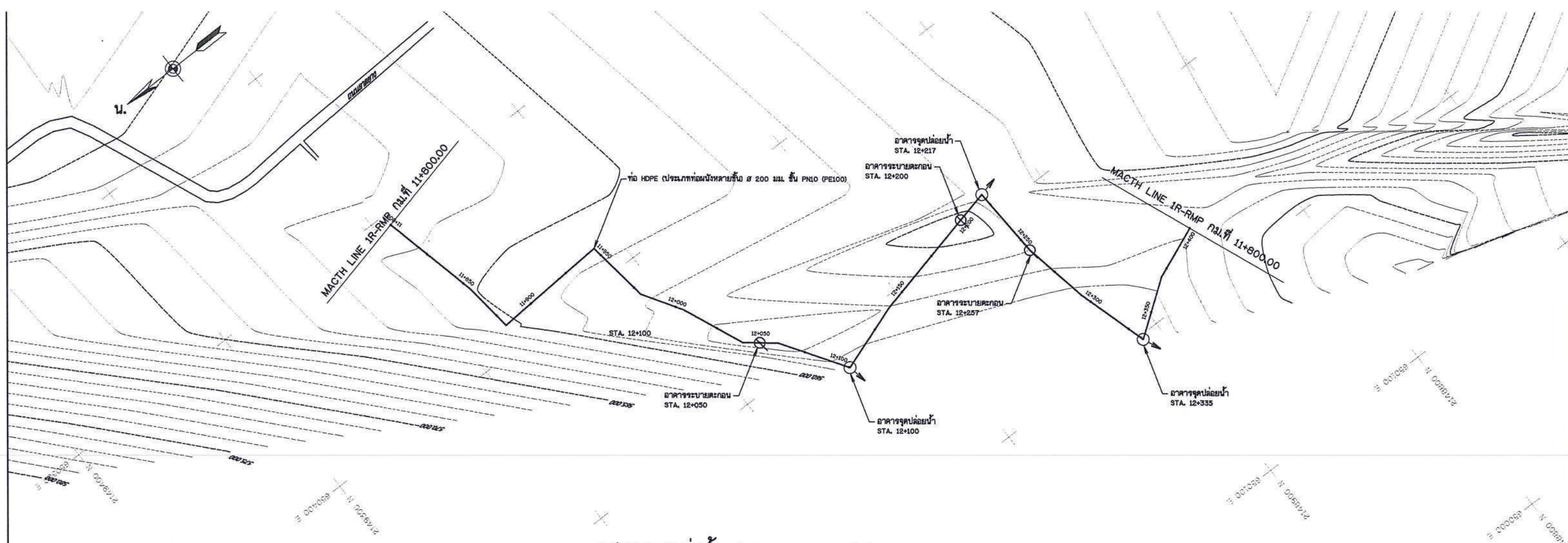
แผนระบบส่งน้ำ สาย 1R-RMP. STA. 11+800 - 12+400 มาตรฐาน 1:1,000
