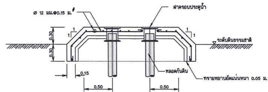
รูปขยายการเสริมเหล็กพื้นคอนกรีตเสริมเหล็ก มาตราส่วน 1:20
