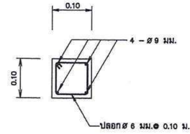
รูปตัด ก - ก
