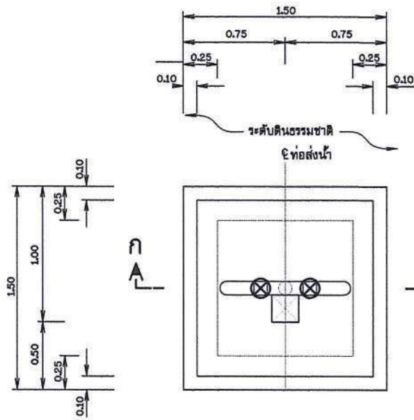
แปลนอาคารจุดปล่อยน้ำ 2 ด้าน
