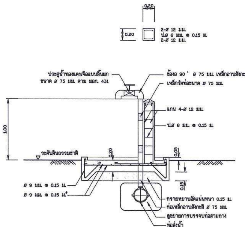
รูปตัด ข - ข
