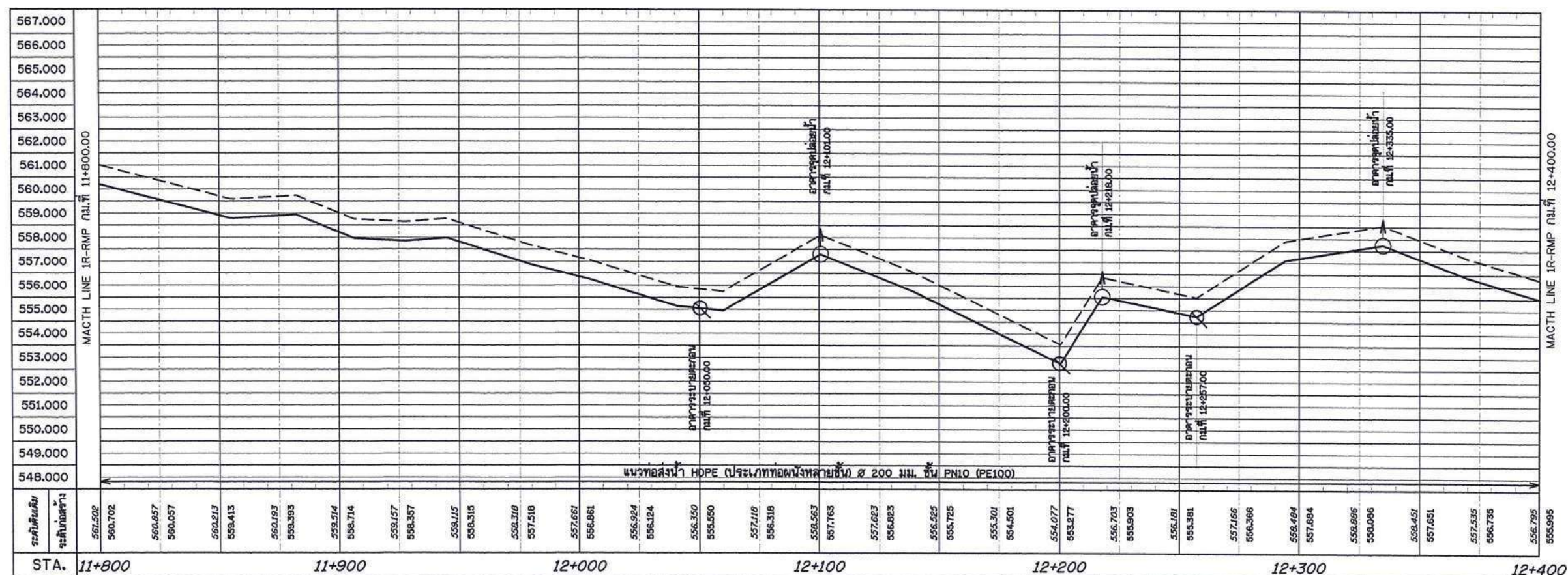
แผนระบบส่งน้ำ สาย 1R-RMP. STA. 11+800 - 12+400 มาตรฐาน 1:1,000
