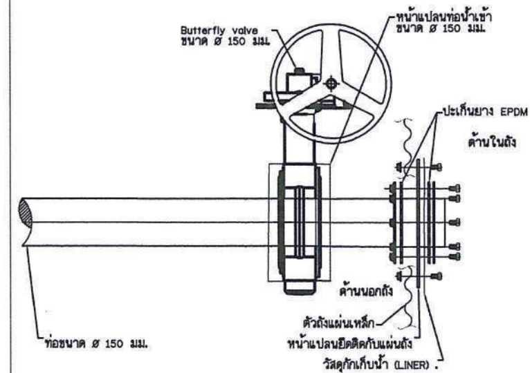
แบบขยาย 4 Scale NTC.
