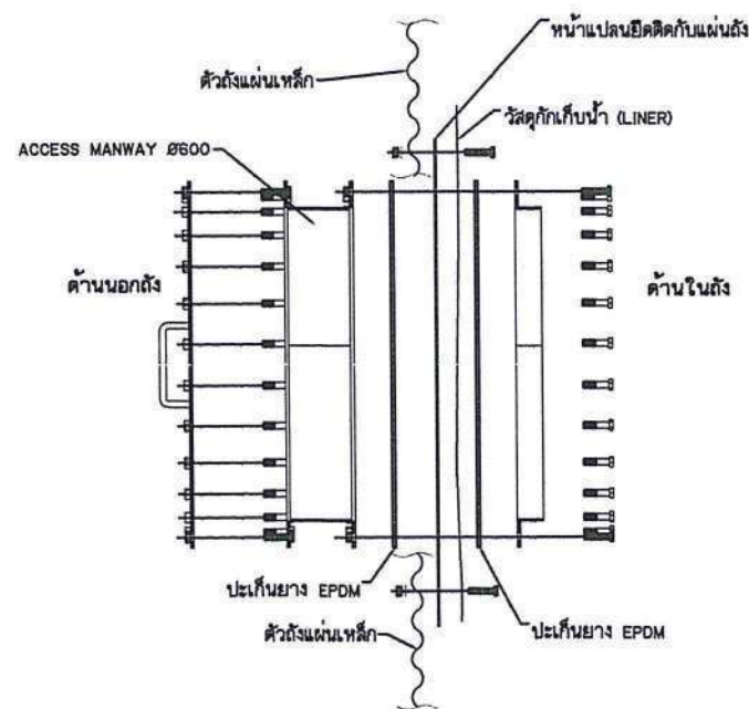
แบบขยายตรวจสอบบำรุงรักษา Scale NTC.
