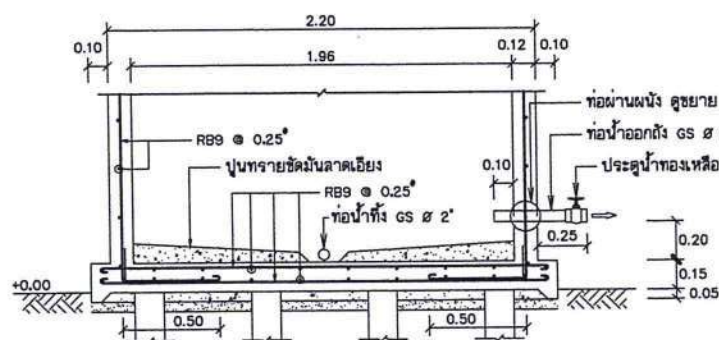
แสดงการเสริมเหล็กพื้นถัง มาตราส่วน 1:20
