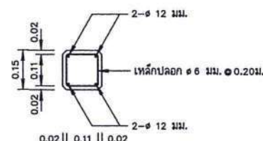
รายละเอียดการติดตั้งเสาป้าย มาตรฐาน 1:20
