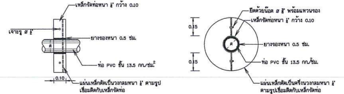
รูปขยาย "4"
