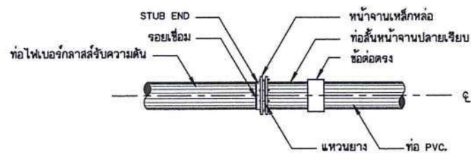
การบรรจบท่อไฟเบอร์กลาส์ กับท่อ PVC.
