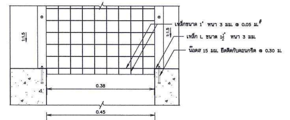
รูปตัด ข - ข
