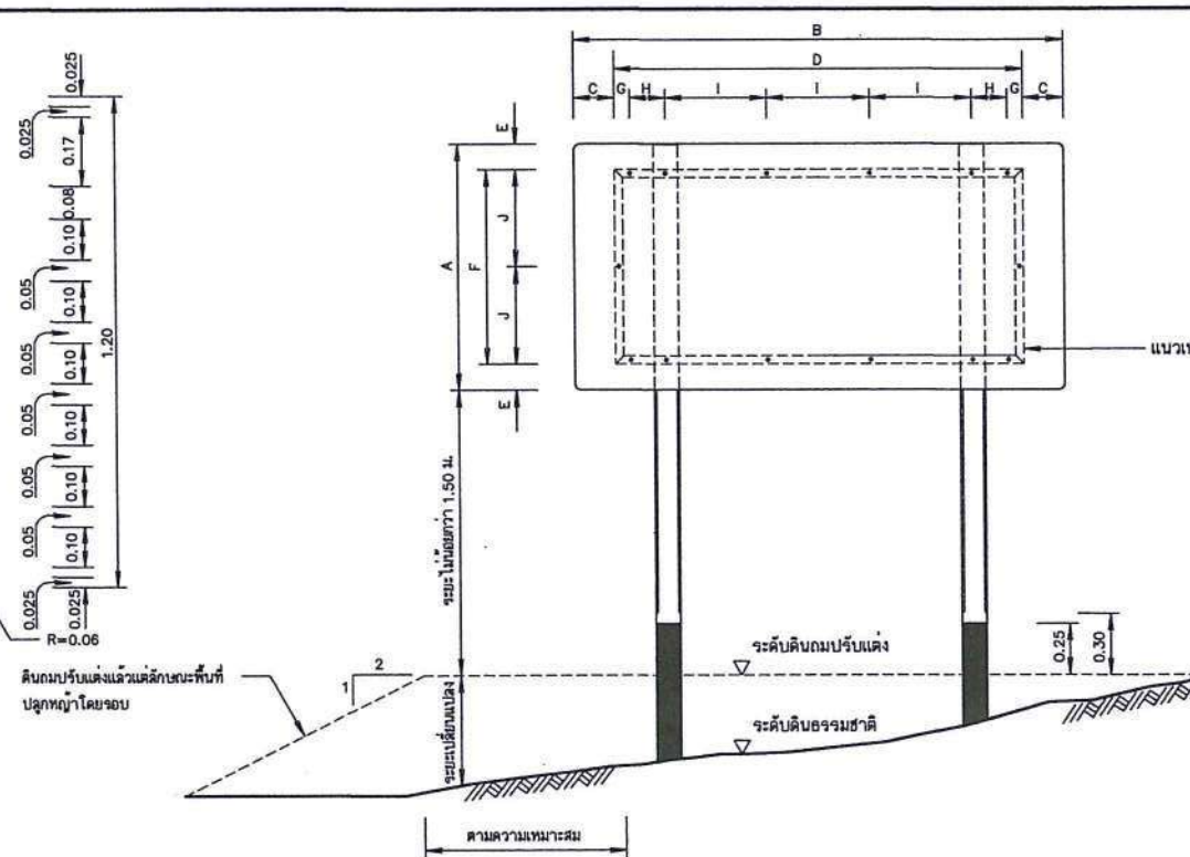
รูปแสดงการประกอบแผนผัง
