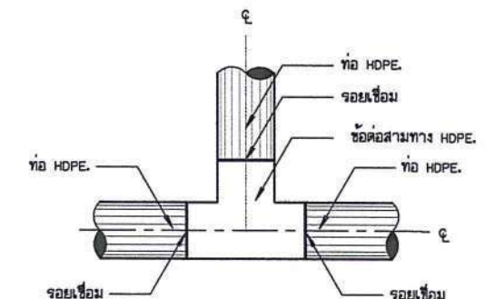
การบรรจบท่อสามทาง HDPE. กับท่อ HDPE.
