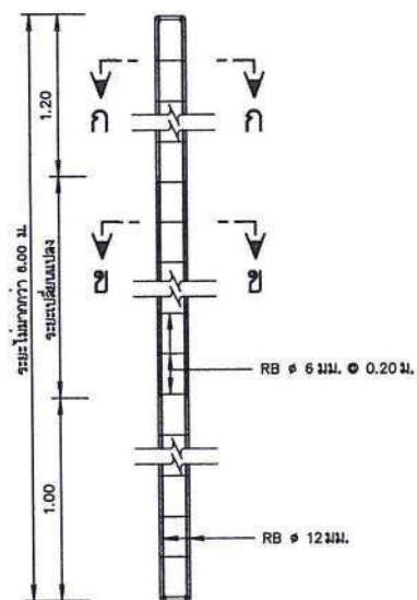
รายละเอียดภายใน คสส.
