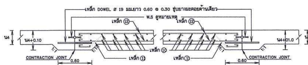
รูปตัดแสดงการเสริมเหล็กพื้นถึงเก็บน้ำ มาตราส่วน 1:20
