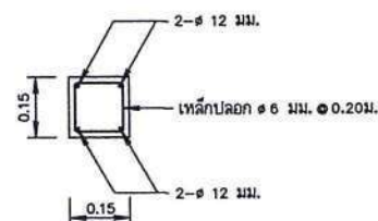
รายละเอียดภายใน คสส.
