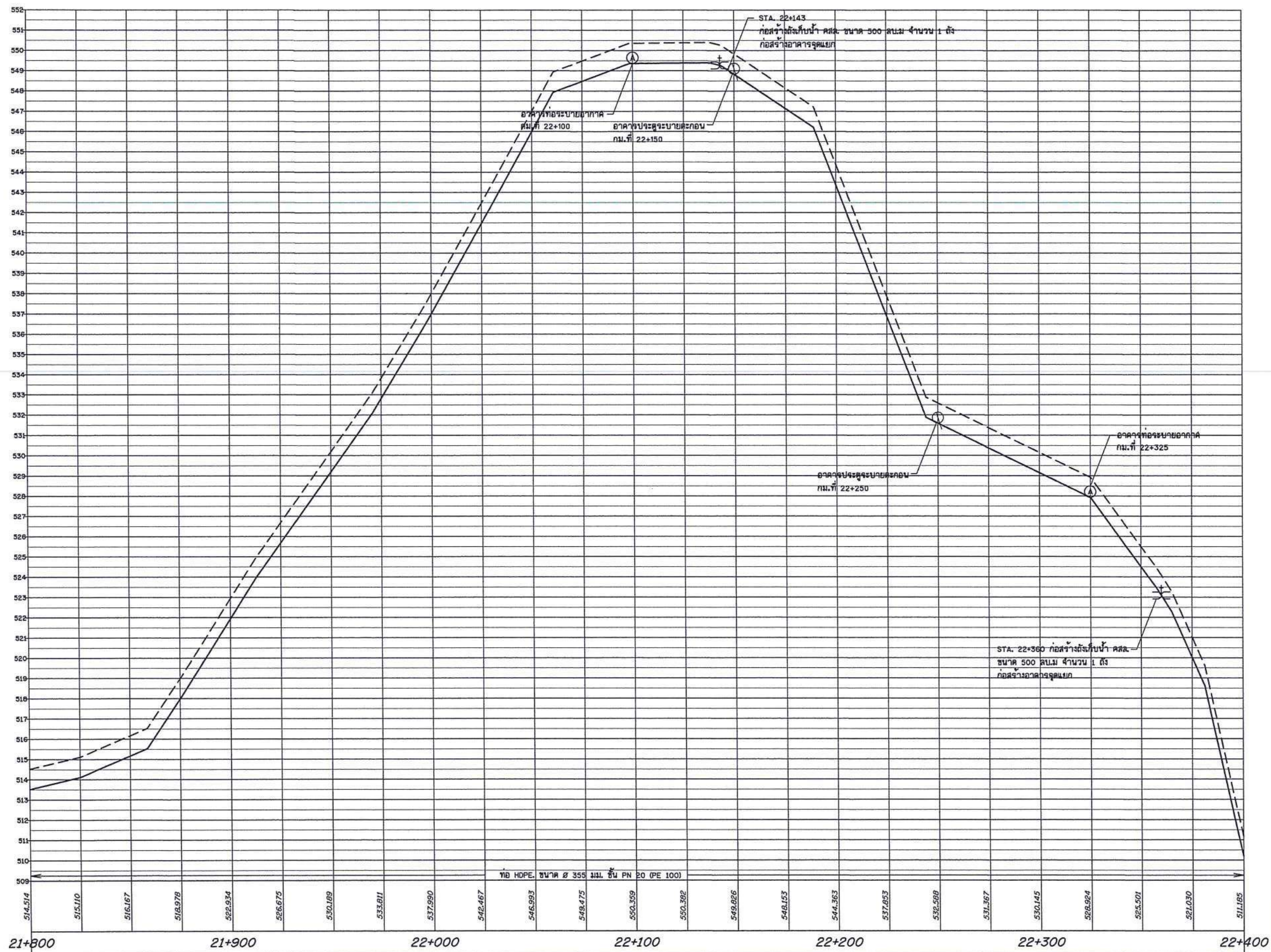
รูปตัดตามแนวยาว STA. 21+800 - 22+400
