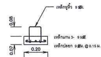
รูปตัด ข - ข
