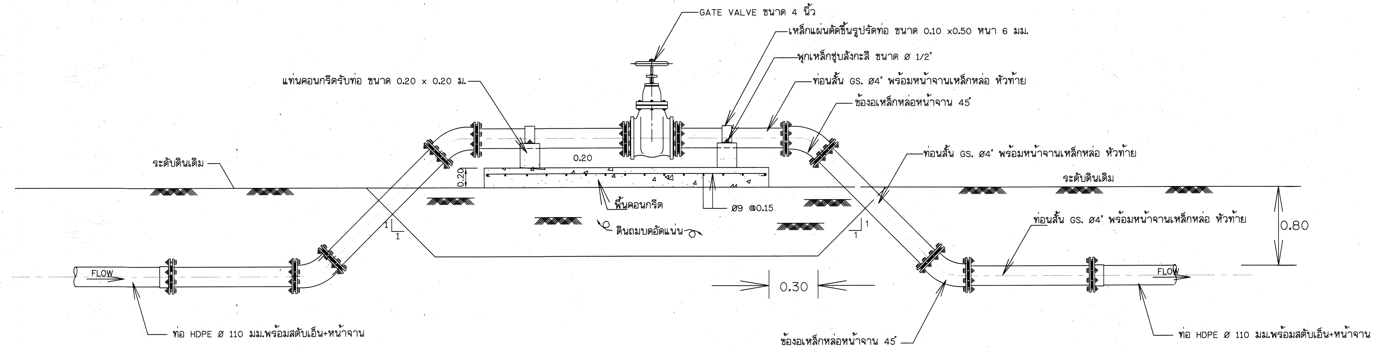
รูปตัดขยายประตุน้ำคูมท่อจ่ายน้ำ ท่อ HDPE ขนาด 110 มม. ก-ก
