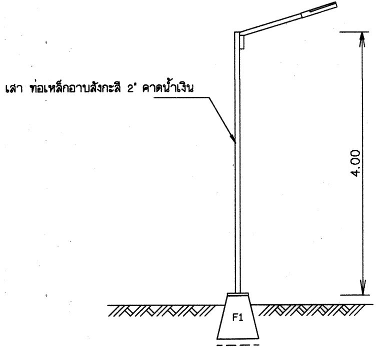
แบบเสาไฟ
