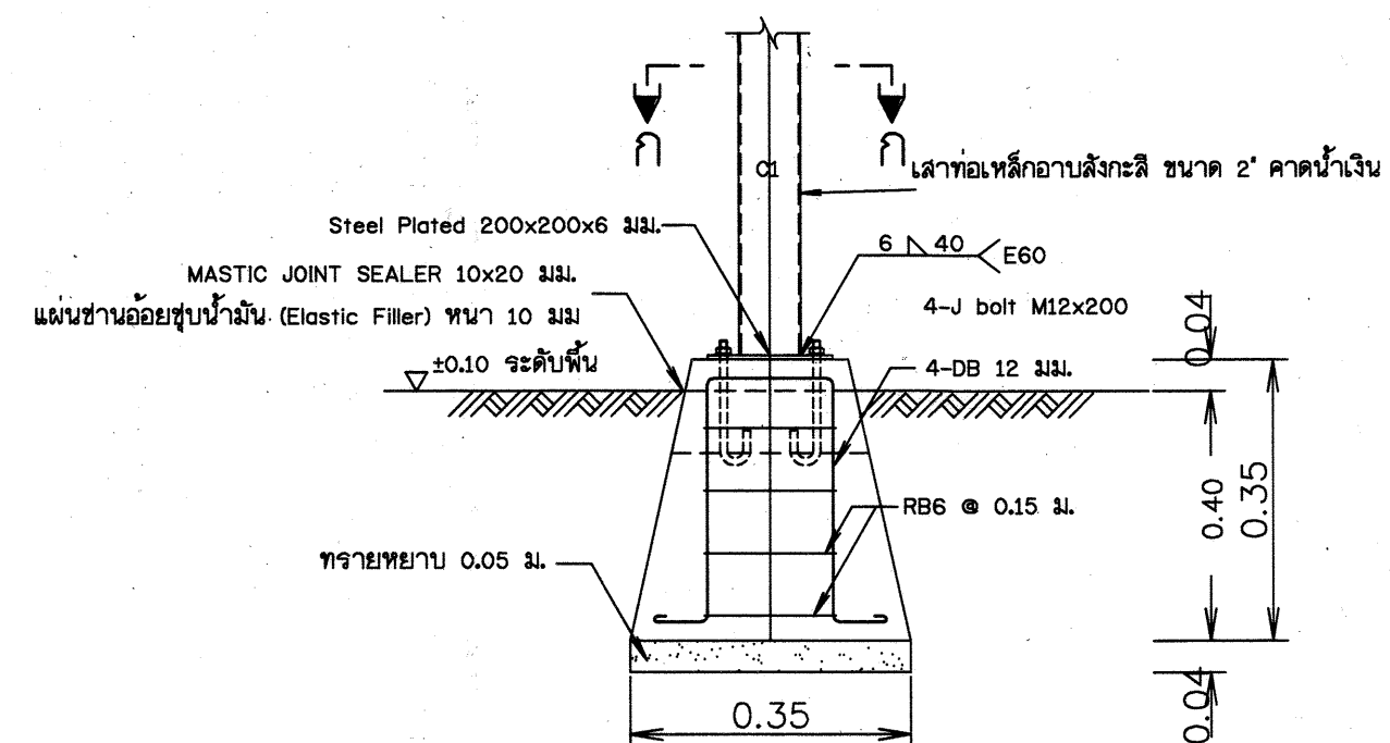
รูปขยายต่อม่อชุดไฟแสงสว่าง (ต่อม คสล. พร้อมสายรัดรูปพร้อมติดตั้ง) ไม่แสดงมาตราส่วน
