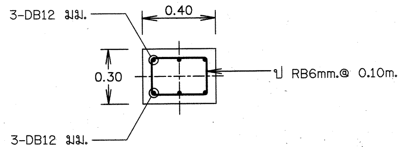
แบบขยายคาน B3
