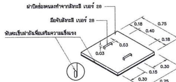
ขยายฝาดัดช่องคนลง
