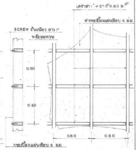
รูปขยายเค็ร่า, ฝา 1820
