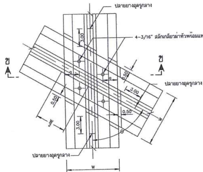
การต่อพาดทับกัน ไม่แสดงมาตราส่วน
