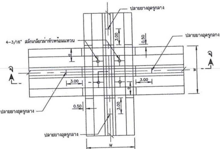
การต่อพาดทับกัน ไม่แสดงมาตราส่วน
