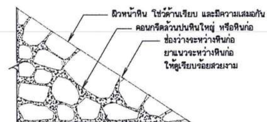
ขยายพืชน้ำคอนกรีตสวนปันทินใหญ่
