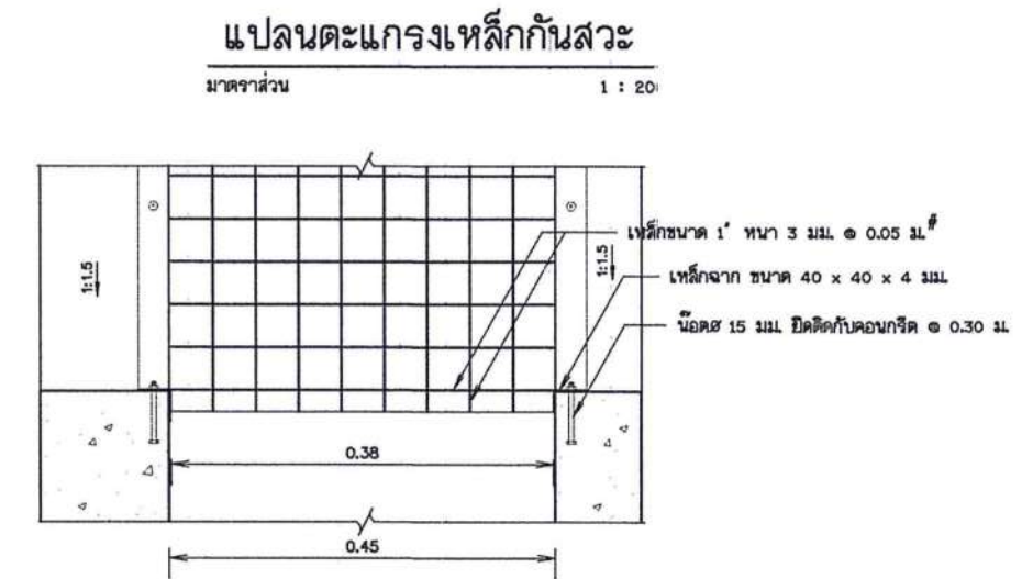
รูปตัด ช - ช
