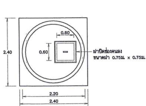
แปลน
