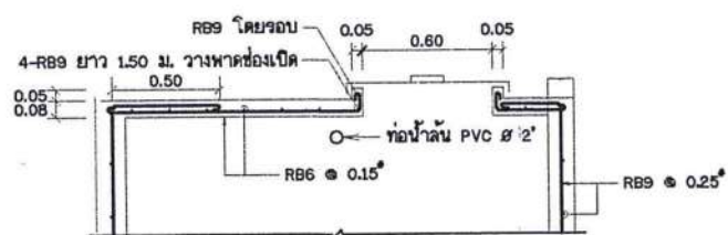
แสดงการเสริมเหล็กฝาดัด
