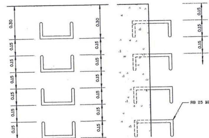
รูปขยายบันไดลิง มาตราส่วน 1:10
