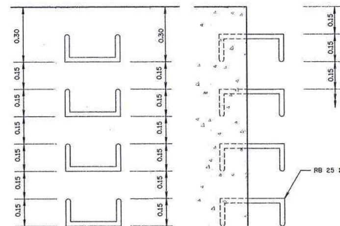
รูปขยายบันได มาตราส่วน 1:10
