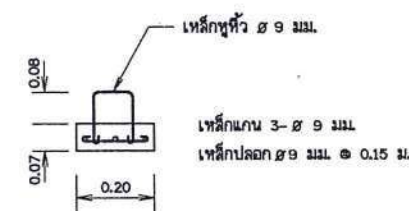
รูปตัด ญ - ญ
