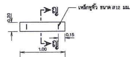
แปลนฝายบ่อดักตะกอน
