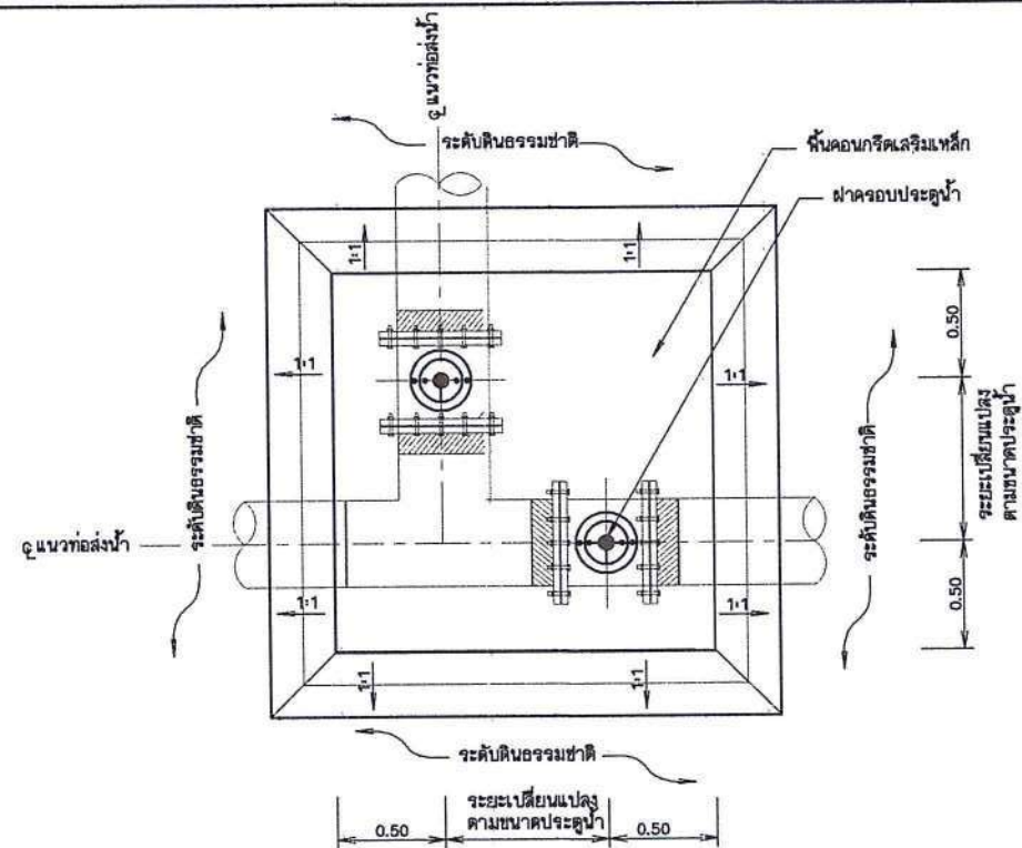
แปลงอาคารจุดแยก
