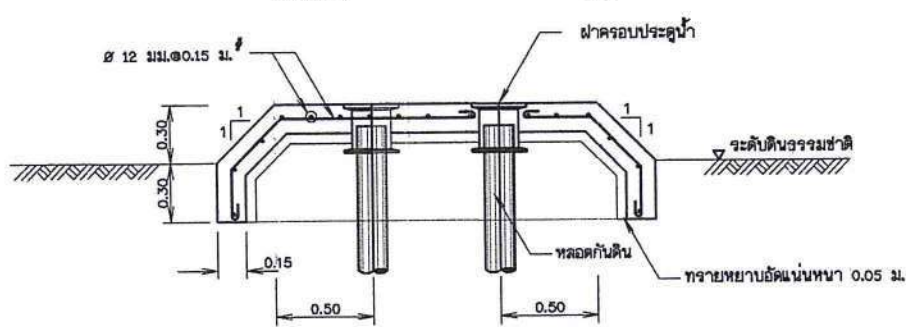
รูปขยายการเสริมเหล็กพื้นคอนกรีตเสริมเหล็ก
