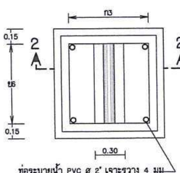
แปลนบ่อประจุรับน้ำ
