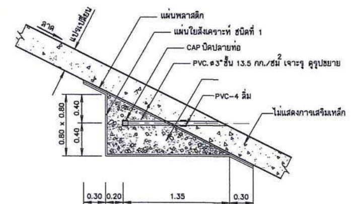
รูปขยายระบายน้ำกำแพงลาดเอียง
