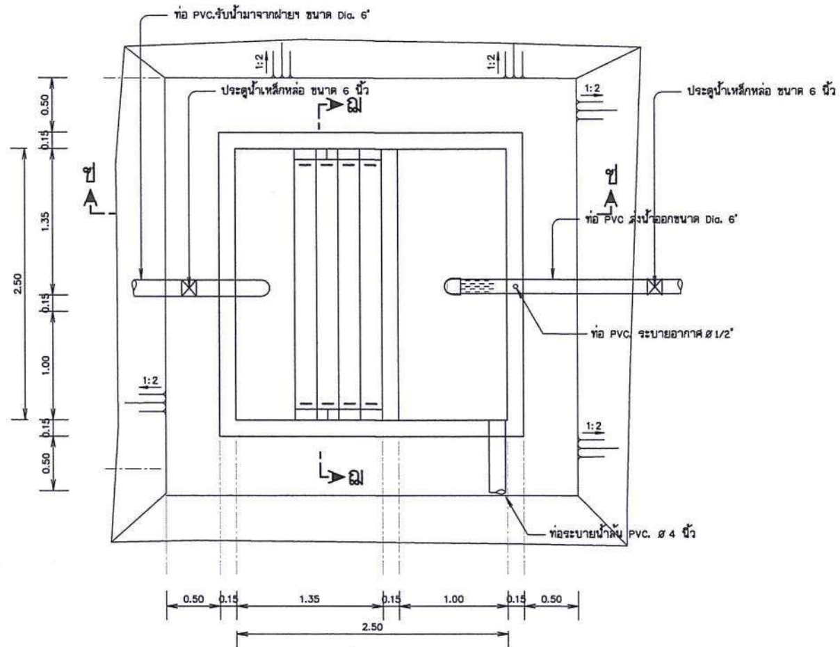
แปลนบ่อดักตะกอน
