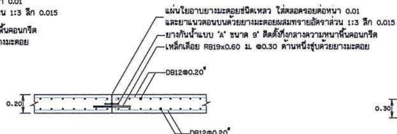
รูปขยายการเสริมเหล็ก 2
