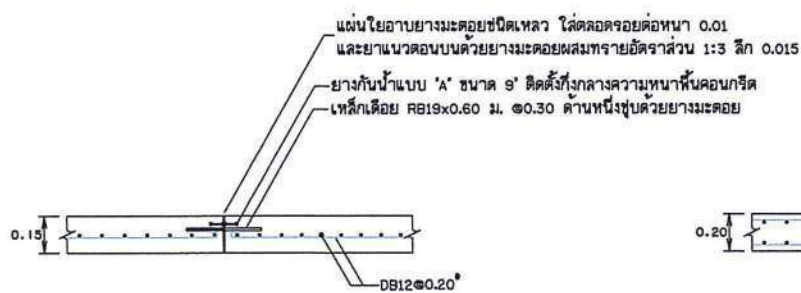
รูปขยายการเสริมเหล็ก 1
