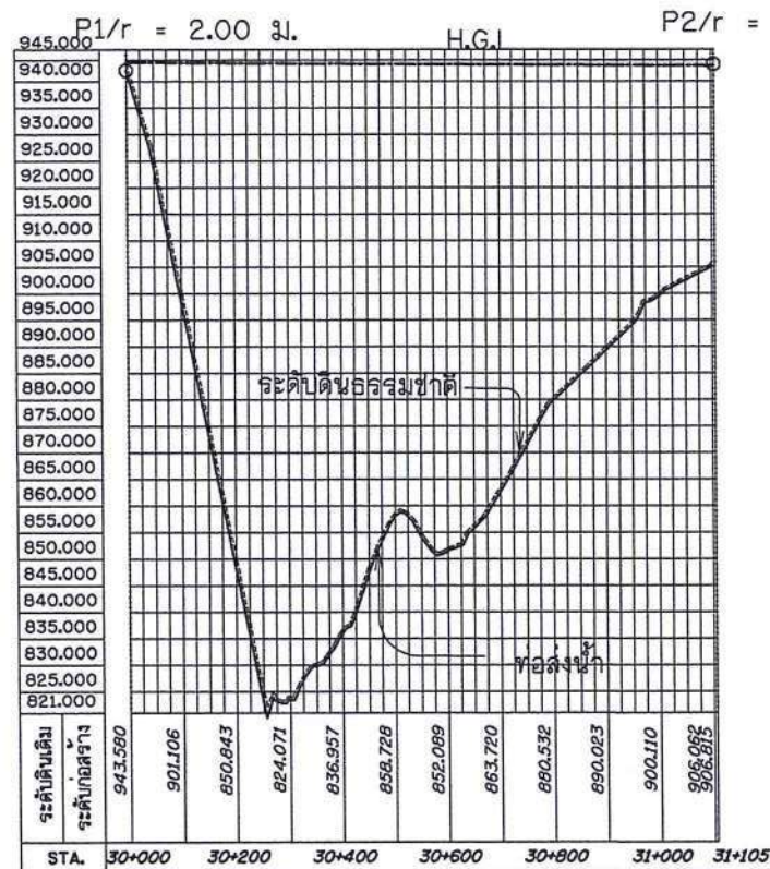
รูปตัดตามแนวยาวแสดง H.G.L. กม. 30+000
