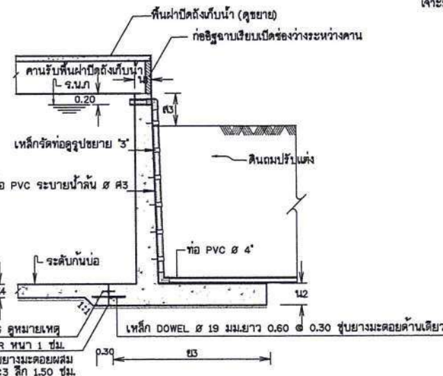
รูปตัดท่อรับน้ำหรือท่อระบายน้ำ
