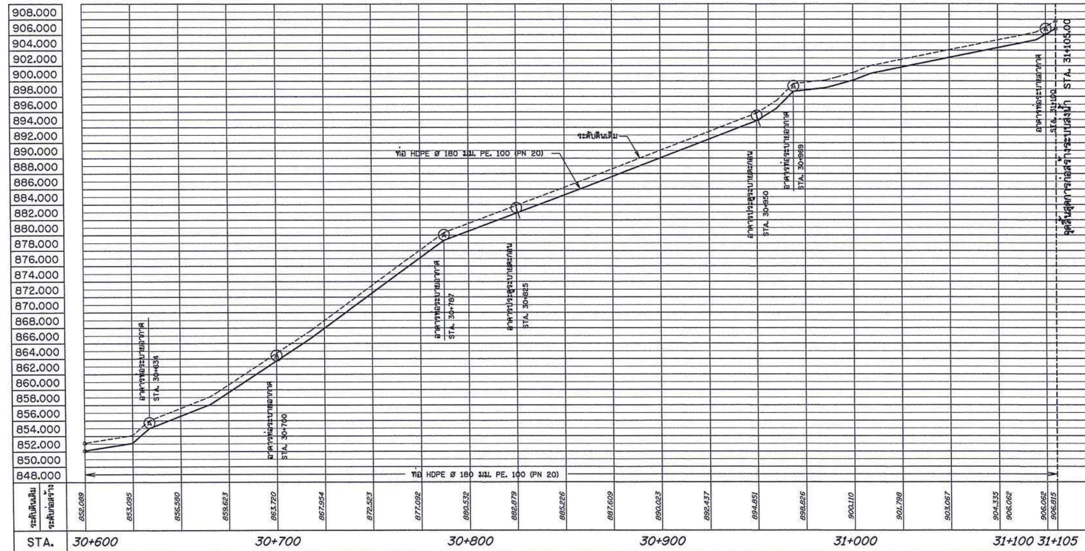
รูปตัดตามแนวยาว STA. 30+600 - 31+105
