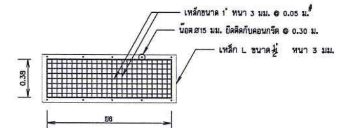
แปลนตะแกรงเหล็กกันลั่ว
