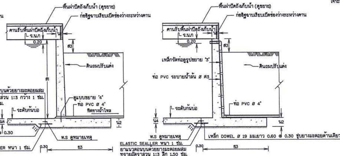
รูปตัดท่อระบายตะกอน
