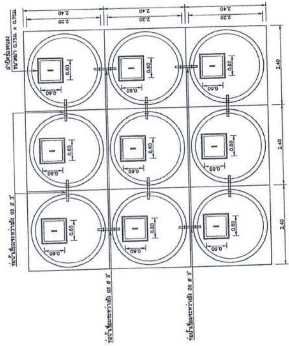
แปลนแบบ 9 ถึง มาตราส่วน 1:40
