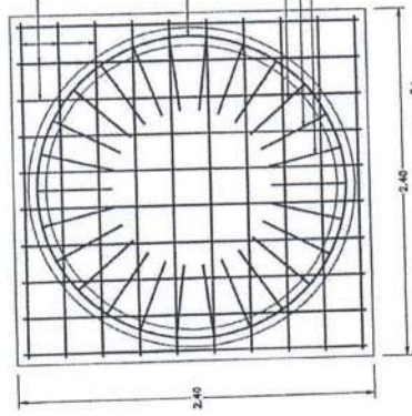
แสดงการเสริมเหล็กพื้นล่าง
