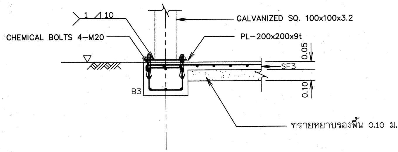
รูปตัด ก1 - ก1
