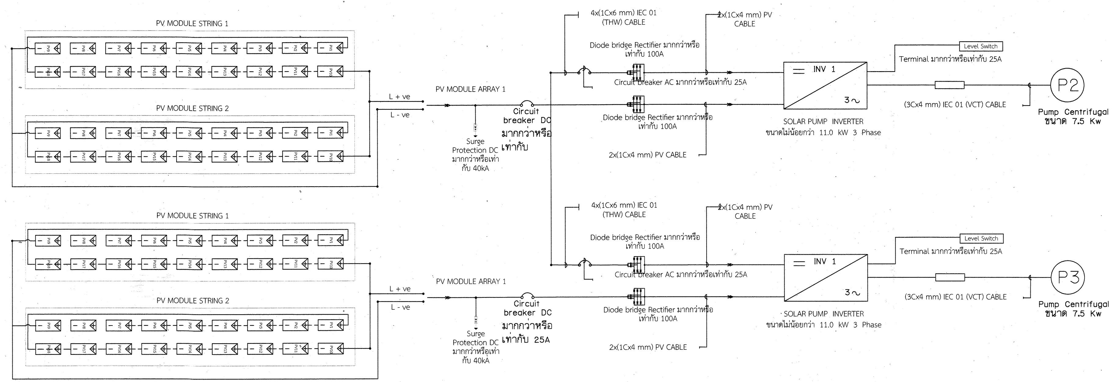
แผนผังระบบไฟฟ้า และไดอะแกรมไฟฟ้า ระบบกระจายน้ำด้วยพลังงานแสงอาทิตย์ N.T.S
