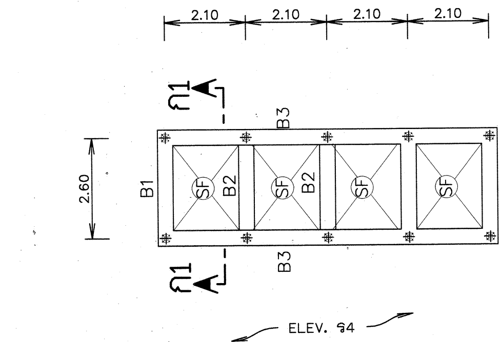
แปลนคานคอดินแผงเซลล์พลังงานแสงอาทิตย์
