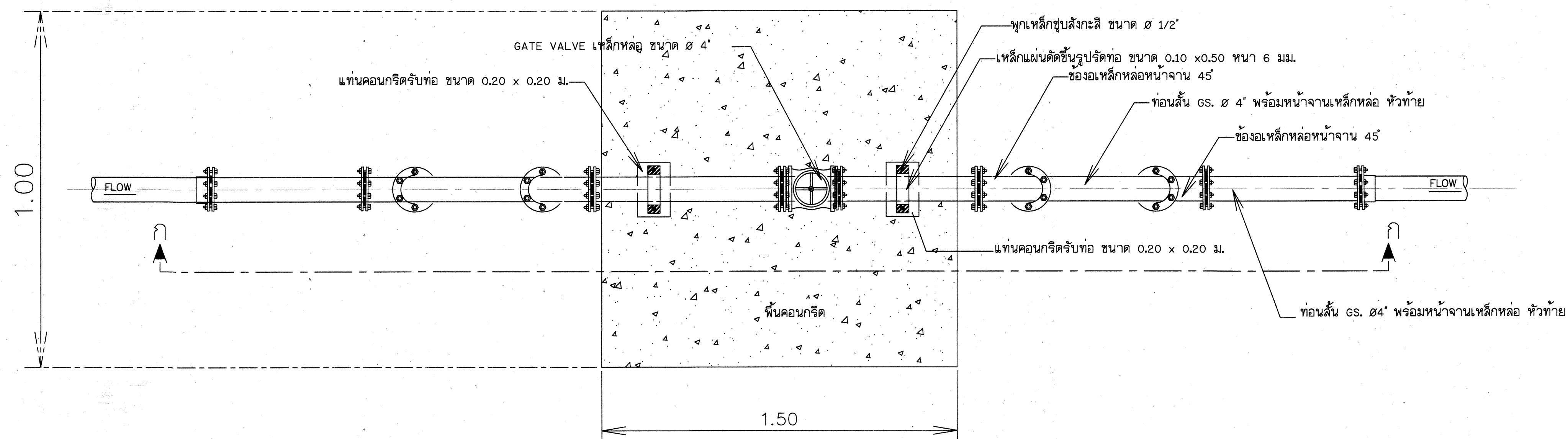
แปลนประตุน้ำคุมท่อจ่ายน้ำ HDPE ขนาด 110 มม.
