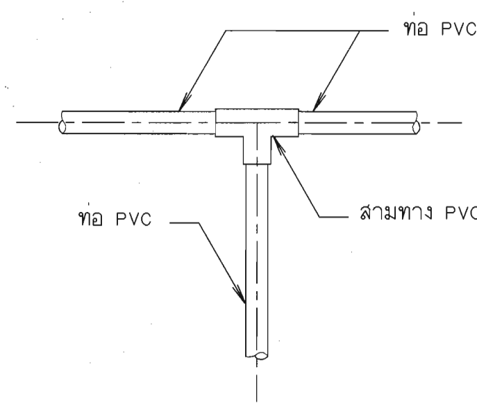
10. แบบการต่อสามทาง PVC
