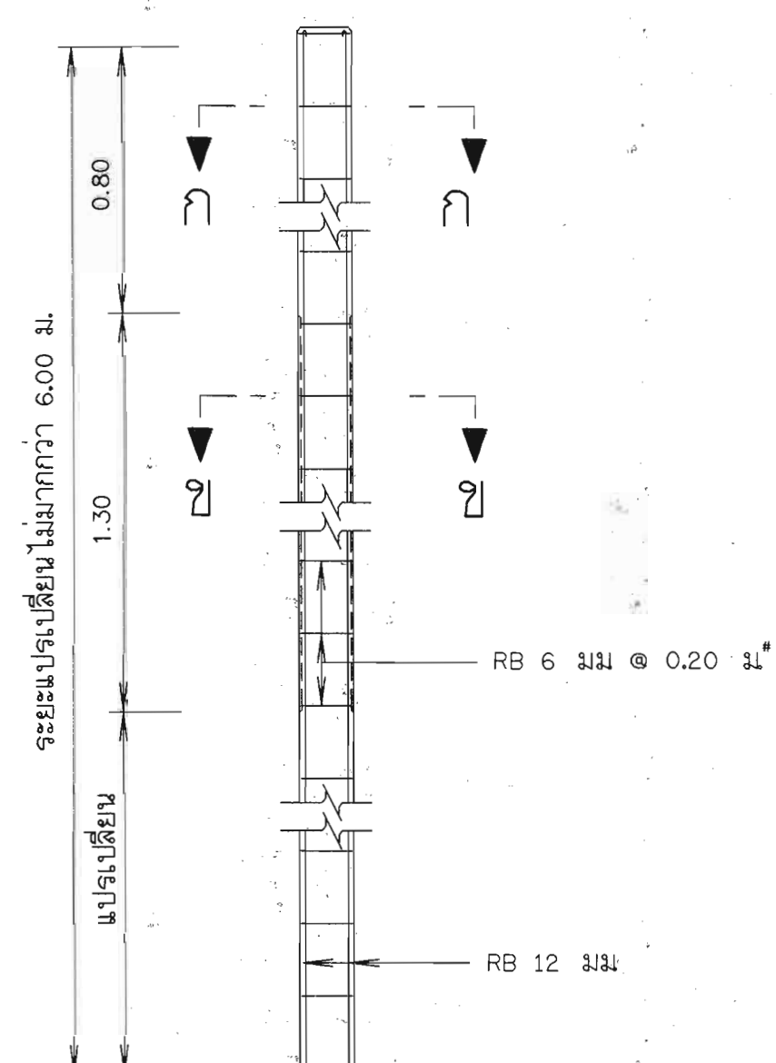
รายละเอียดสํำบาย คสส.
