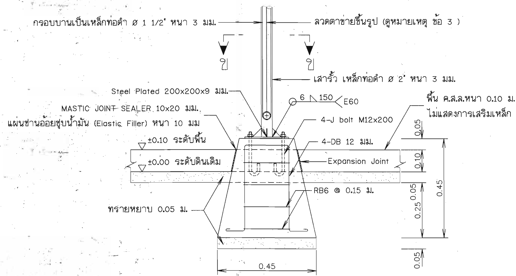
รูปขยายฐานรากโครงสร้างรับแผง F1 (คอมมู คสล. หลังสำเร็จรูปพร้อมติดตั้ง) ไม่แสดงมาตราส่วน
