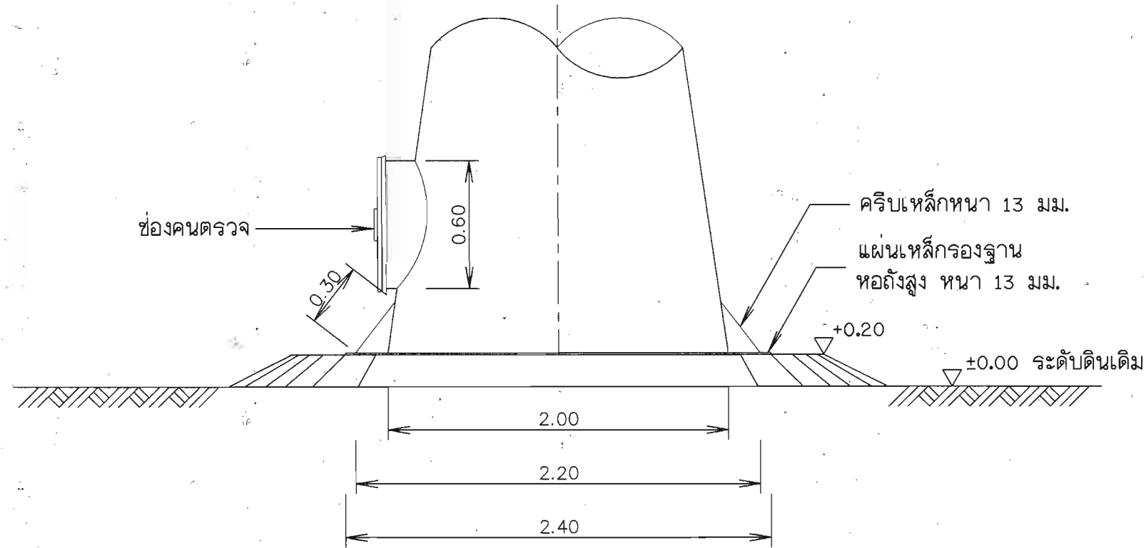
แบบขยายแมนโฮลล่างของถังสูง
