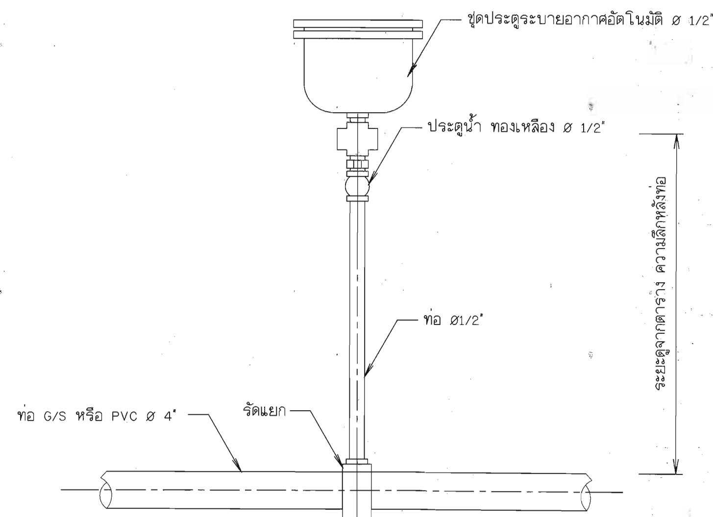
12. การติดตั้งประตูละบายอากาศอัตโนมัติ
