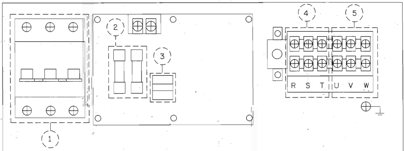
รายละเอียดตู้ควบคุมการปิด - เปิด
