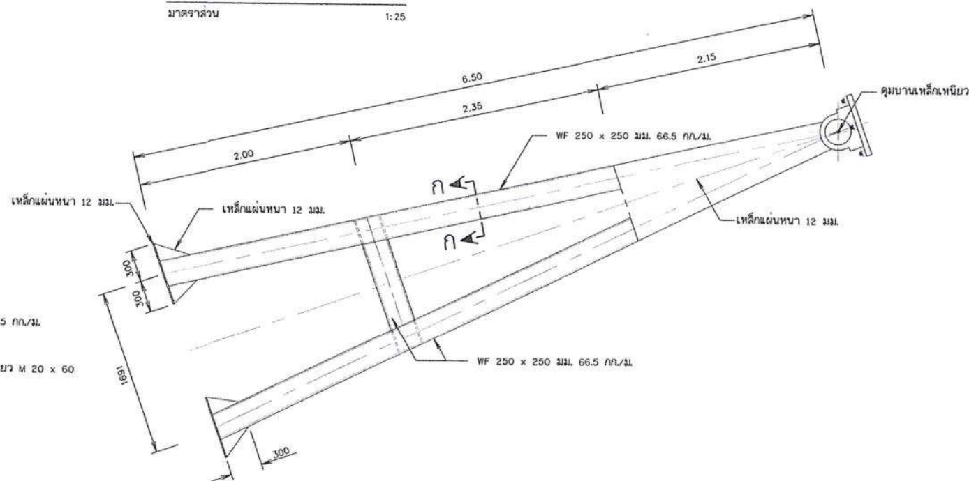
แปลนแขนบาน
