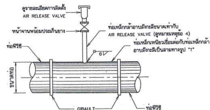
รายละเอียดข้อต่อแบบที่ 2 (กรณีท่อลงน้ำเป็นท่อสวิตซ์) ไม่แสดงมาตราส่วน
