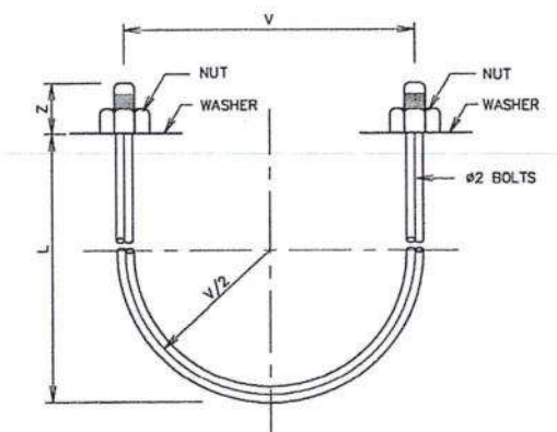
มาตรฐานการจ่อ U - BOLT ไม่แสดงมาตราส่วน
