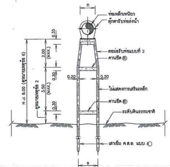
รูปตัด ข-ข ไม้แสดงนวลส่วน
