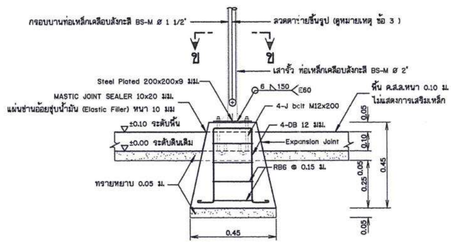
รูปขยายฐานรากโครงสร้างรับแผง F1 (ต่อม่อ คสล. หล่อสำเร็จรูปพร้อมติดตั้ง) ไม่แสดงมาตราส่วน
