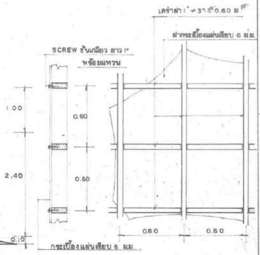
รูปขยายเคาะ, ฝา 1820
