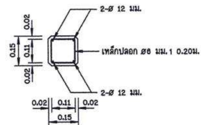
รูปตัด ข - ข มาตรฐาน 1:10
