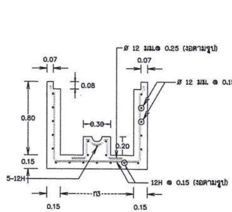
เหล็กเสริมบ่อประตูปรับน้ำ
