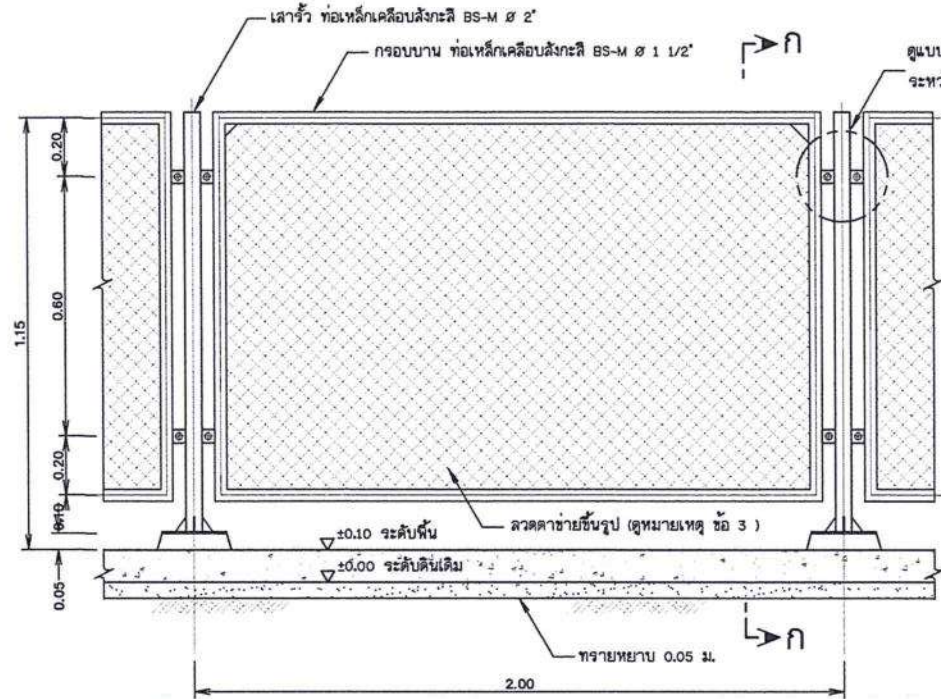
แบบขยายรั้วลวดตาข่าย ไม่แสดงขนาดจาล้วน
