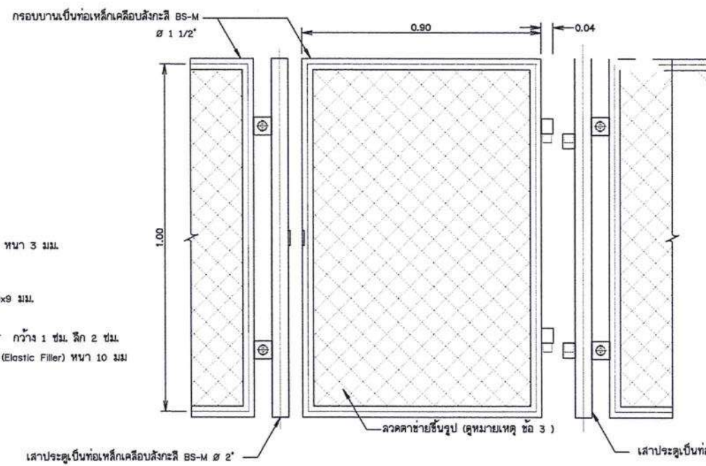
แบบขยายรายละเอียดประตู ไม่แสดงขนาดจาล้วน
