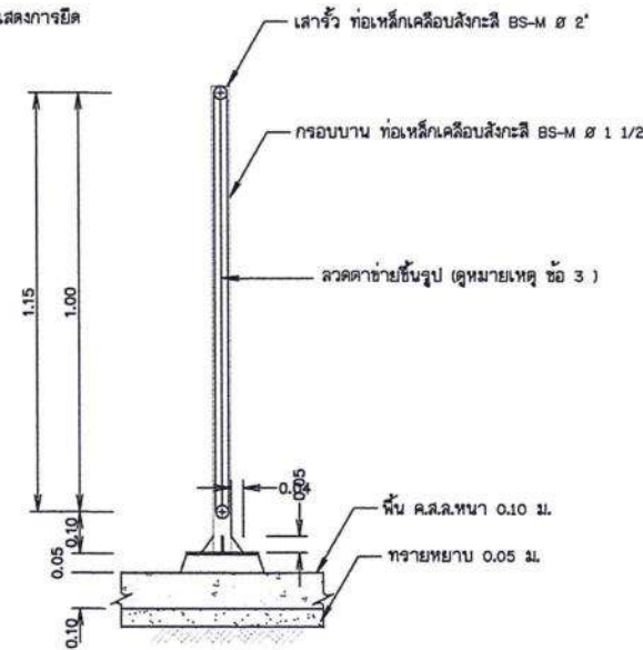
รูปตัด ก-ก ไม่แสดงขนาดจาล้วน
