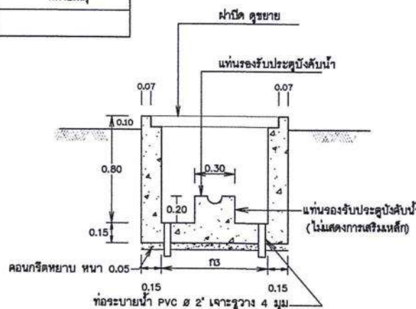
รูปตัด 2 - 2
