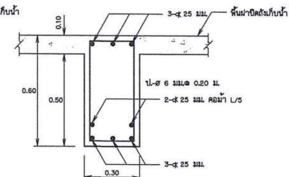
เสริมเหล็กคานแบบที่ ② มาตราส่วน 1:10
