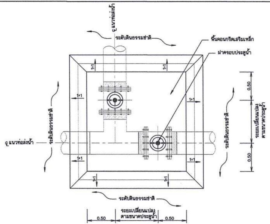
แปลนอาคารจุดแยก
