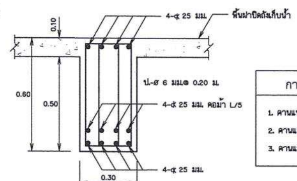
เสริมเหล็กคานแบบที่ ③ มาตราส่วน 1:10
