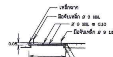
รูปตัดแนว 4 - 4
