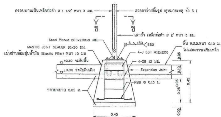
รูปขยายฐานจากโครงสร้างรับแผง F1 (คอม่อ คส.ล. ห่อผ้าใบรูปหรือมอดูล) ไม่แสดงขนาดจั่วส่วน
