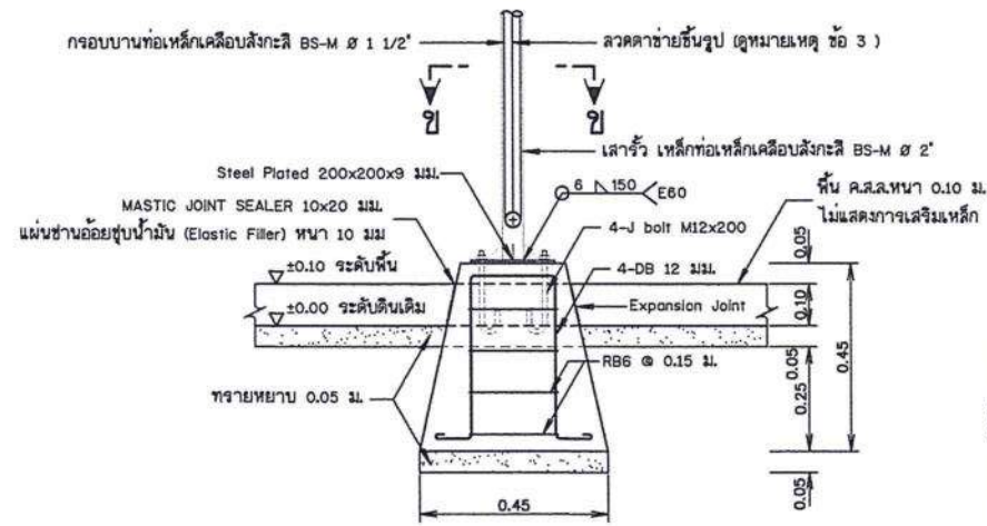
รูปขยายฐานรากโครงสร้างรับแผง F1 (เดอม่อ คสล. หล่อสำเร็จรูปพร้อมติดตั้ง) ไม่แสดงขนาดจาล้วน
