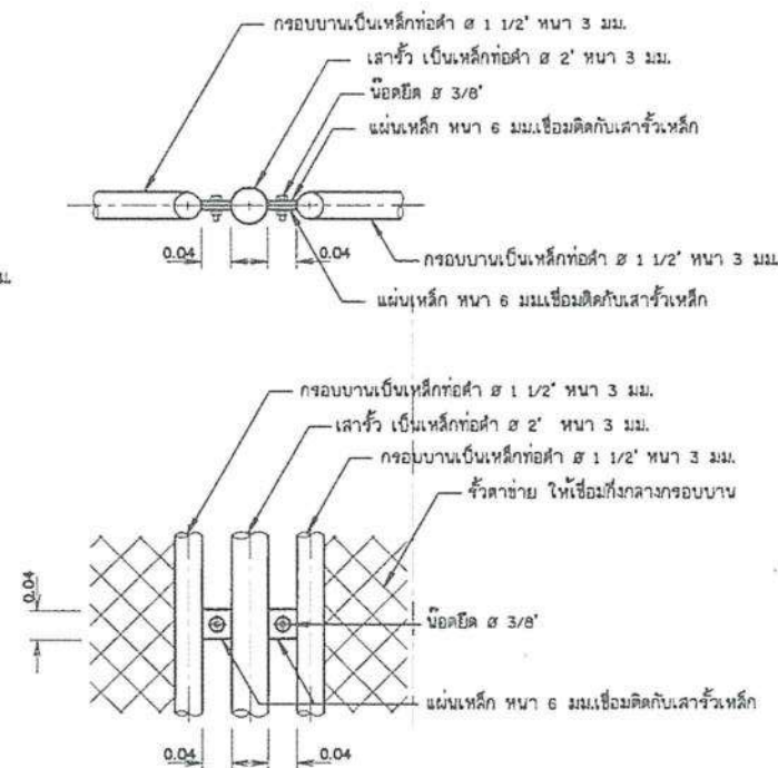
แบบขยายรายละเอียดแสดงการยึดระหว่างรั้วกับเสา ไม่แสดงขนาดจั่วส่วน
