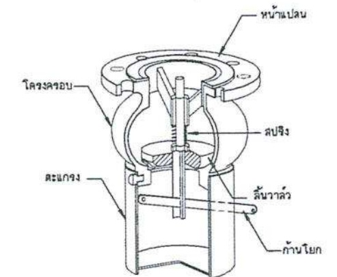
15. การต่อท่อเครื่องสูบน้ำ ไม่แสดงขนาดราส่วน
