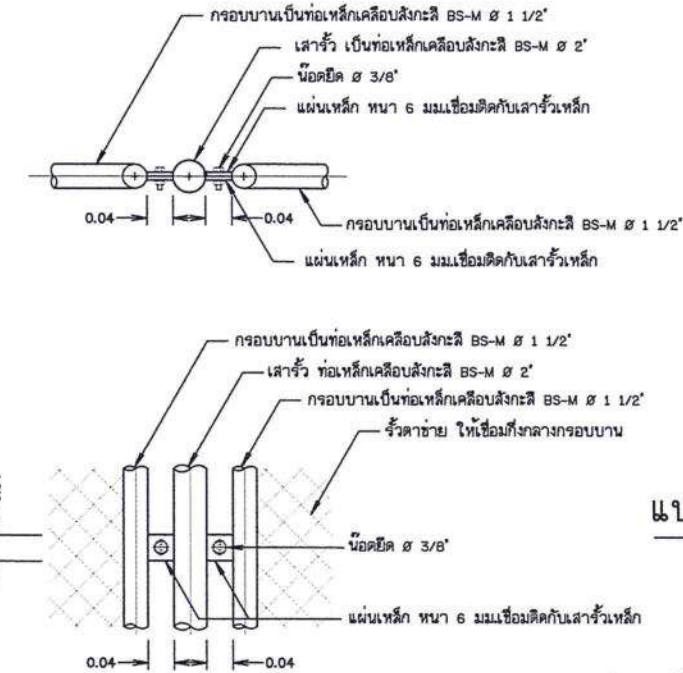
แบบขยายรายละเอียดแสดงการยึดระหว่างรั้วกับเสา ไม่แสดงขนาดจาล้วน
