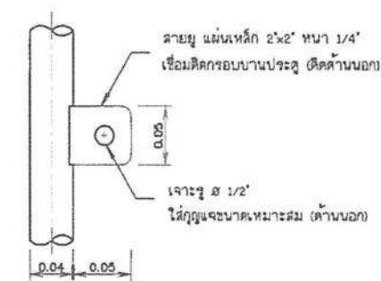
แบบขยายสายยู ไม่แสดงขนาดจั่วส่วน
