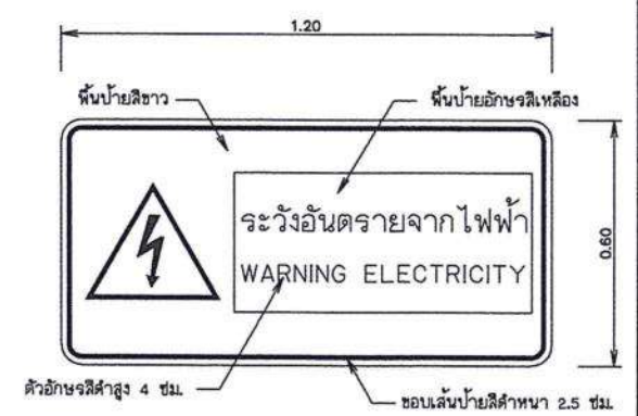
ป้ายเตือนกระแสไฟฟ้า ไม่แสดงขนาดจาล้วน
