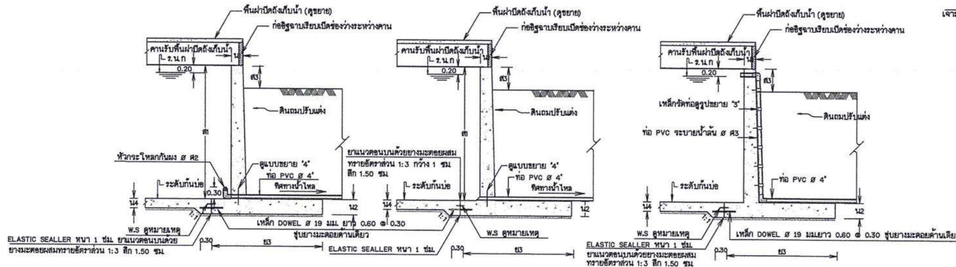
รูปตัดท่อน้ำ
