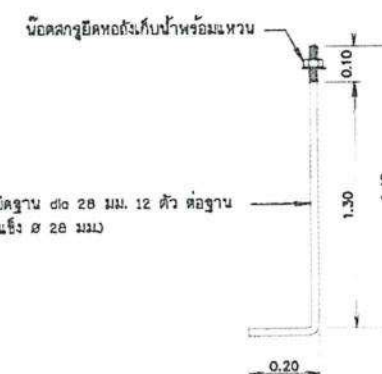
แบบขยายหลักเกลิวยึดฐาน
