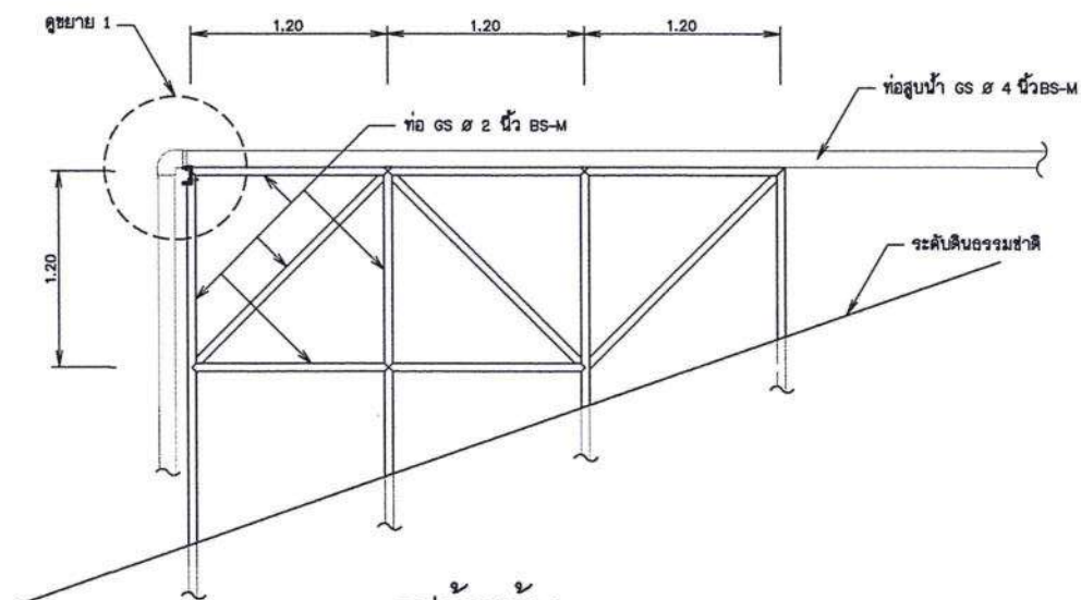
รูปด้านข้าง
