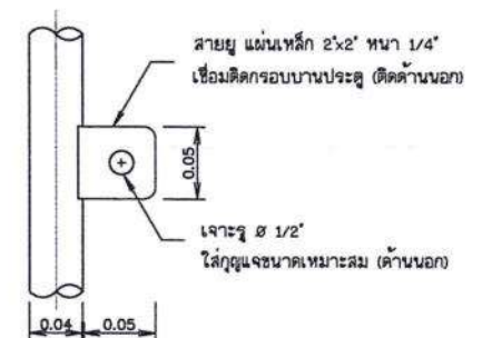
แบบขยายสายยู ไม่แสดงขนาดจาล้วน
