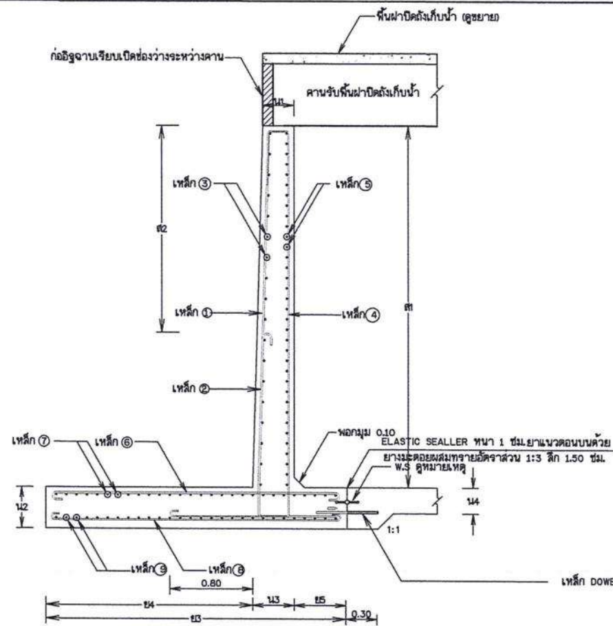
รูปตัดแนว ค - ค มาตราส่วน 1:25
