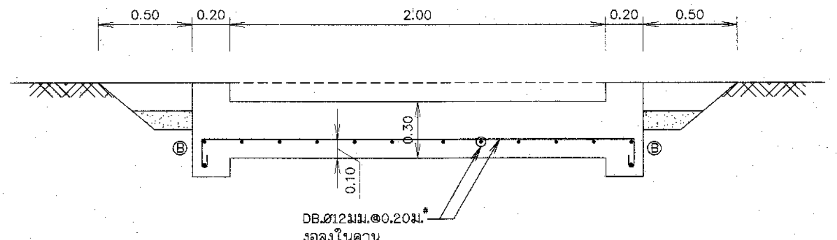
รูปตัด ข - ข
