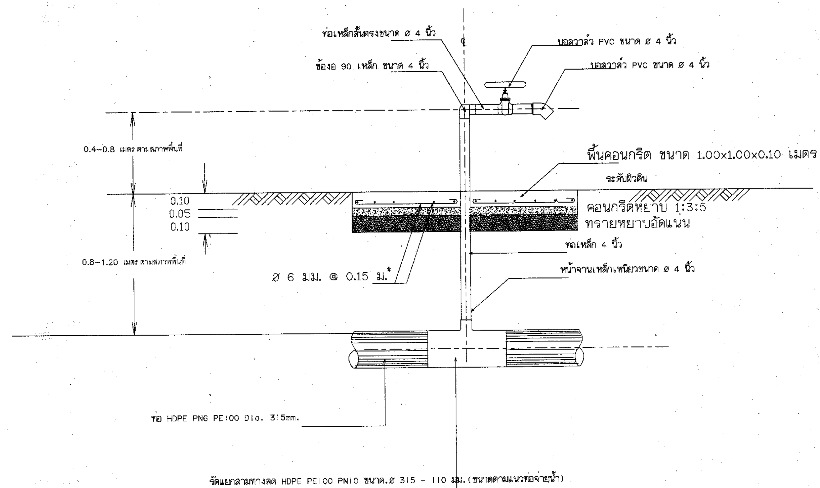
รูปตัด, แสดงการติดตั้งจุดกระจายน้ำสำหรับท่อเหล็ก HDPE Dia.315
