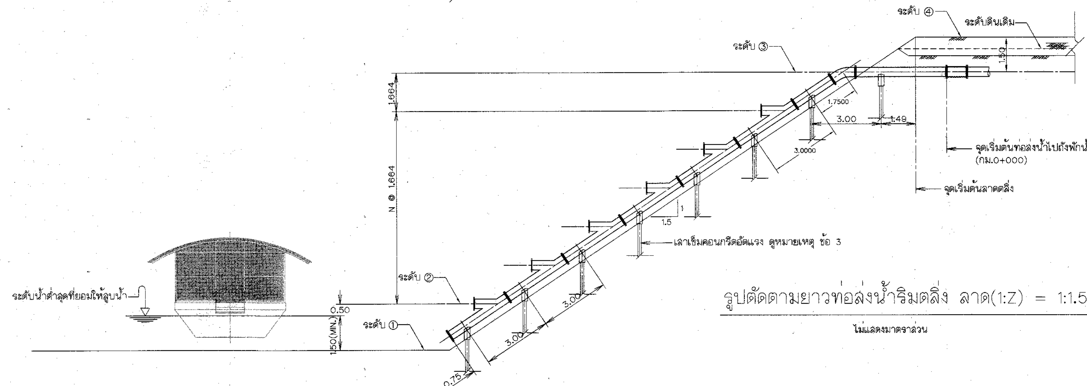
รูปตัดแสดงการเปลี่ยนท่อน้ำ 10" -> 16"
