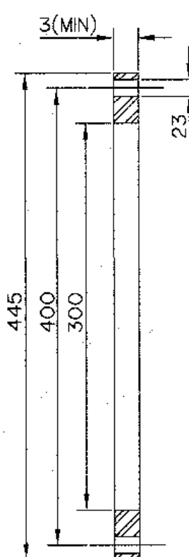
ปะเก็นยาง
