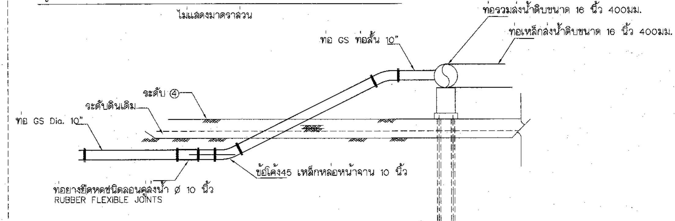
รูปตัดแสดงการเปลี่ยนท่อน้ำ 10" -> 16"
