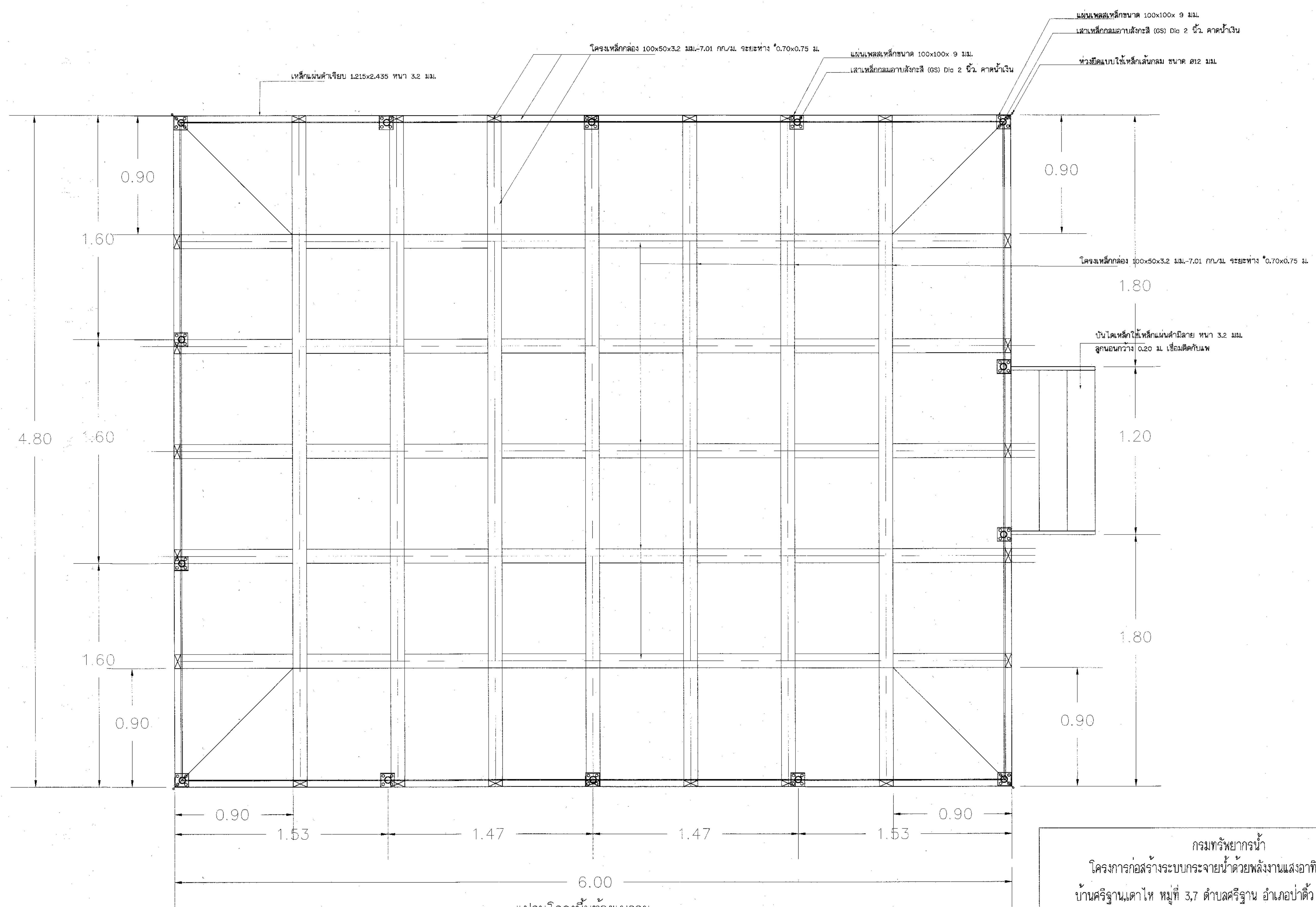
แปลน โครงพื้นที่ถังแพลลอย มาตราส่วน 1:100
