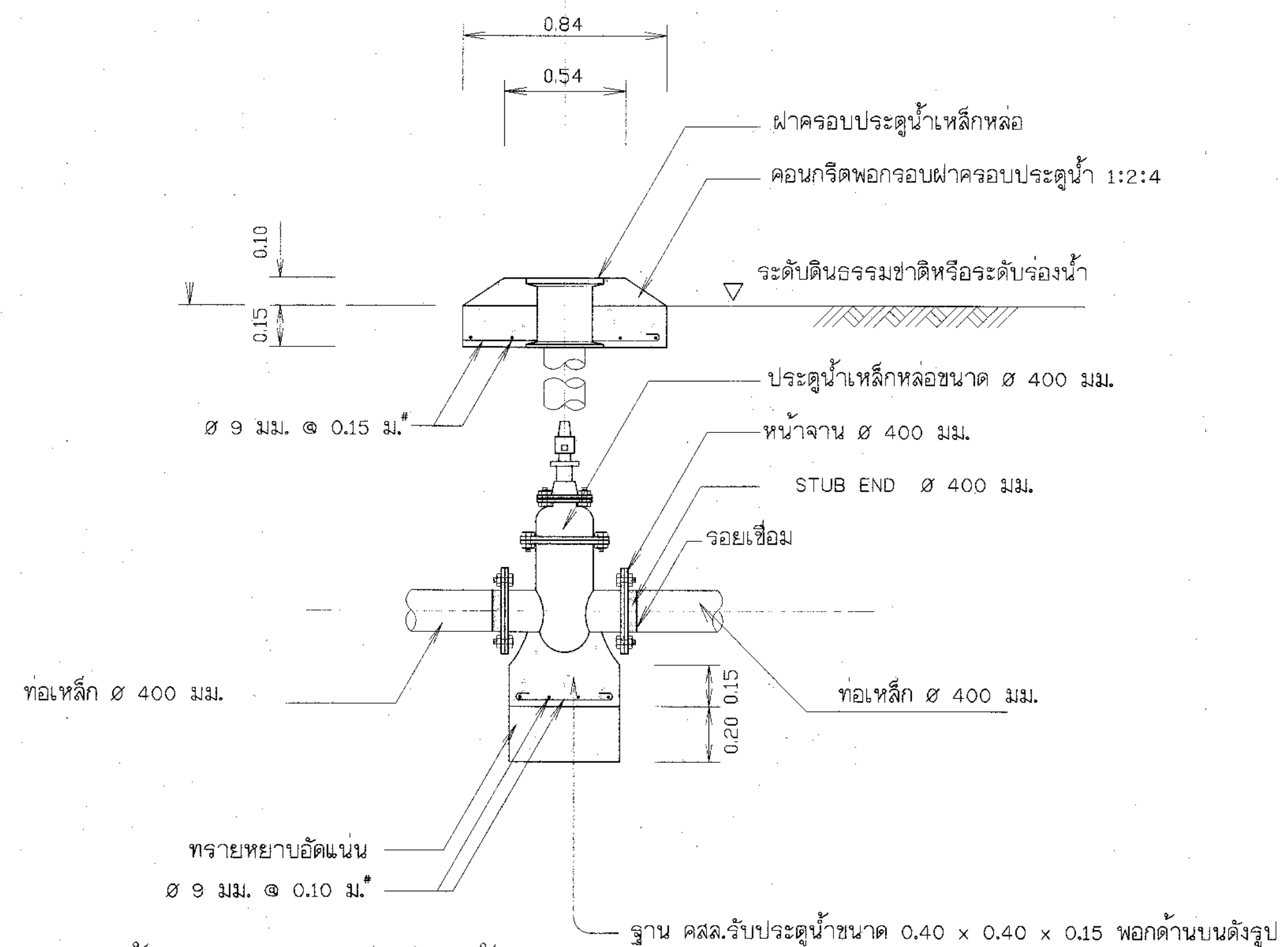
รูปตัด ก - ก แสดงการติดตั้งประตูกวควบคุมท่อย้ายน้ำ ขนาด 400 มม.
