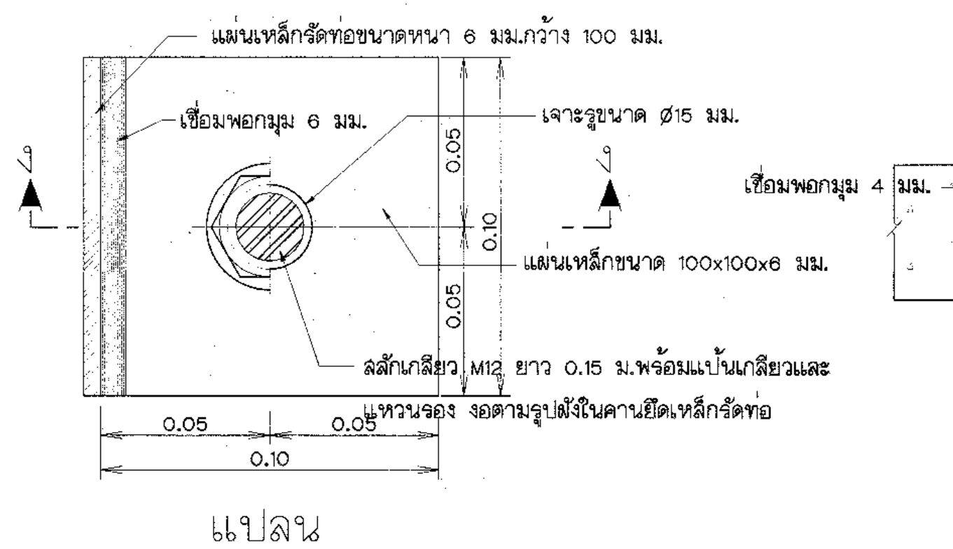
รายละเอียดแผ่นเหล็กยึดท่อ ไม่แสดงมาตราส่วน
