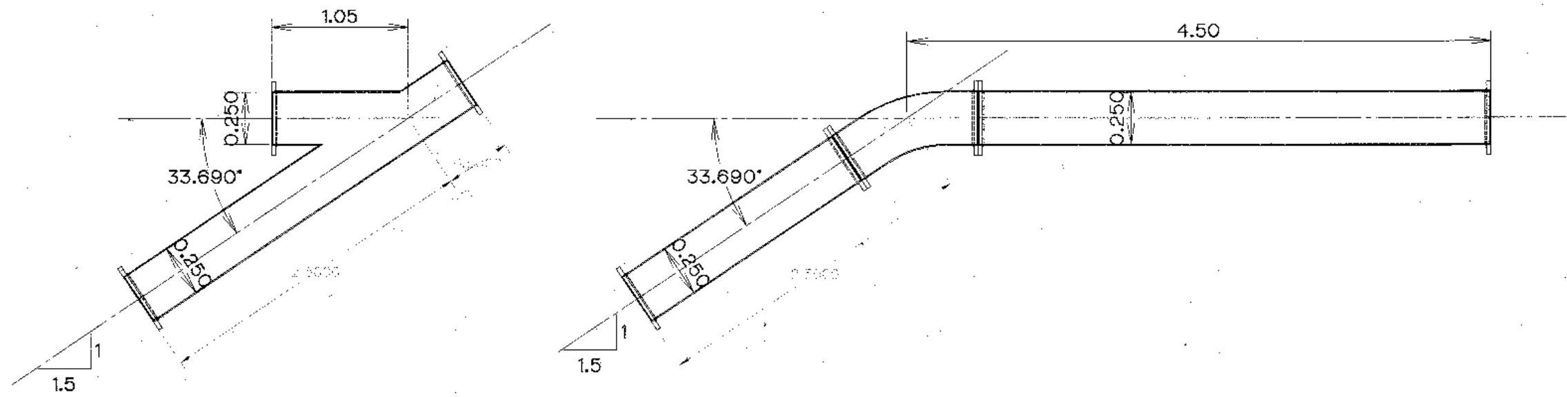
รายละเอียดทอริมตลิ่ง ลาด 1:1.5 มาตราส่วน 1 : 40
