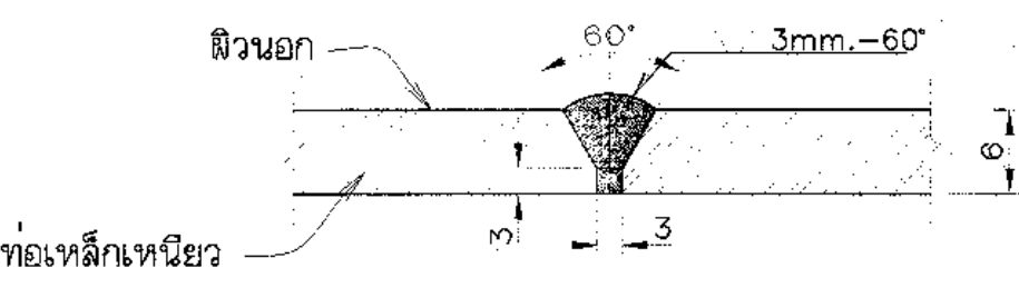
รูปขยายรอยเชื่อมท่อ ไม่แสดงมาตราส่วน
