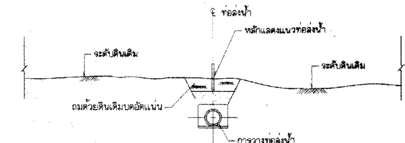
รูปตัดแสดงท่อลงน้ำ ไม่แสดงมาตราส่วน
