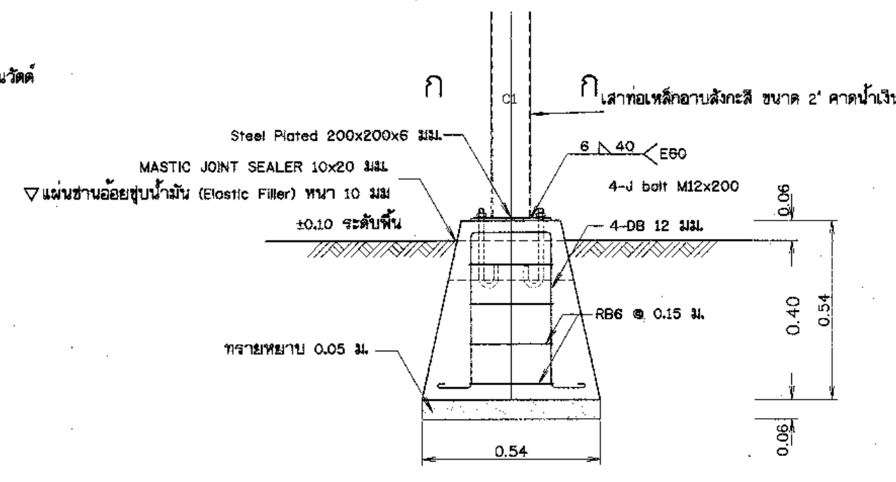
รูปขยายต่อม่อู่อุปไฟแสงสว่าง (ต่อม) คสล. หล่อสำเร็จรูปพร้อมติดตั้ง ไม่แสดงมาตรฐาน
