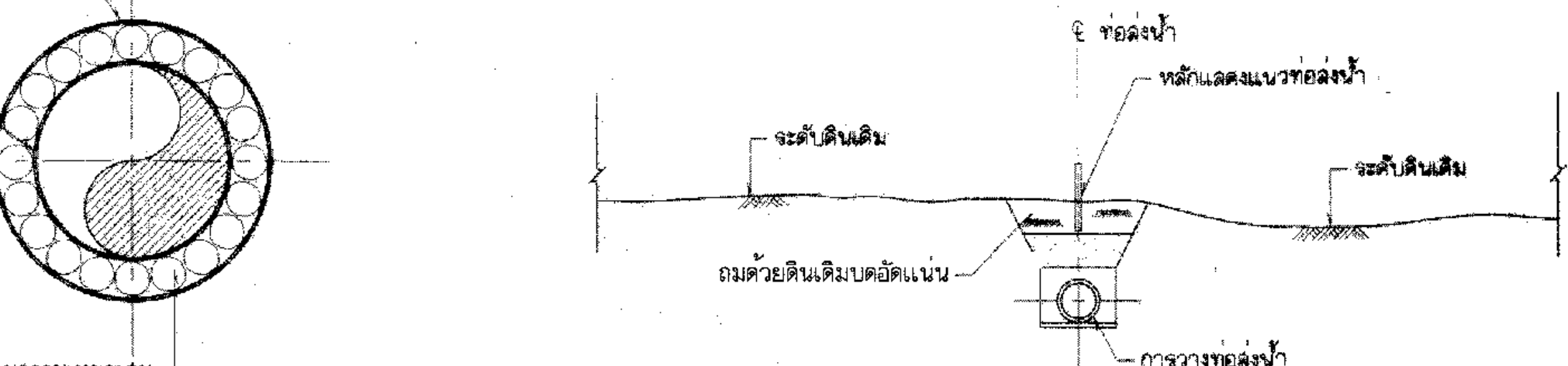
รูปตัดแสดงท่อลงน้ำ ไม่แสดงมาตราส่วน
