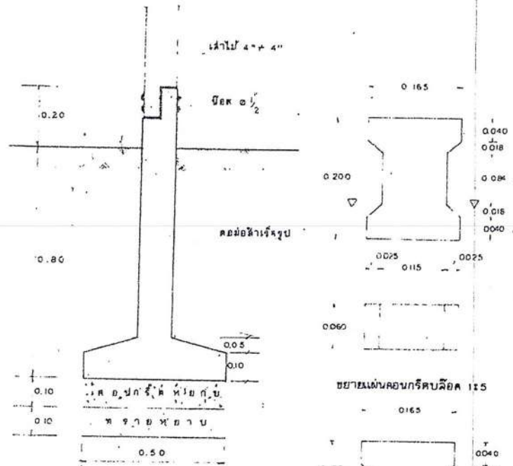
รูปขยายต่อม่อ 1810
