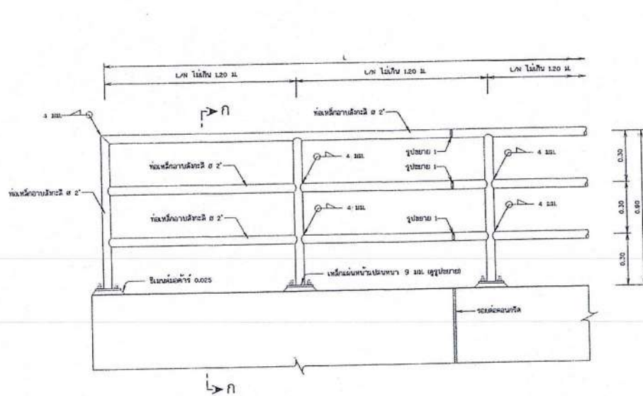
รูปขยายจาวเหล็กกันดก มาตราส่วน 1:10
