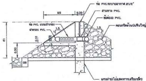
รูปตัด ช - ช
