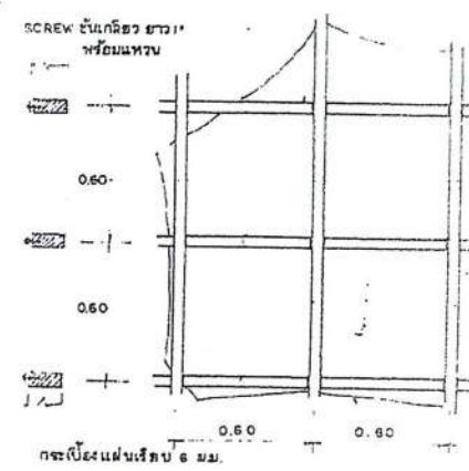
รูปขยายโครงฝ้า 1820
