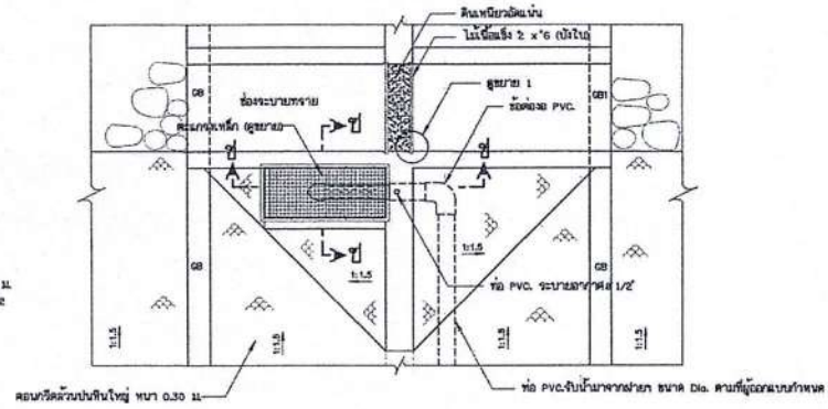
แปลนอาคารรับน้ำ
