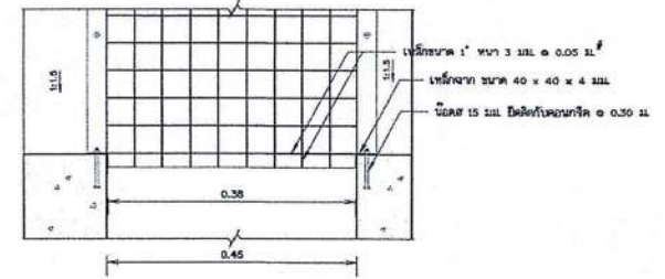
รูปตัด ข - ข
