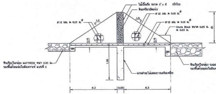
รูปตัด จ - จ
