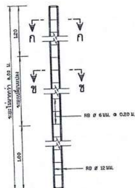
รายละเอียดเล่าป้าย คสล.
