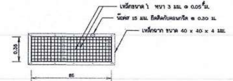
แปลนตะแกรงเหล็กกั้นสวะ
