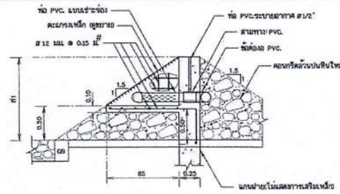
รูปตัด ซ - ซ
