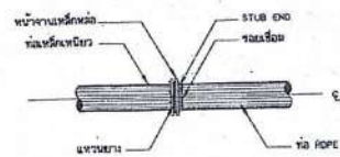
การบรรจุท่อหลักเหนียวกับท่อ HDPE
