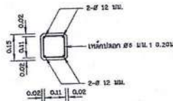
รูปตัด ข - ข
