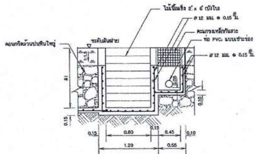
รูปตัด ฉ - ฉ
