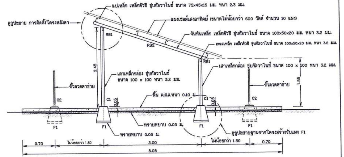
รูปด้านข้าง ไม่แสดงขนาดจั่วส่วน
