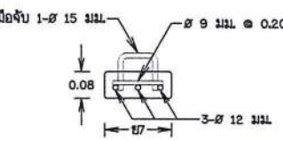
รูปตัดแนว 3 - 3
