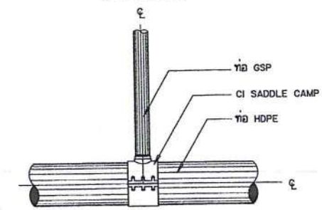
การบรรจุบ่อสามทาง HDPE กับท่อ GSP แบบ CI SADDLE CLAMP
