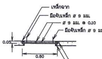
รูปตัดแนว 4 - 4
