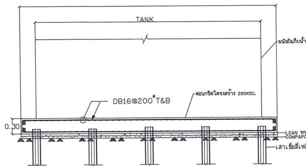
แบบตัด ก-ก scale NTC.
