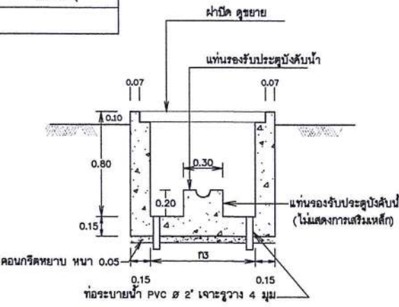
รูปตัด 2 - 2
