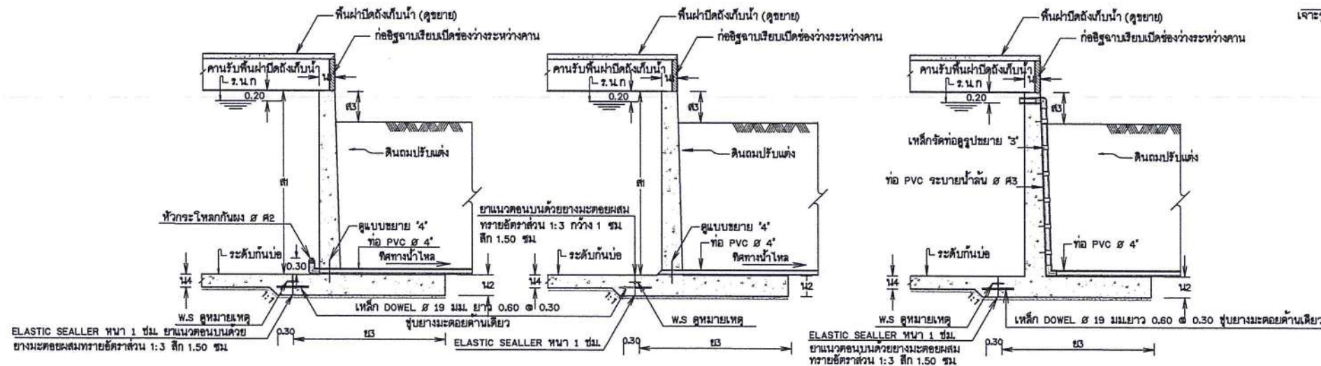
รูปตัดท่อส่งน้ำ
