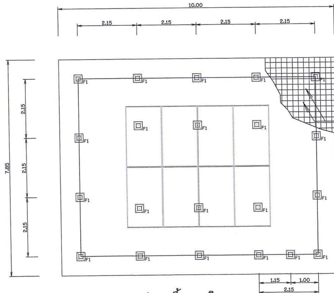
รูปขยายพื้นคอนกรีต ไม่แสดงขนาดจั่วส่วน
