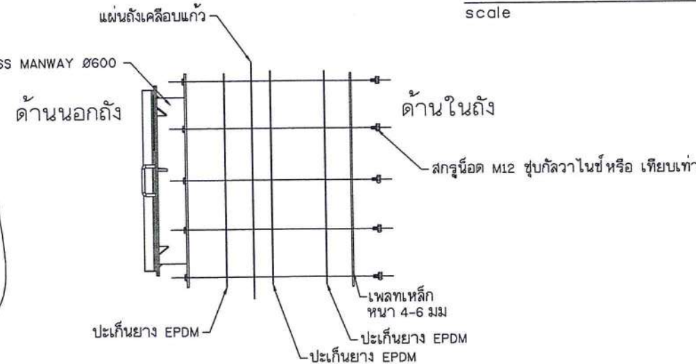
แบบขยายประตูตรวจสอบบำรุงรักษา scale NTC.
