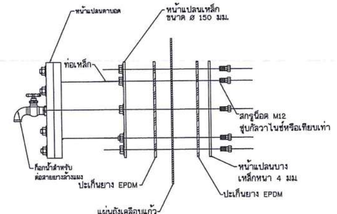
แบบขยายหน้าแปลนคานอด scale NTC.
