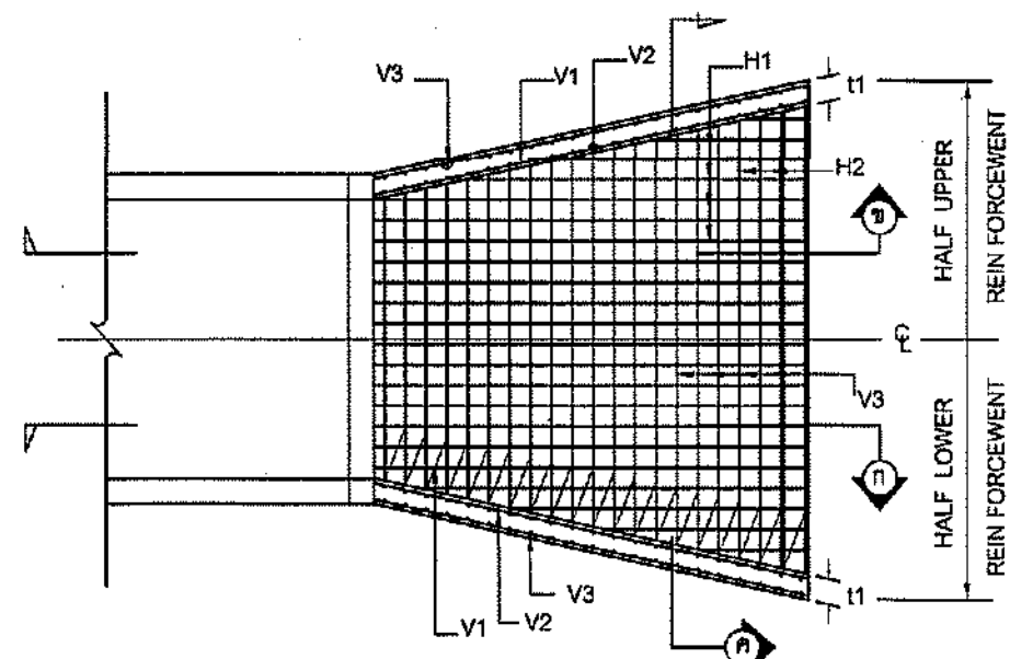
รูปตัด ๒ NOT TO SCALE
