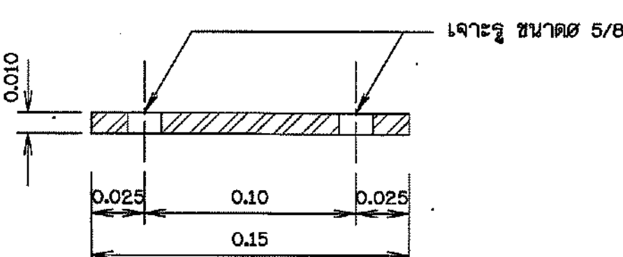
รูปตัด ค-ค
