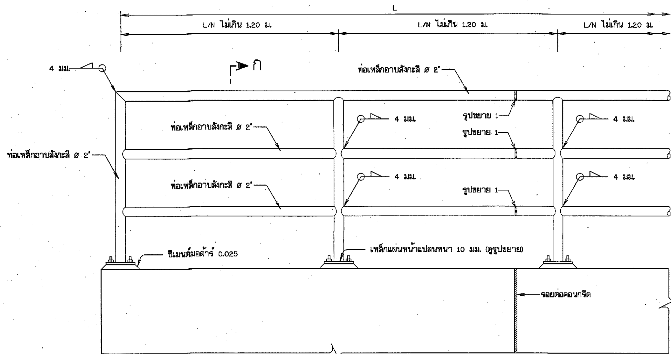
รูปขยายจาวเหล็กกันตก
