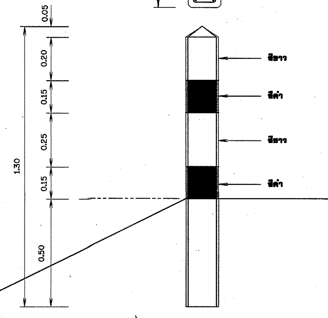
แบบขยายหลักกริมคันทัน
