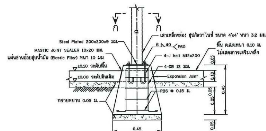
รูปขยายฐานรากโครงสร้างรับแผง F1 (ต่อม่อ คสล. หล่อสำเร็จรูปพร้อมติดตั้ง) ไม่แสดงมาดราส่วน
