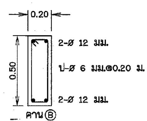
ขยายคาน B ไม่แสดงขนาดราส่วน
