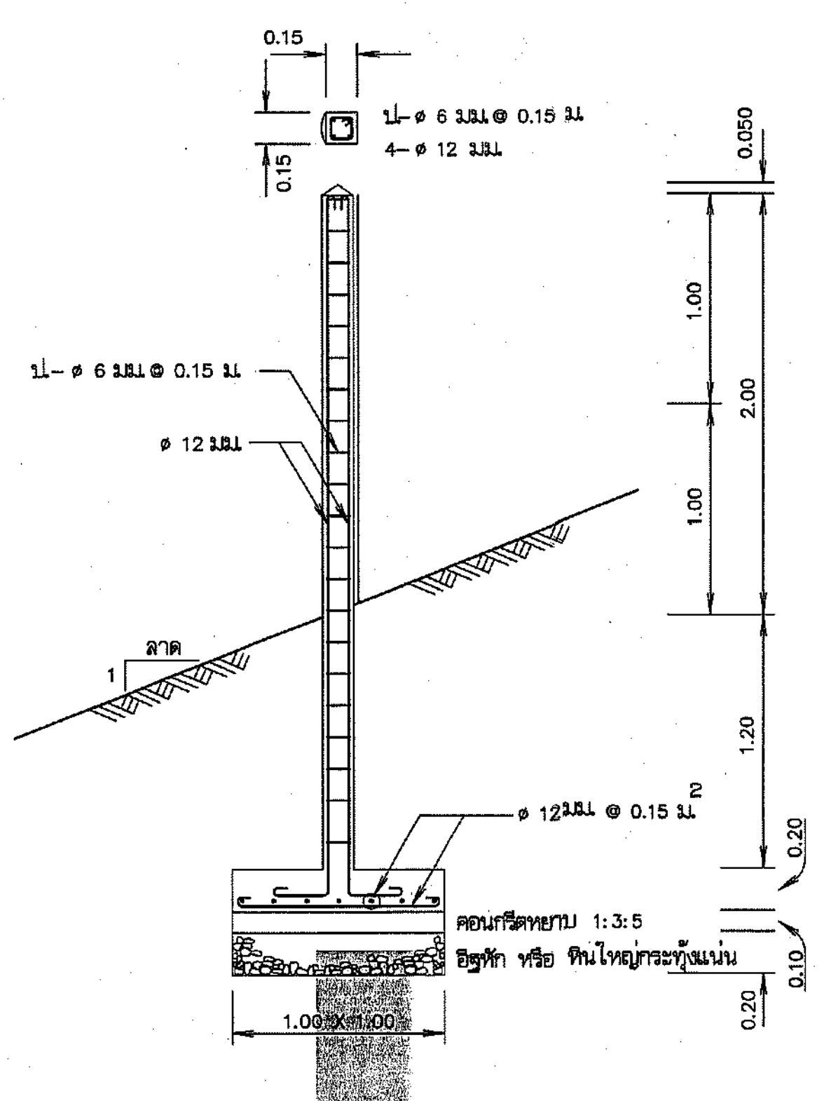
ขยายหลัก คสล.บอกระดับ มาตราส่วน 1:25
