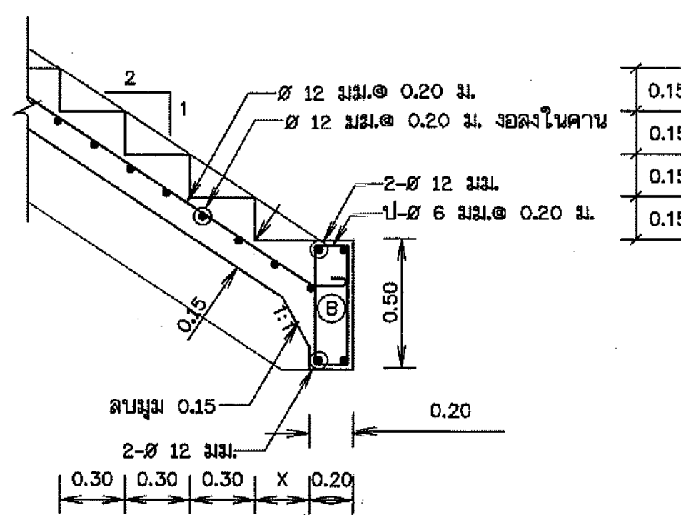
รูปขยาย 2 ไม่แสดงขนาดราส่วน
