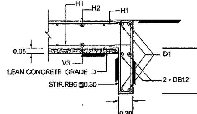
รูปตัด ๑๘ NOT TO SCALE
