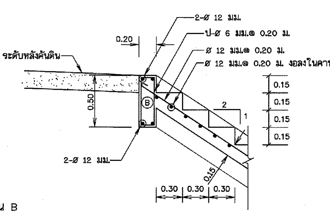
รูปขยาย 1 ไม่แสดงขนาดราส่วน
