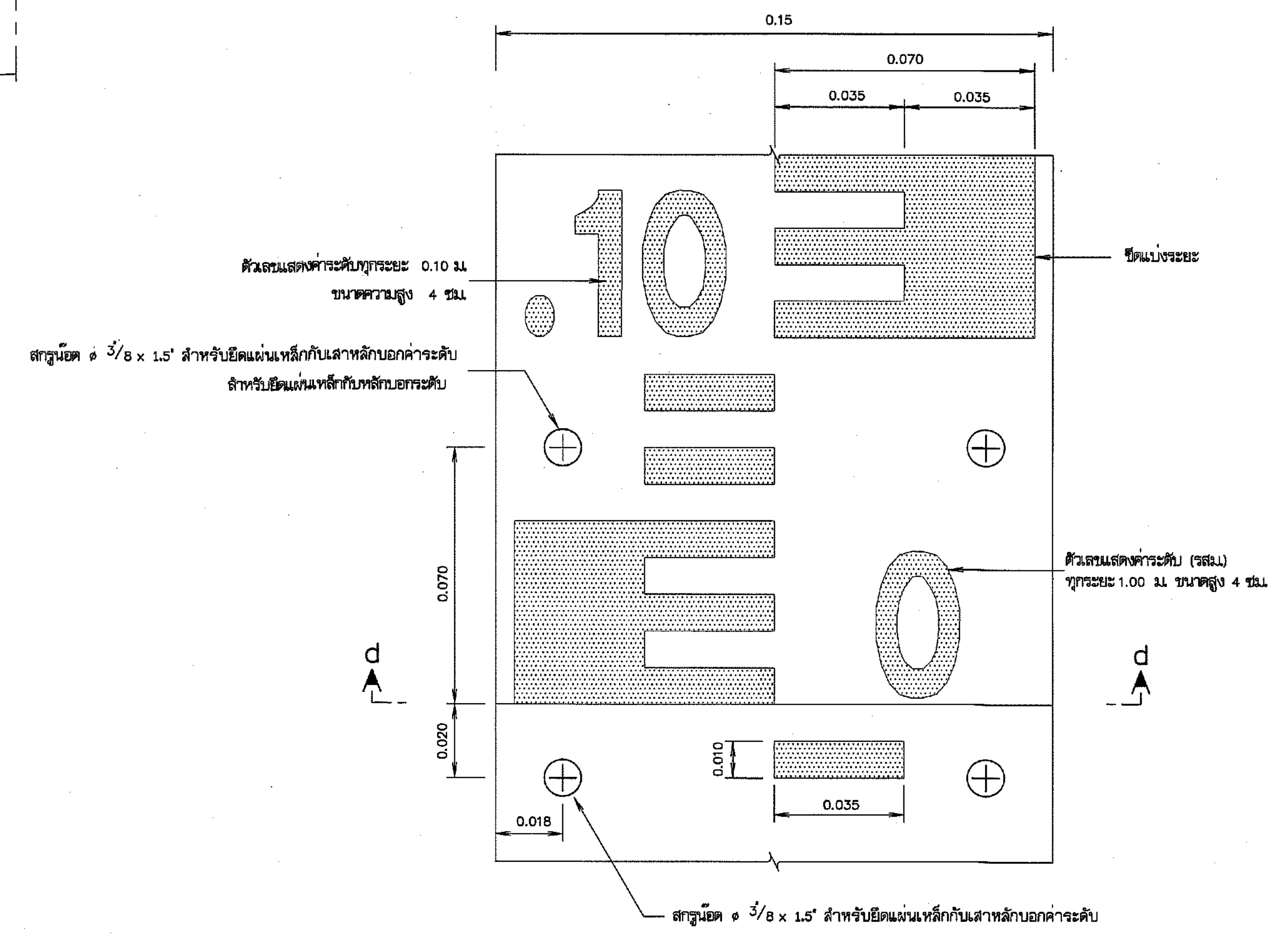
ขยายแผ่นเหล็กบอกระดับ มาตราส่วน 1:1
