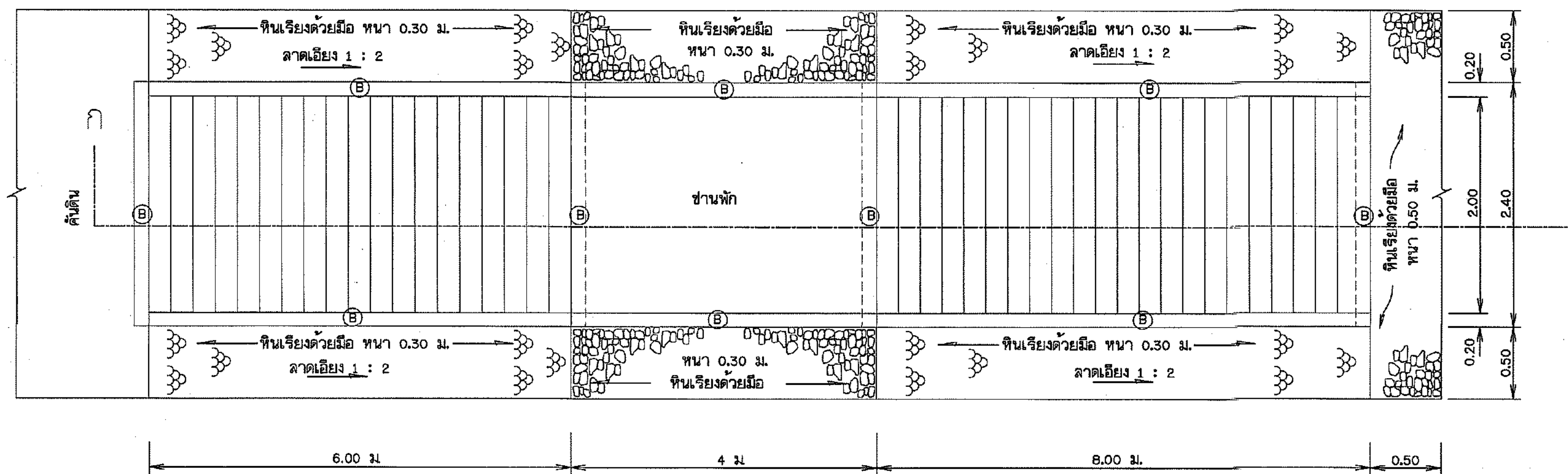
แปลนบ้าน ใต้ คสล. แบบมีชานพัก ไม่แสดงขนาดราส่วน
