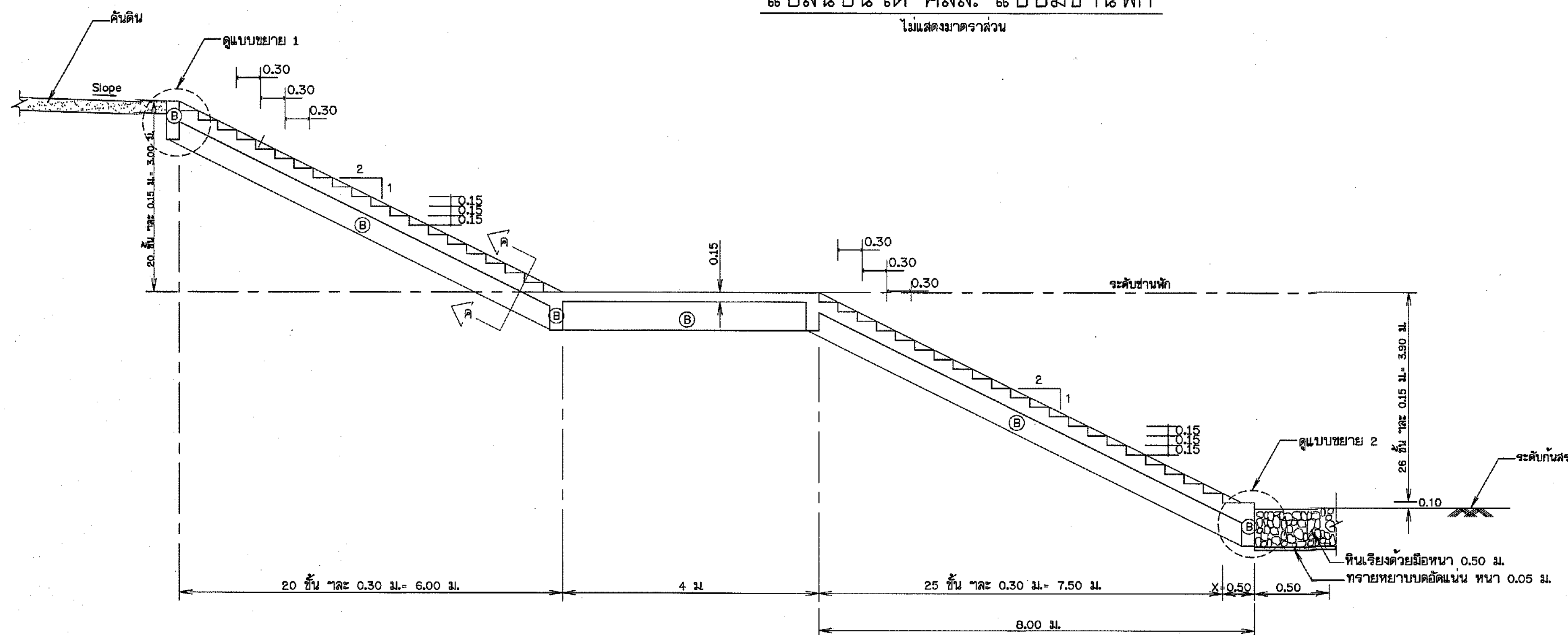
รูปตัด ก - ก ไม่แสดงขนาดราส่วน
