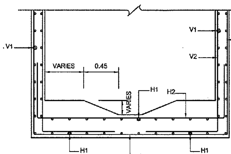
รูปตัด ๒๐ NOT TO SCALE
