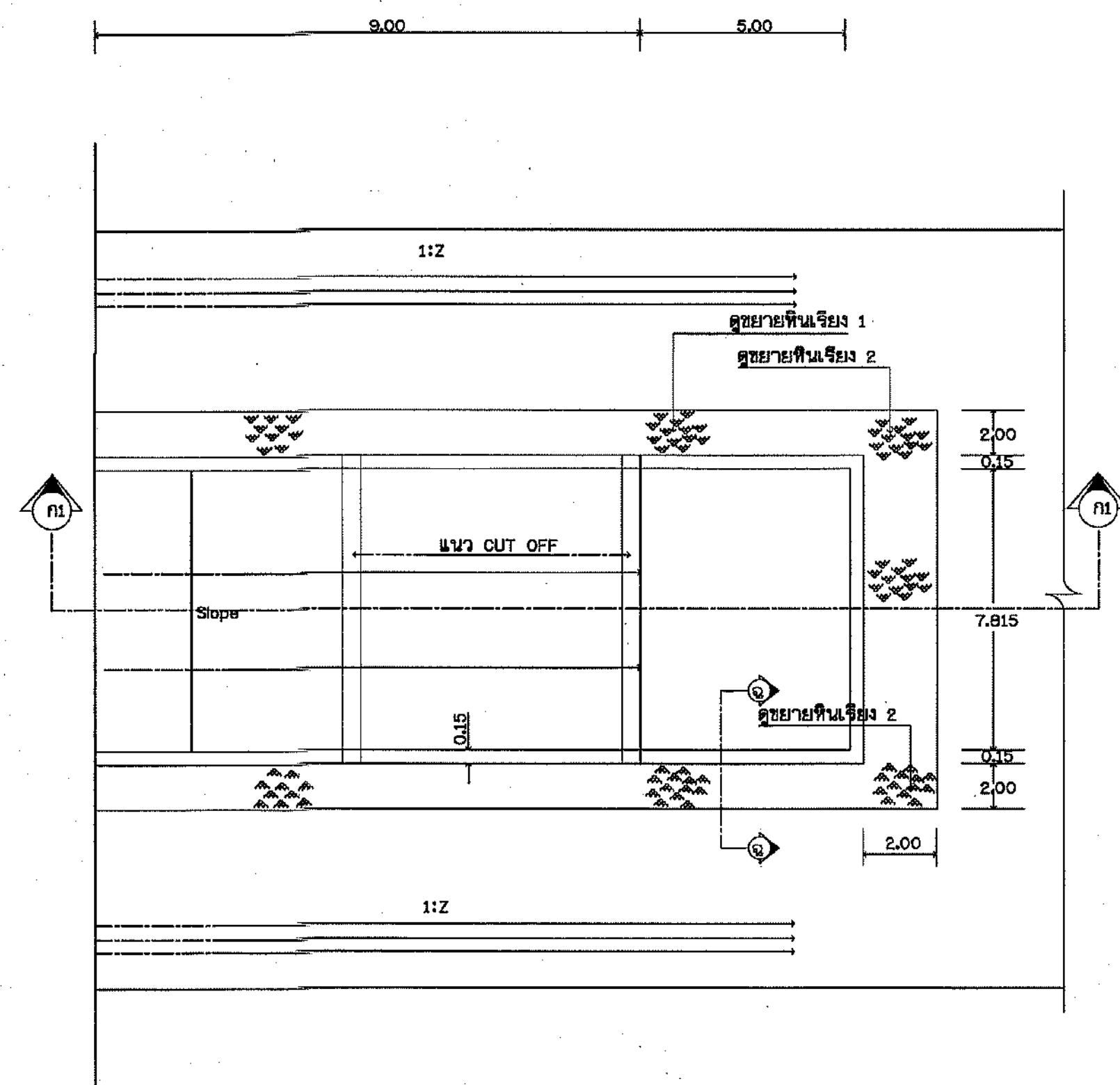
แปลนอาคารราง Chute (กรณีไม่มีขานพัก) ไม่แสดงมาตราส่วน
