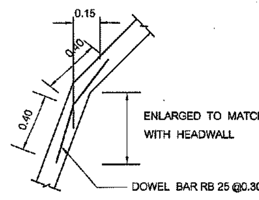
รูปตัด ๑๗ NOT TO SCALE
