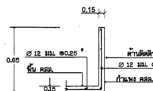
รูปตัด ๑-๑ (ความหนาพื้น 0.15 ม.) ไม่แสดงมาตราส่วน
