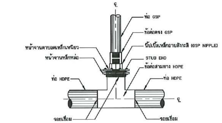
การบรรจุท่อสามทาง HDPE กับท่อ GSP แบบข้อต่อ สำหรับอาคารจุดปล่อยน้ำ อาคารประจวบประจวบตอน อาคารท่อระบายอากาศ กรณีท่อส่งน้ำขนาดเส้นผ่าศูนย์กลางมากกว่า 315 มม.
