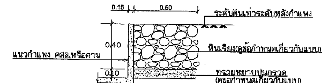
ขยายหินเรียง ๑ ไม่แสดงมาตราส่วน
