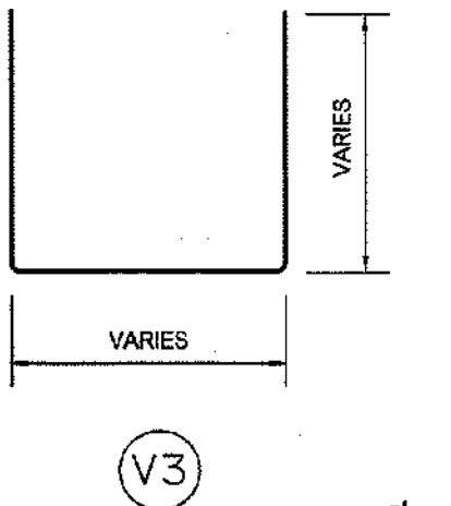
รายละเอียดเหล็กเส้น
