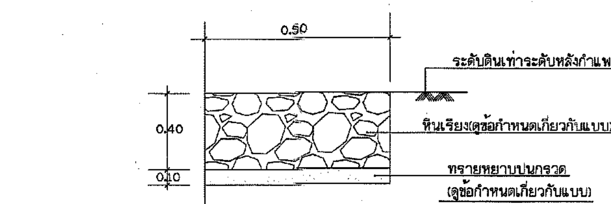
ขยายหินเรียง 2 ไม่แสดงขนาดราส่วน
