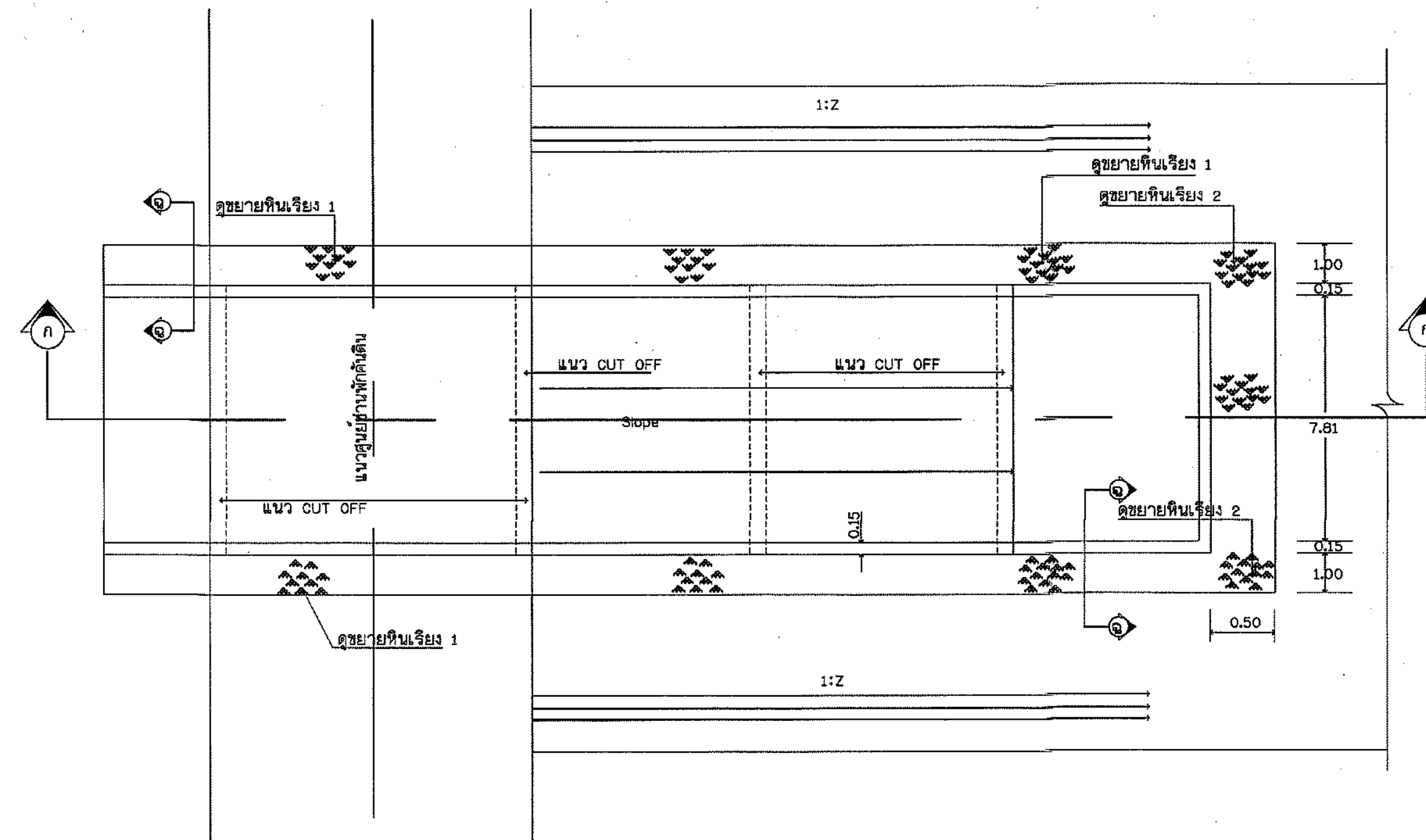
แปลนอาคารราง Chute (กรณีพื้น Box อยู่สูงกว่าระดับชั้นพัก) ไม่แสดงขนาดราส่วน
