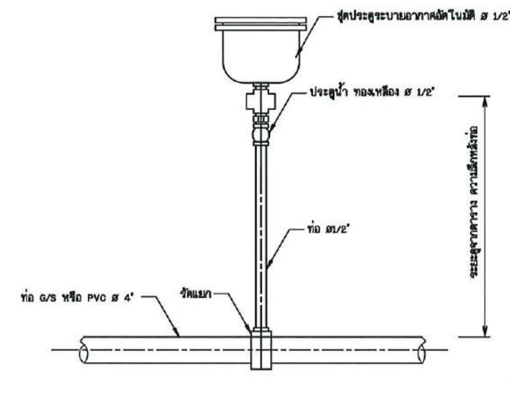
การติดตั้งประตูระบายอากาศอัดโบมบี ไม่แสดงมาตราส่วน
