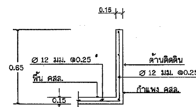
รูปตัด (ค)-(ค) (ความหนาพื้น 0.15 ม.) ไม่แสดงขนาดราส่วน
