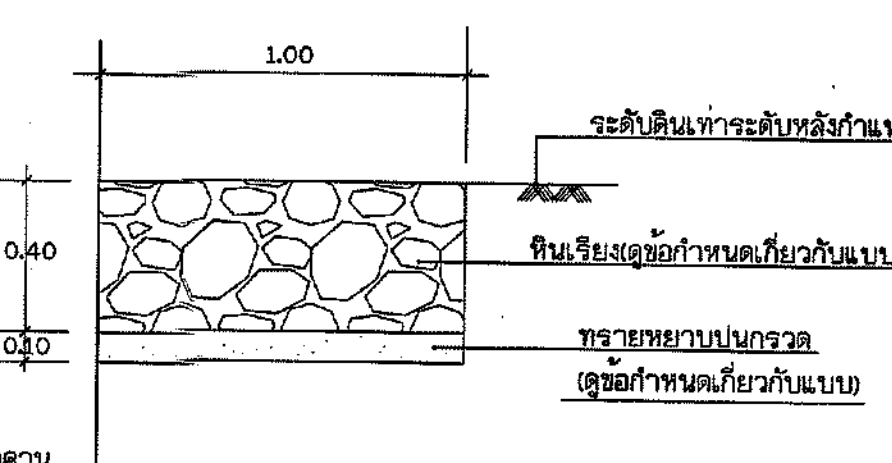
ขยายหินเรียง ๒ ไม่แสดงมาตราส่วน
