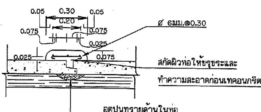
รูปตัด ๗-๗ ไม่แสดงมาตราส่วน
