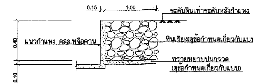
ขยายหินเรียง 1 ไม่แสดงขนาดราส่วน
