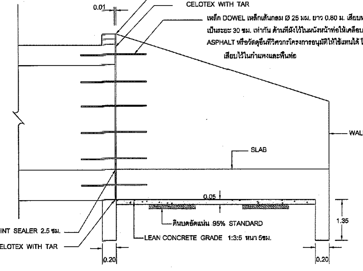
รายละเอียดรอยต่อเพื่อการขยายตัว
