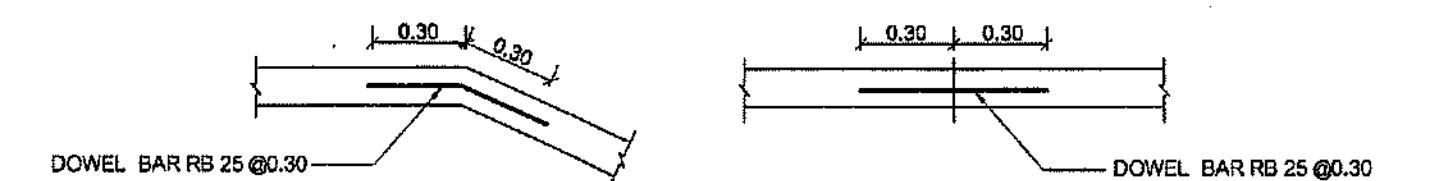
รายละเอียด ① ไม่แสดงขนาดราส่วน
