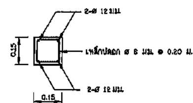
รูปตัด ก-ก ไม้ผสมมาตราช่วน
