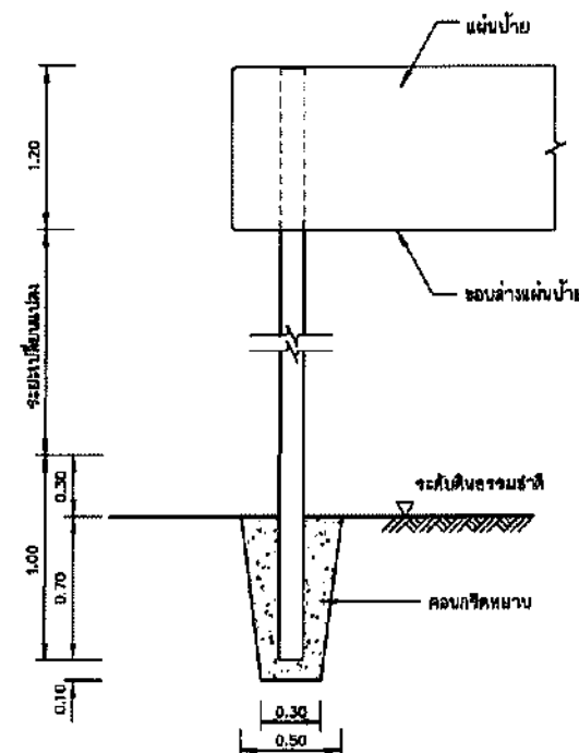
รายละเอียดการติดตั้งเสาป้าย ไม่แสดงมาตรฐาน
