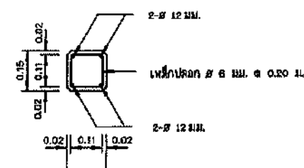
รูปตัด ข-ข ไม้ผสมขนาดยาว
