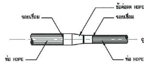
การบรรจุบ่อ HDPE กับข้อต่อ HDPE ไม่แสดงขนาดราส่วน
