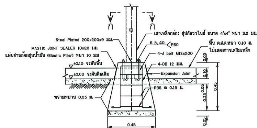
รูปขยายฐานรากโครงสร้างรับแผง F1 (ต่อม่อ คสล. ห่อผ้าสำเร็จรูปพร้อมติดตั้ง) ไม่แสดงขนาดจั่วส่วน
