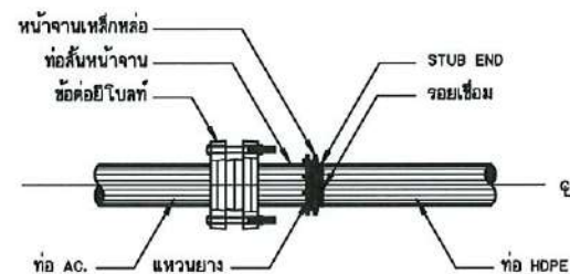
การบรรจุบ่อ AC. กับท่อ HDPE ไม่แสดงขนาดราส่วน
