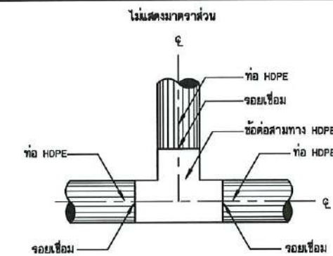
การบรรจุบ่อสามทาง HDPE กับท่อ HDPE ไม่แสดงขนาดราส่วน
