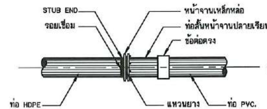
การบรรจุบ่อ HDPE กับท่อ PVC. ไม่แสดงขนาดราส่วน
