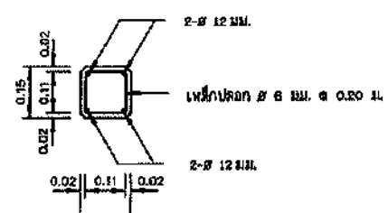
รูปตัด ข-ข ไม่แสดงขนาดจริง
