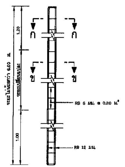
รายละเอียดเสาป้าย คสล. ไม่แสดงขนาดจริง
