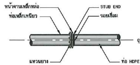
การบรรจุบ่อเหล็กเหนียวกับท่อ HDPE ไม่แสดงขนาดราส่วน
