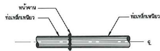
การบรรจุบ่อเหล็กเหนียวกับท่อเหล็กเหนียว ไม่แสดงขนาดราส่วน
