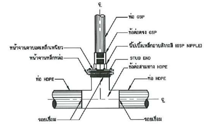
การบรรจุบ่อสามทาง HDPE กับท่อ GSP แบบข้อต่อ สำหรับอาคารจุดปล่อยน้ำ อาคารประตูดระบายตะกอน อาคารท่อระบายอากาศ กรณีท่อส่งน้ำขนาดเส้นผ่าศูนย์กลางมากกว่า 315 มม.
