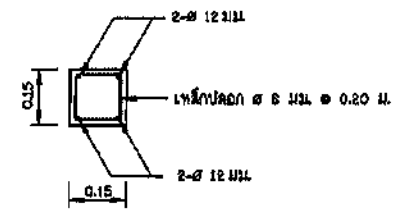
รูปตัด ก-ก ไม่แสดงขนาดจริง
