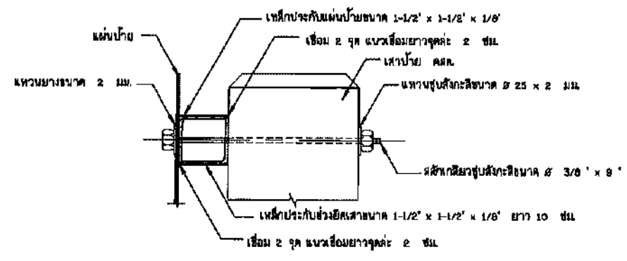
รูปตัดขยายการยึดแผ่นป้ายและเสา ไม่แสดงขนาดจริง
