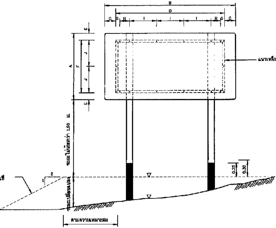
รูปแสดงการประกอบแผ่นป้าย ไม่แสดงขนาดจริง
