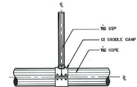
การบรรจุบ่อสามทาง HDPE กับท่อ GSP แบบ CI SADDLE CLAMP สำหรับอาคารจุดปล่อยน้ำ อาคารประตูดระบายตะกอน อาคารท่อระบายอากาศ กรณีท่อส่งน้ำขนาดเส้นผ่าศูนย์กลางน้อยกว่าหรือเท่ากับ 315 มม.
