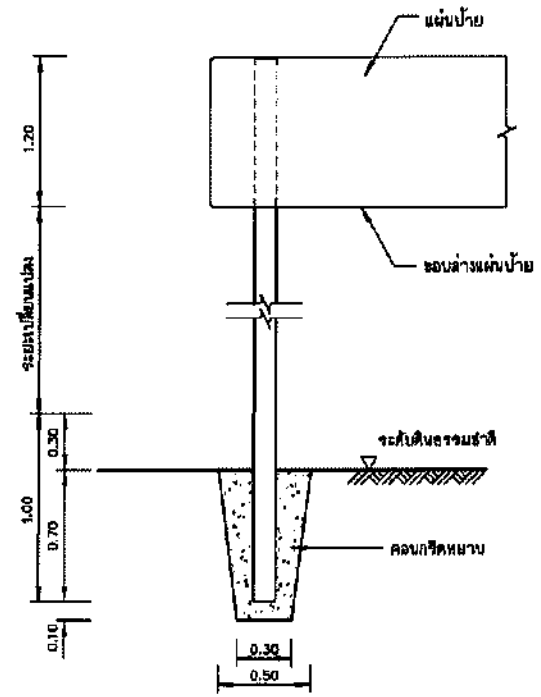
รายละเอียดการติดตั้งเสาป้าย ไม่แสดงขนาดจริง
