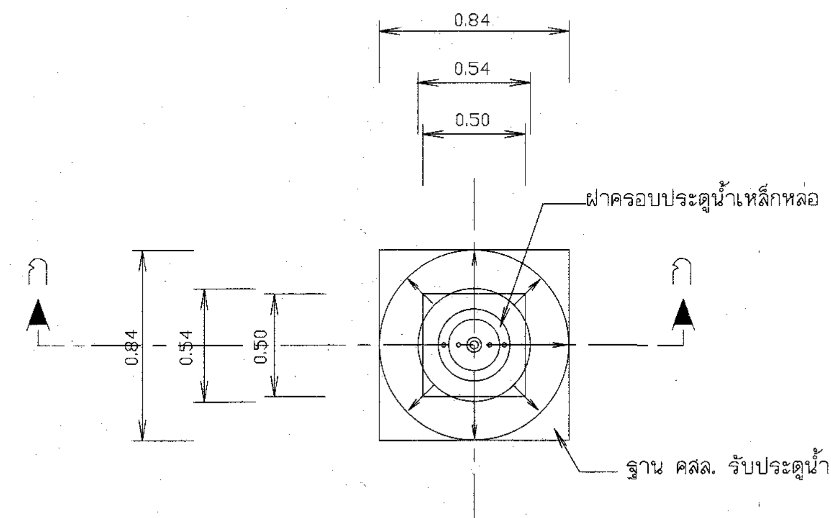
แปลนแสดงจุดติดตั้งประตูกวควบคุมท่อจ่ายน้ำ ขนาด 400 มม.
