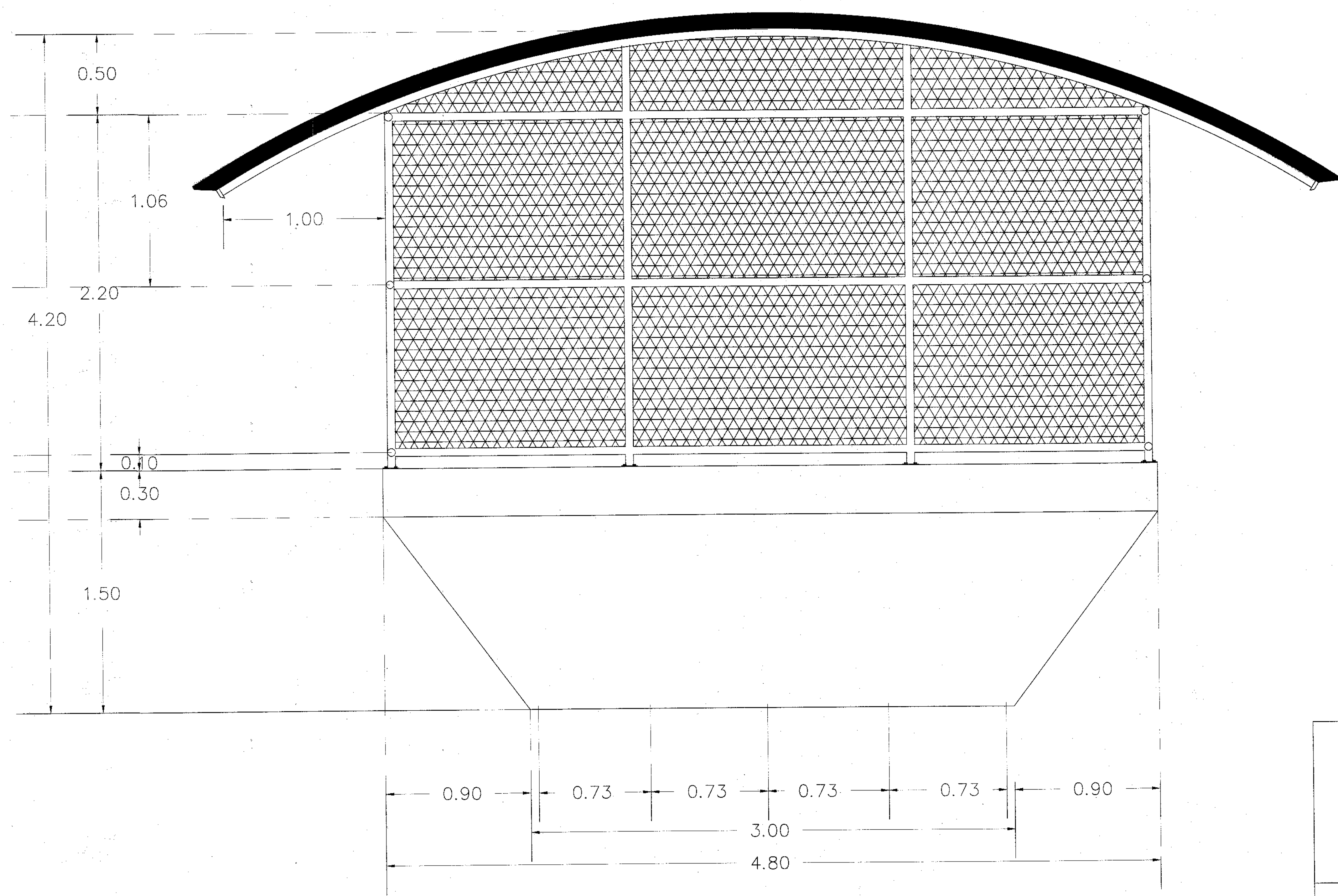
รูปด้านหลัง
