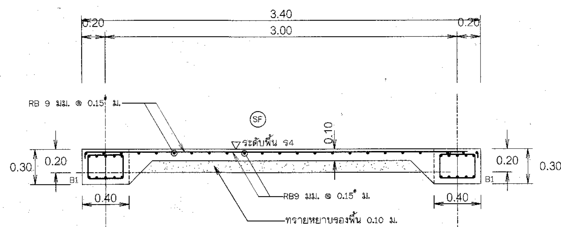
รูปตัด ก1 - ก1
