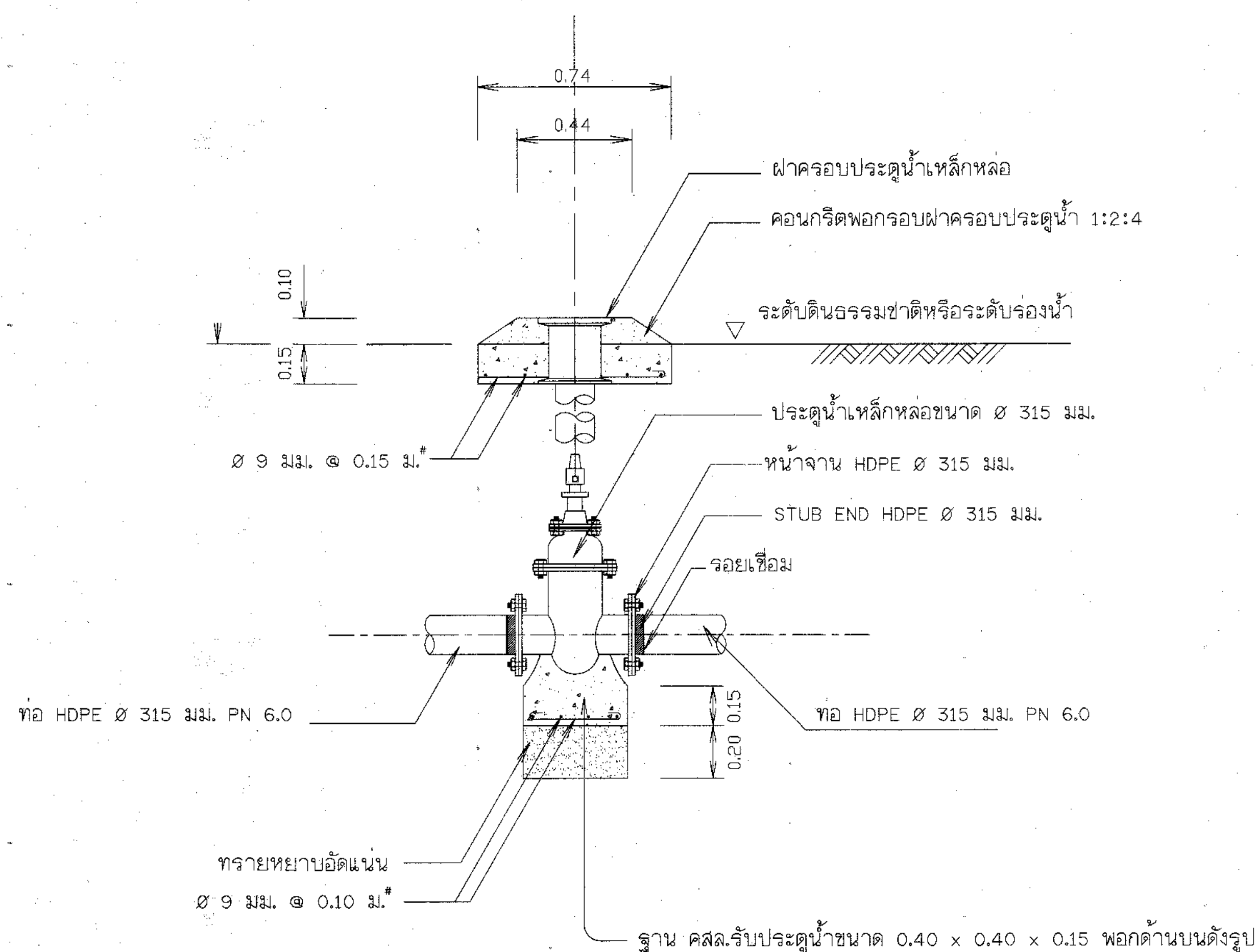
รูปตัด ก - ก แสดงการติดตั้งประตูกวควบคุมท่อจ่ายน้ำ ขนาด 315 มม.
