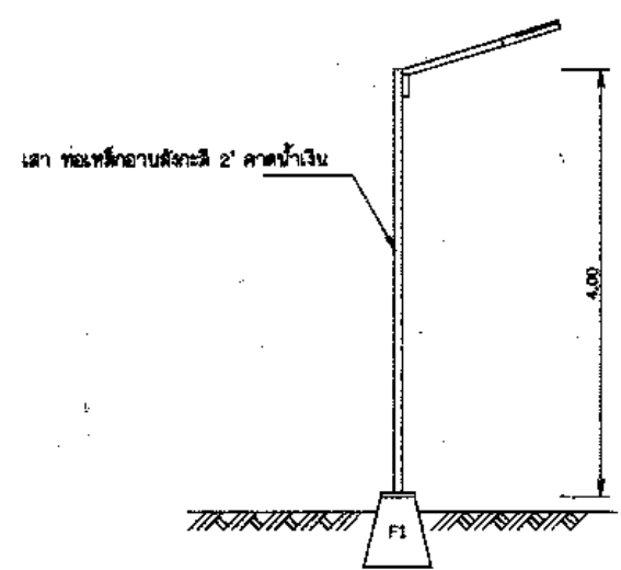
แบบเสาไฟ
