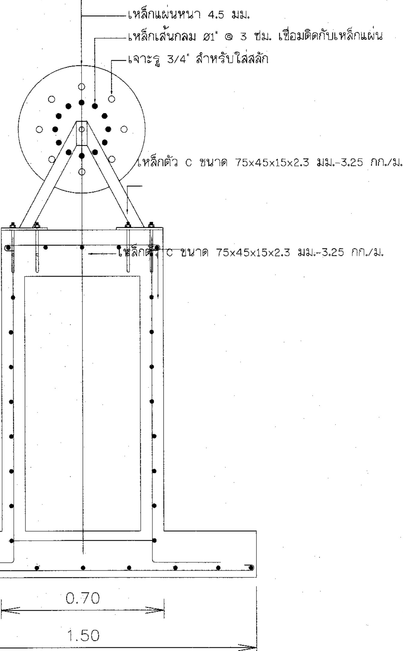
รูปตัด 2-2 ไม่แสดงมาตราส่วน
