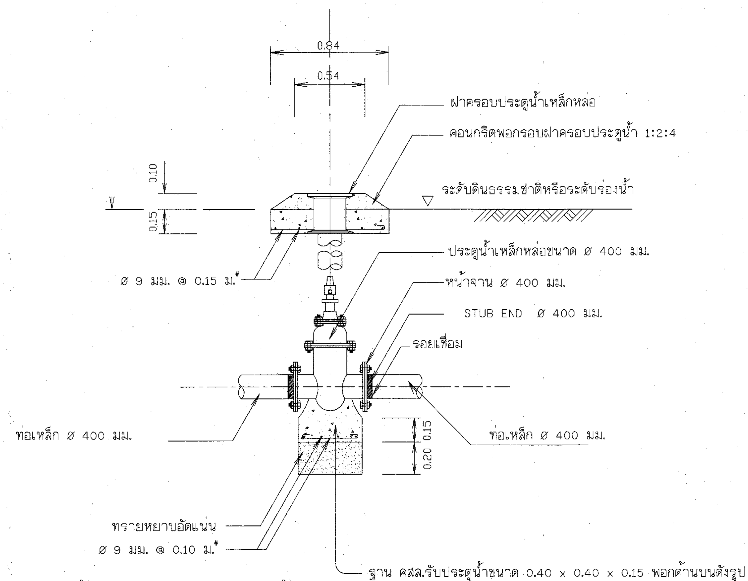
รูปตัด ก - ก แสดงการติดตั้งประตูกวควบคุมท่อจ่ายน้ำ ขนาด 400 มม.
