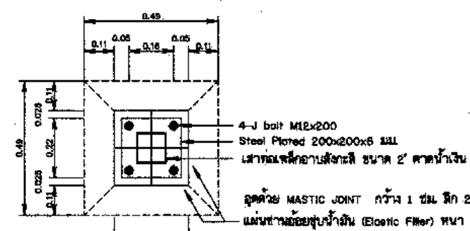
รูปตัด ก-ก
