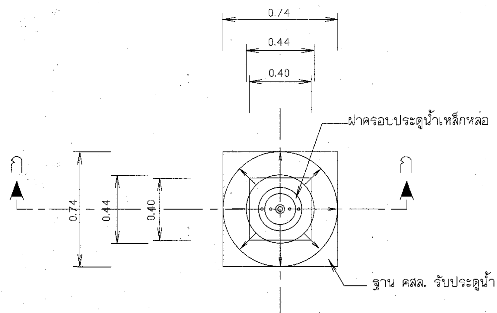
แปลนแสดงจุดติดตั้งประตูกวควบคุมท่อจ่ายน้ำ ขนาด 315 มม.
