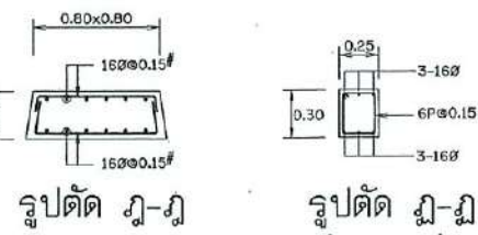
การเสริมเหล็ก ตอม่อแบบที่ 3
