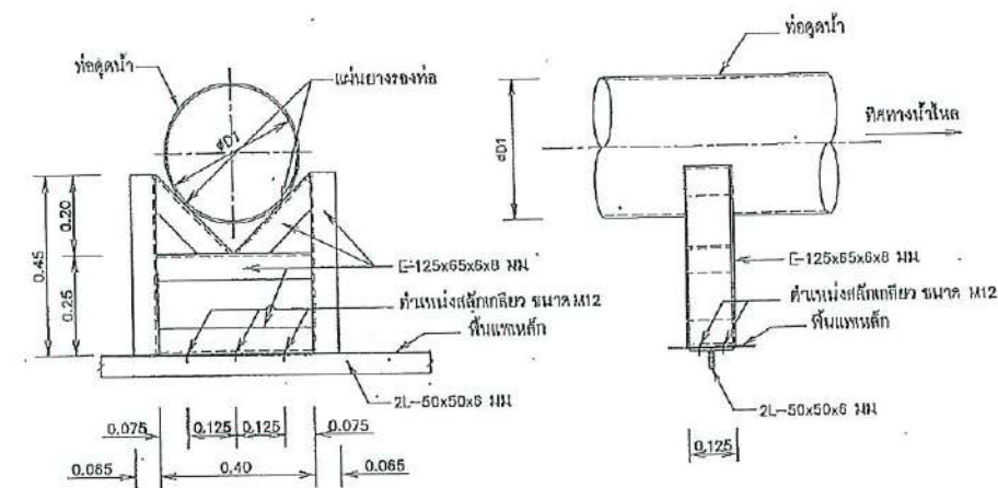
รูปขยาย SUPPORT "A" ไม่แสดงขนาดตัว
