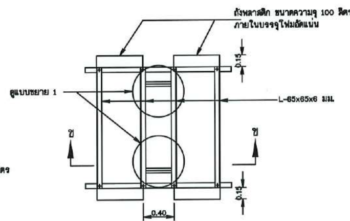
ท่อนรับท่อวางตัวนอน
