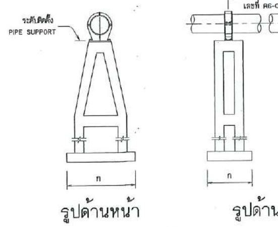
ตอม่อรับท่อแบบที่ 3,4 มาตรฐาน
