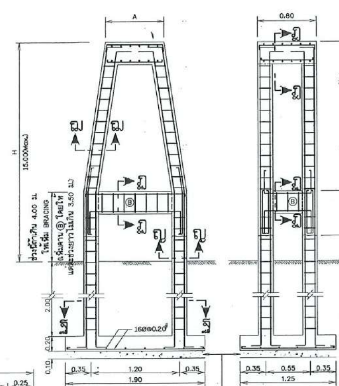
ตอม่อรับท่อแบบที่ 1 มาตรฐาน
