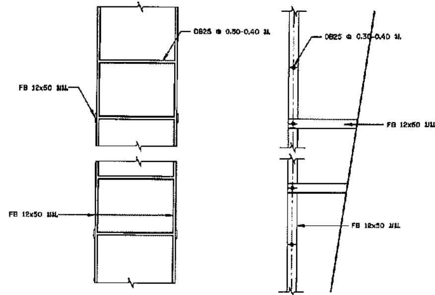
แบบขยายบันได ภายในท่อถึงสูง ไม่แสดงขนาดจั่วหัว
