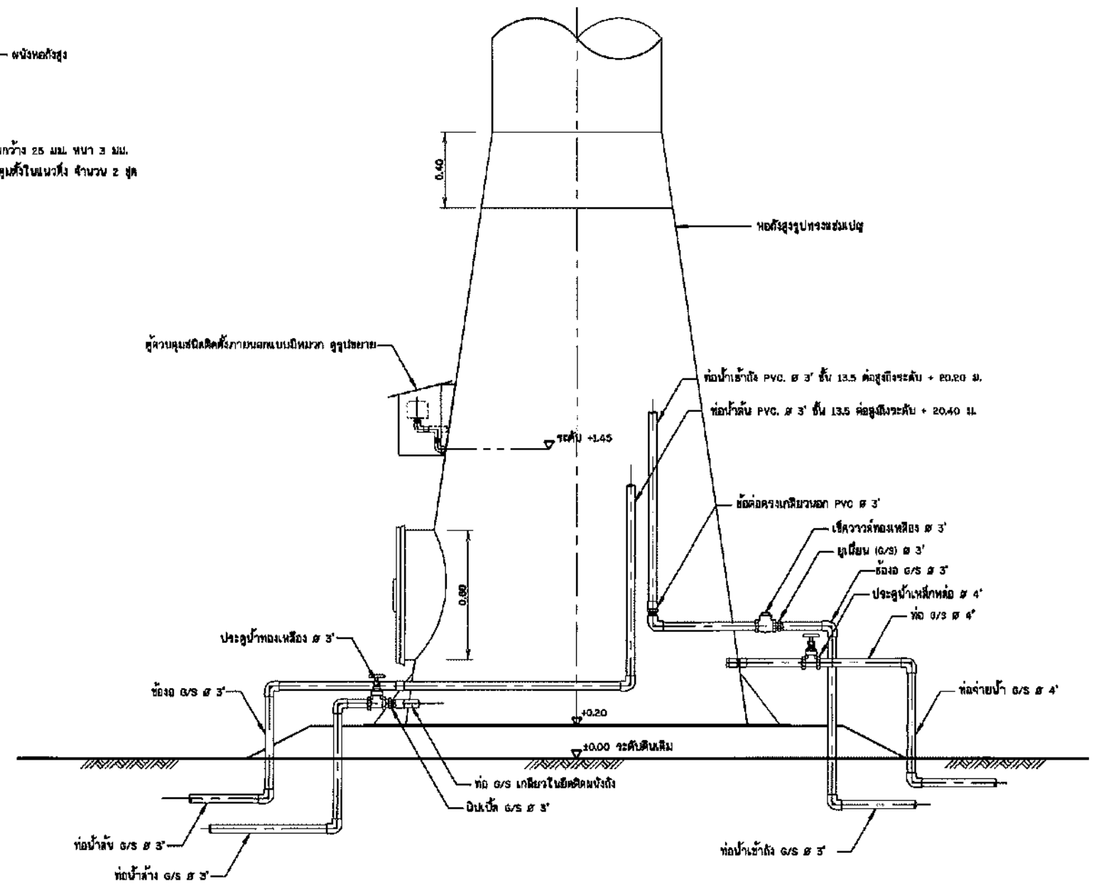
แบบแสดงการเดินท่อในท่อถึงสูง ไม่แสดงขนาดจั่วหัว
