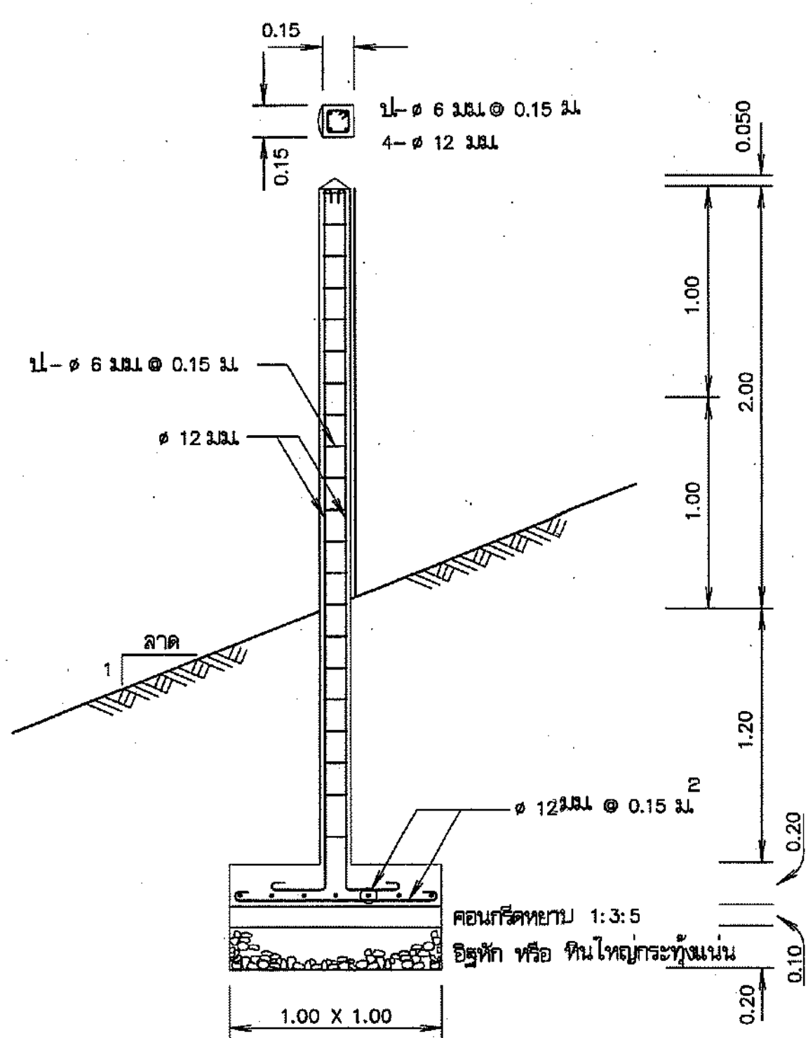
ขยายหลัก คลองบ่อค่าระดับ
