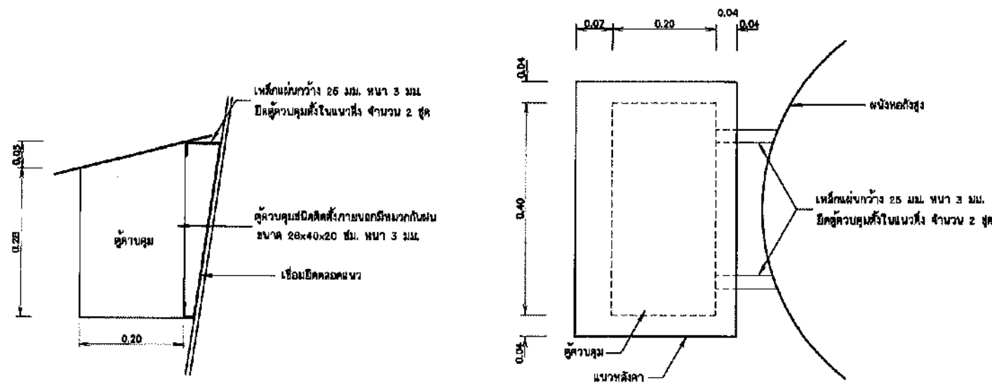
แบบขยายตัวควบคุม ไม่แสดงขนาดจั่วหัว
