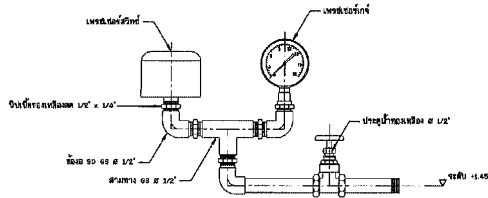
แบบขยายสวิตช์ควบคุมและเกจวัดความดัน ไม่แสดงขนาดจั่วหัว
