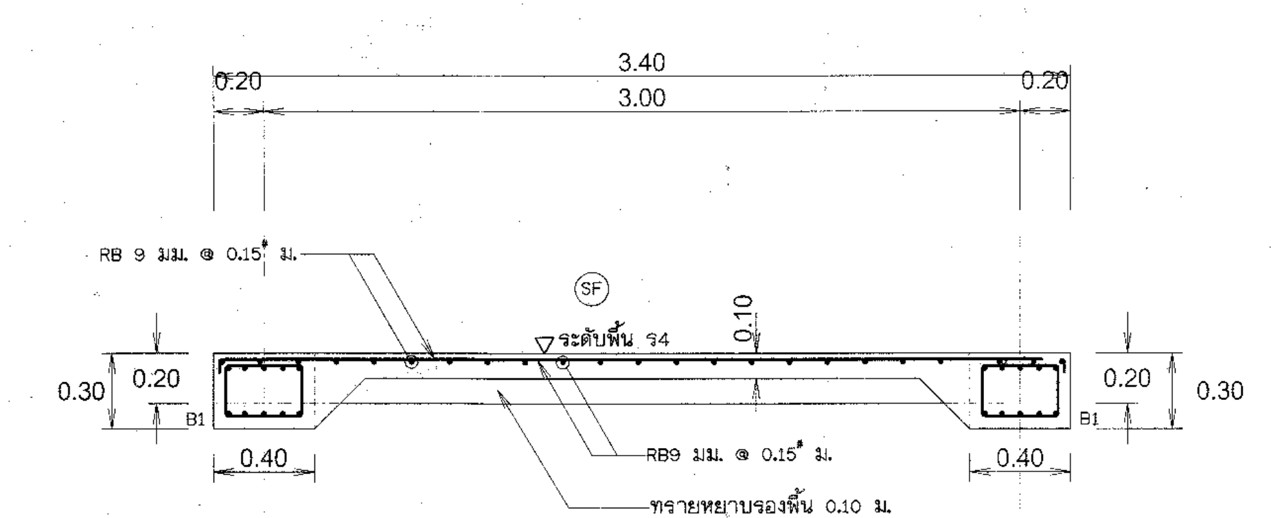
รูปตัด ก1 - ก1
