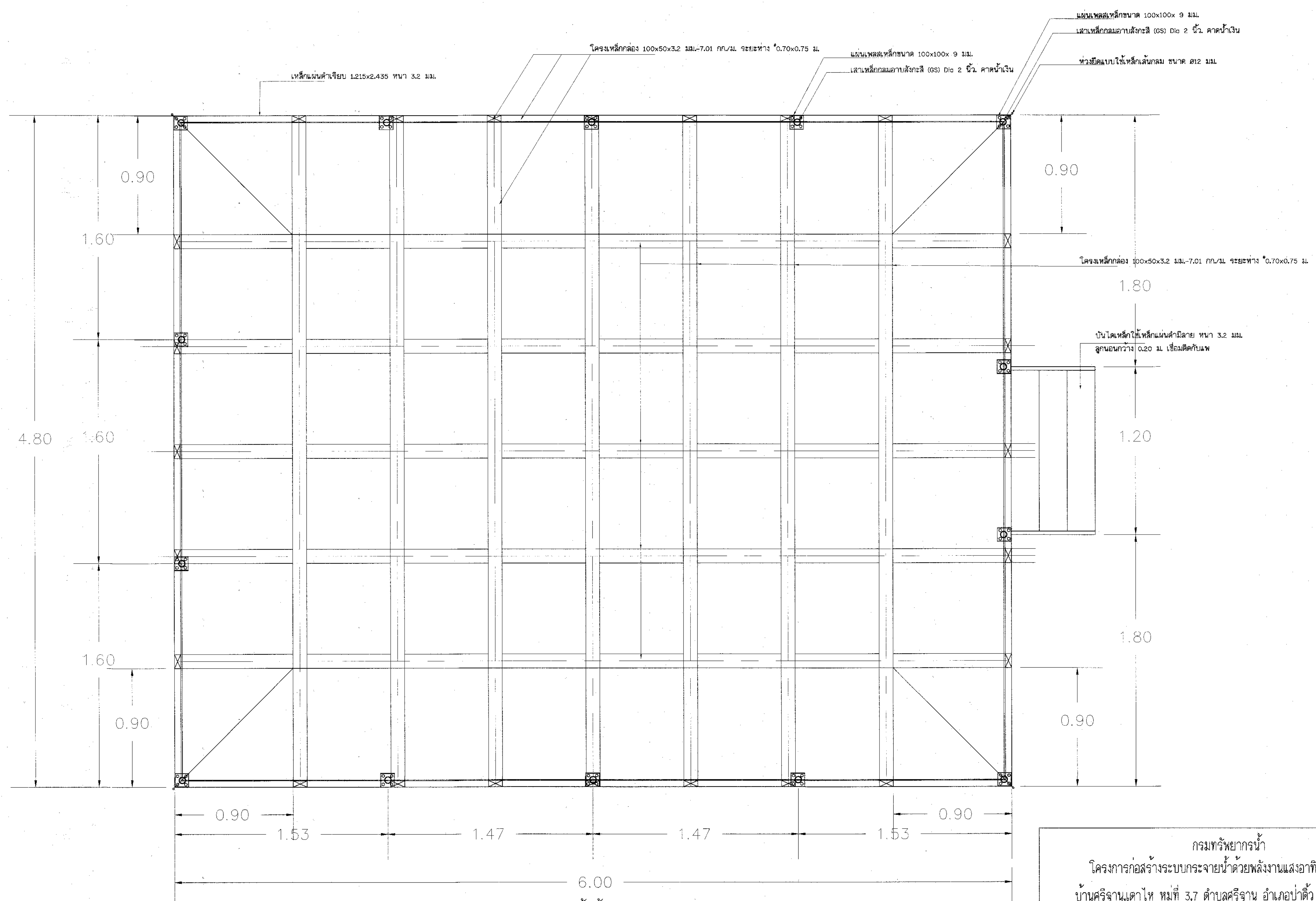
แปลน โครงพื้นที่ถังแพลลอย มาตราส่วน 1:100
