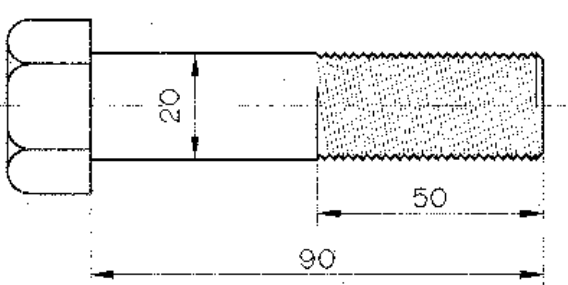
สลักเกลียวขนาด M20 ไม่แสดงมาตราส่วน
