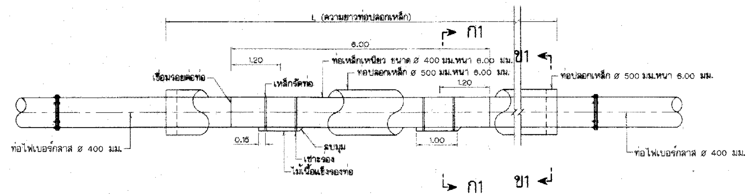
รูปตัดแสดงมาตรฐานการวางท่อเหล็กเหนียวในท่อปลอกเหล็กถนนลาดยาง ไม่แสดงมาตราส่วน
