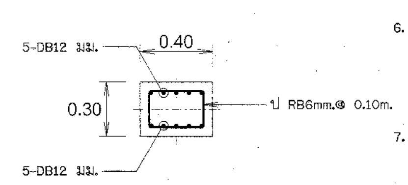
แบบขยายคาน B1
