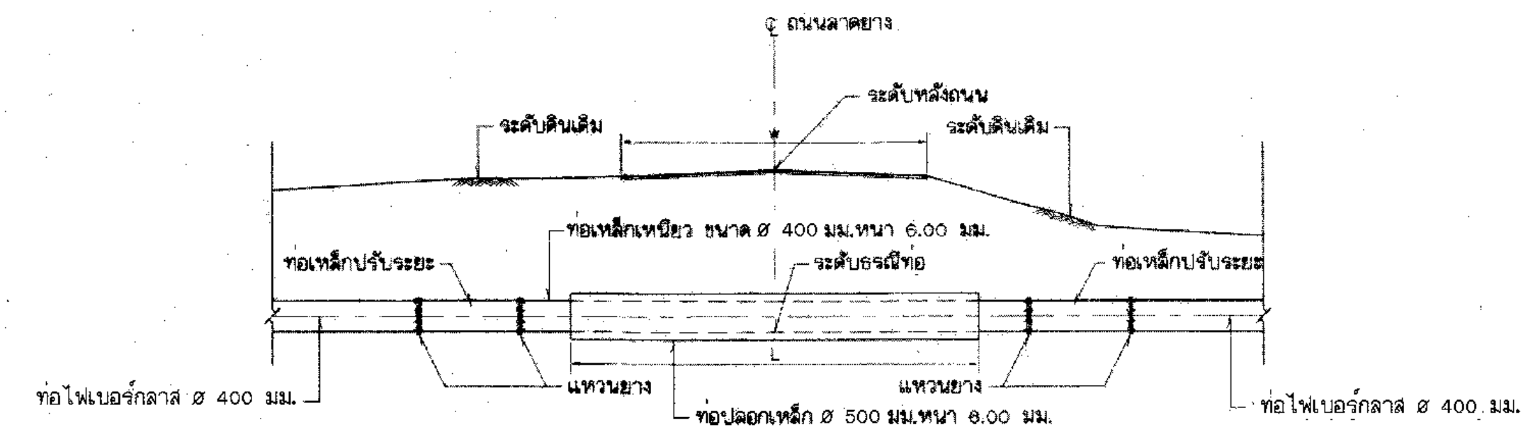
รูปตัดตามยาวแนว ก ท่อลอดถนนลาดยาง ไม่แสดงมาตราส่วน
