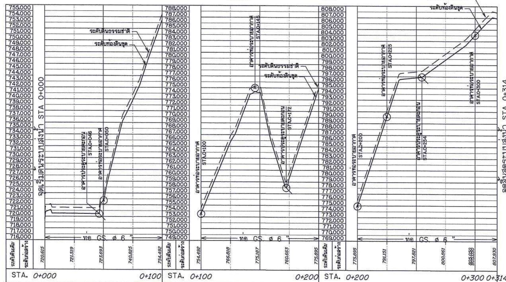
รูปตัดตามแนวยาว
