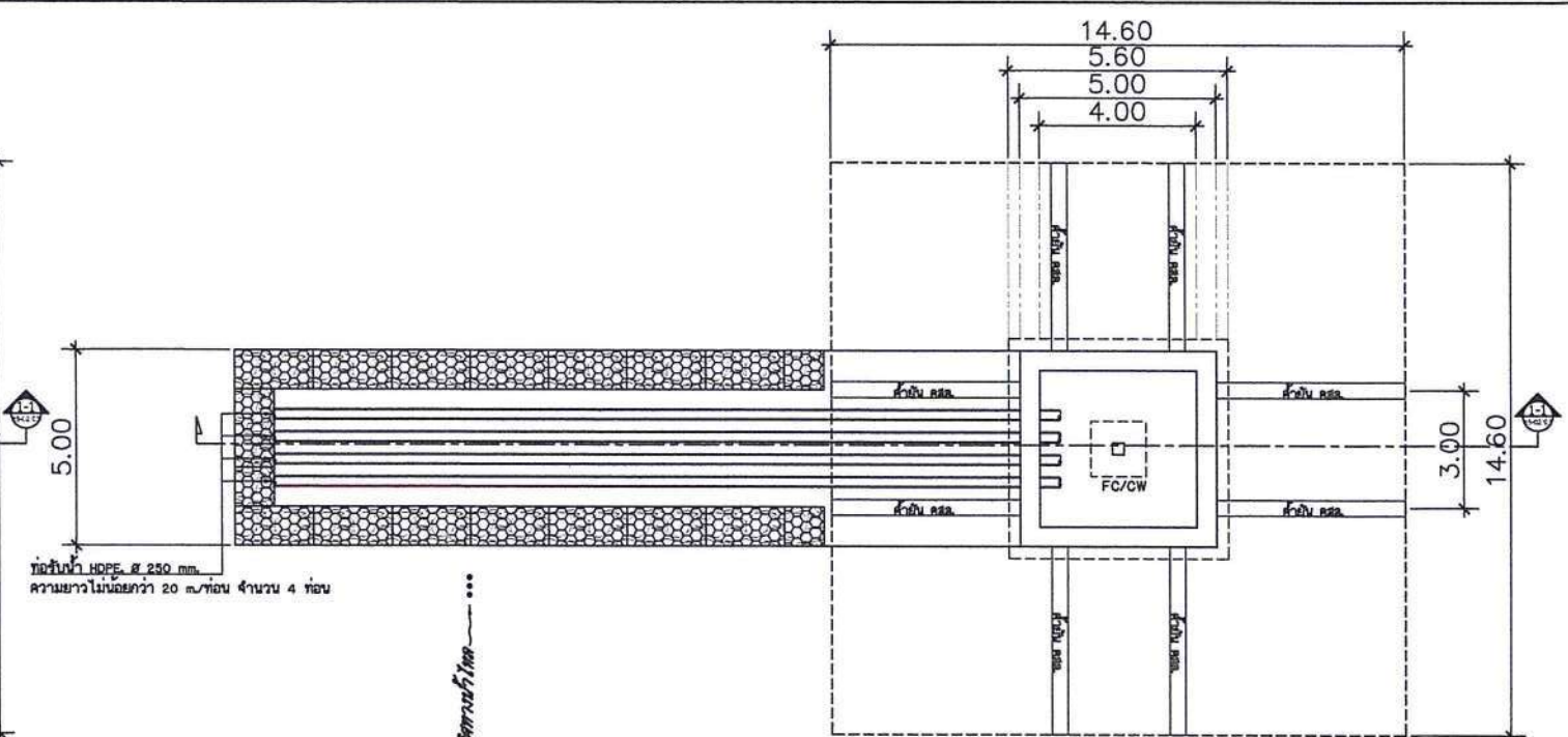
แปลนเสาและฐานราก
