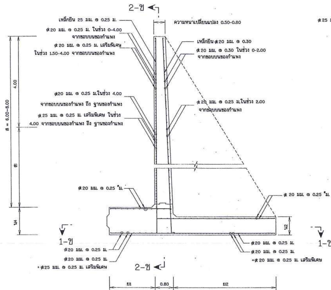
รูปตัด 2-2 (ที่กึ่งกลางช่วง)
