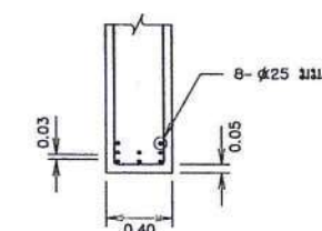
แบบขยาย 1 มาตรา 1:25
