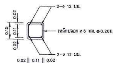
รายละเอียดการติดตั้งเสาป้าย มาตราส่วน 1:20
