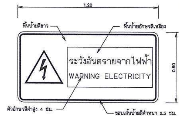
ป้ายเตือนกระแสไฟฟ้า ไม่แสดงมาตราส่วน
