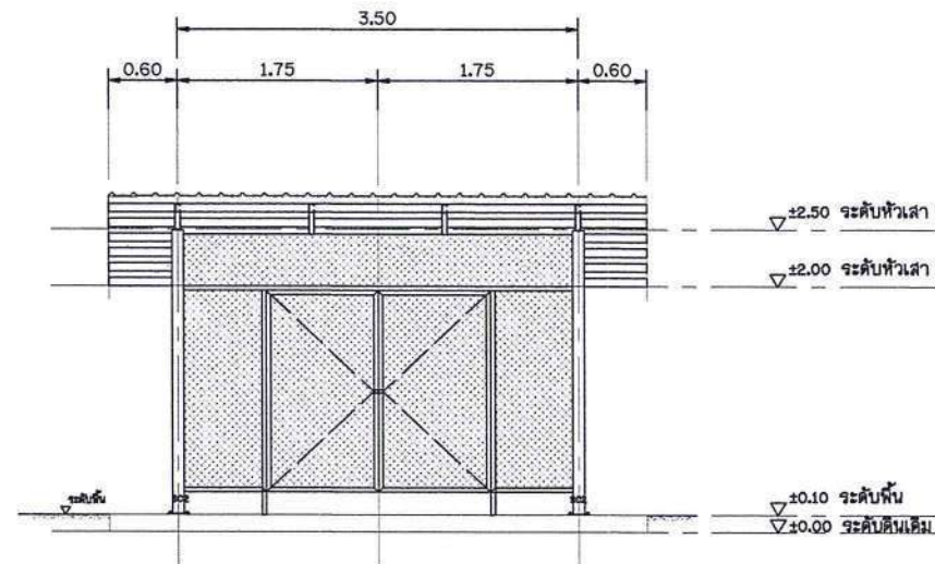
รูปด้าน 1
