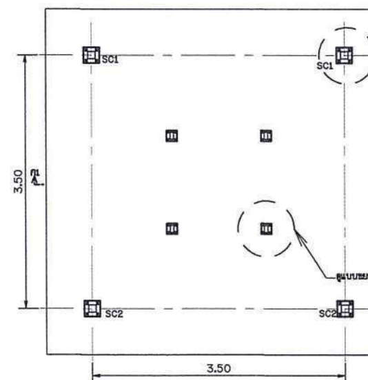
แปลนเสาอาคารโรงสูบน้ำ
