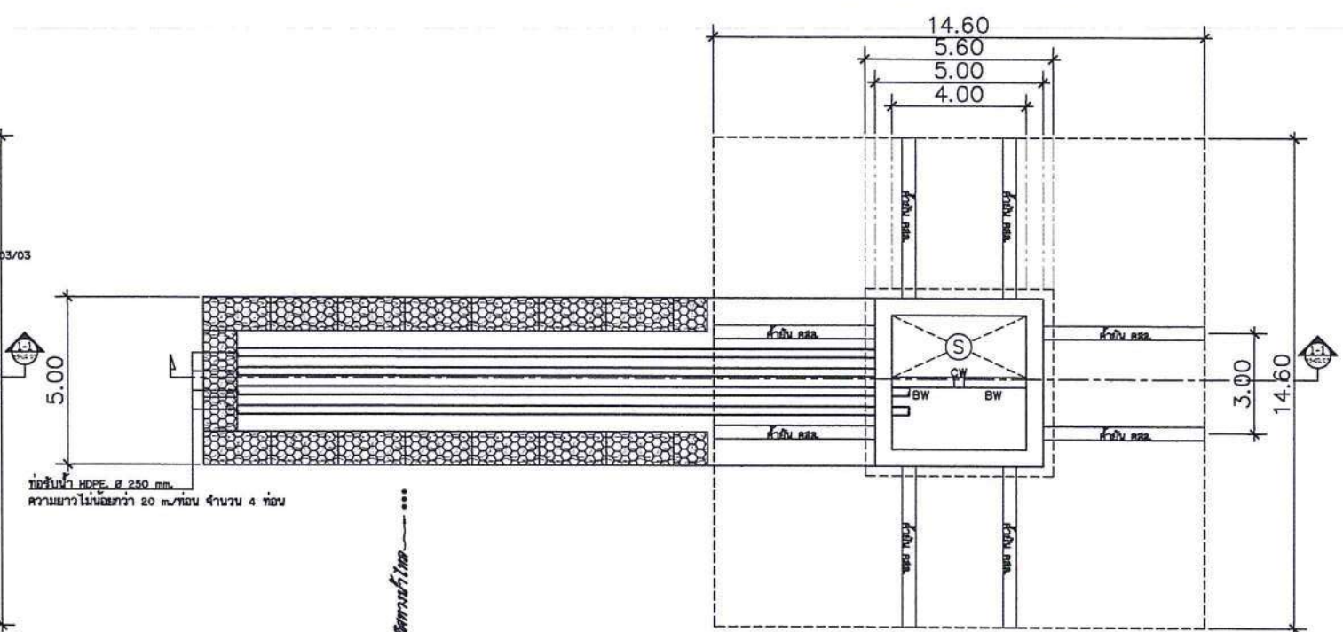
แปลนแสดงโครงสร้างคานและพื้นสำหรับปั้มสูบน้ำ
