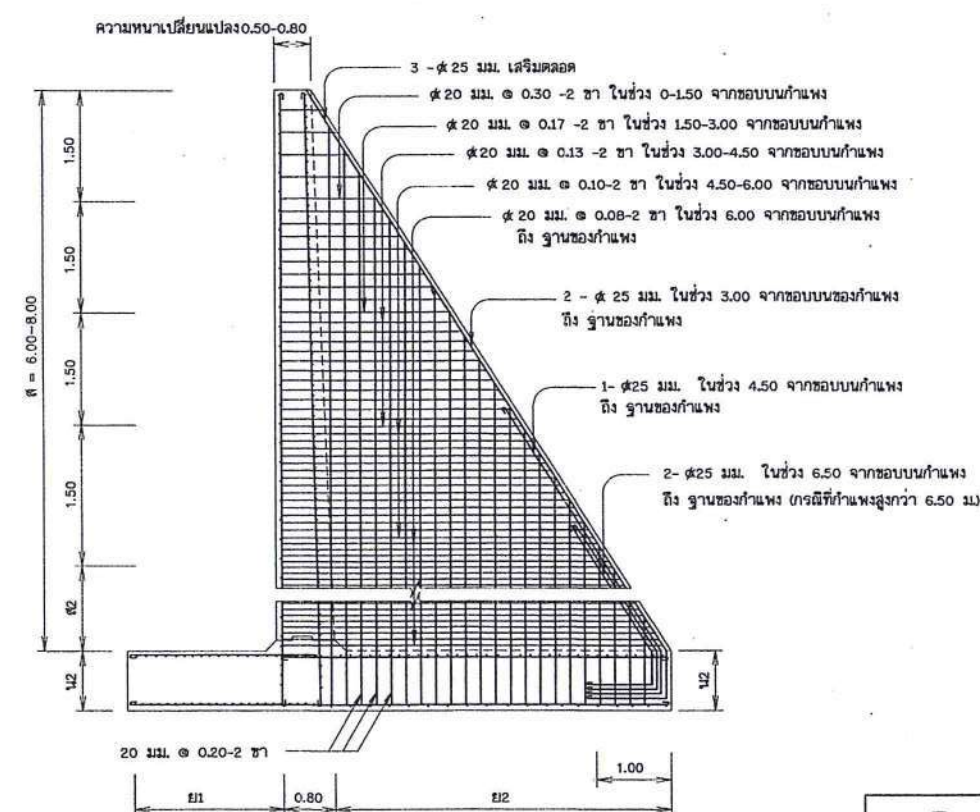
แบบแสดงการเสริมเหล็กในค้ำยัน
