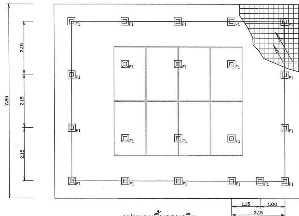
รูปขยายพื้นคอนกรีต
