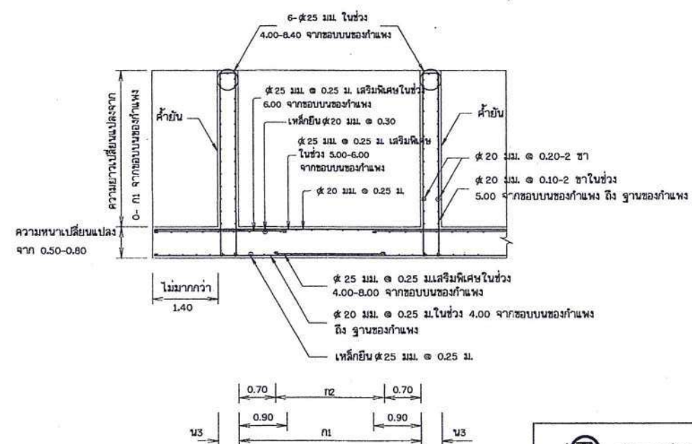
รูปตัด 3-3
