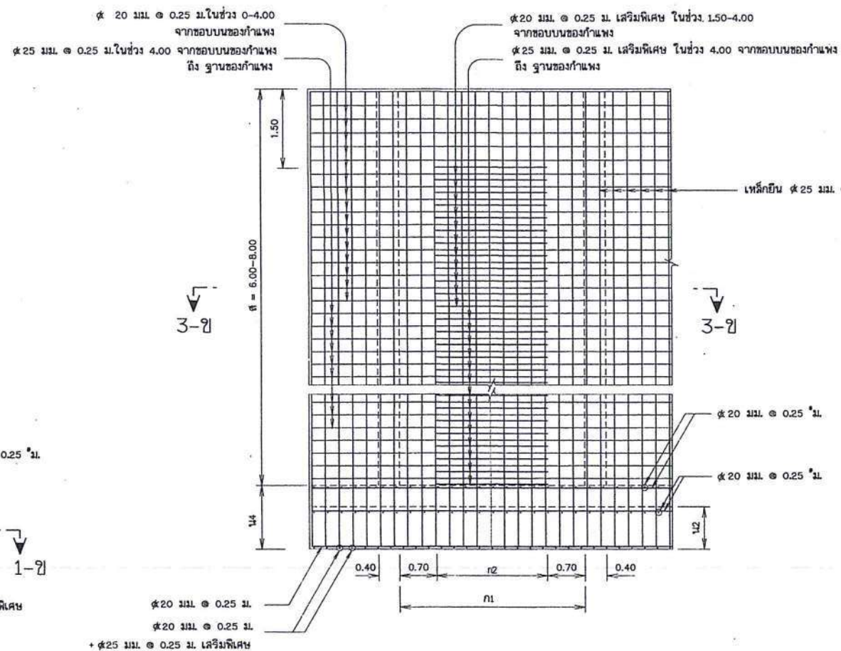
รูปตัด 2-2 (ด้านไม่ติดดิน)
