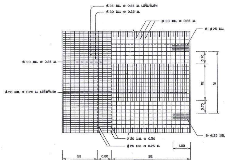
รูปตัด 1-1 (พื้นด้านล่าง)
