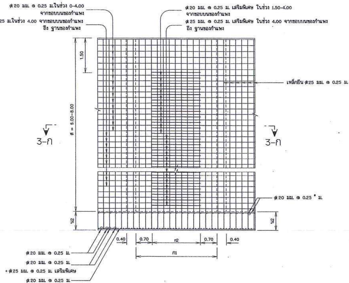
รูปตัด 2-ก (ด้านไม่ติดดิน)
