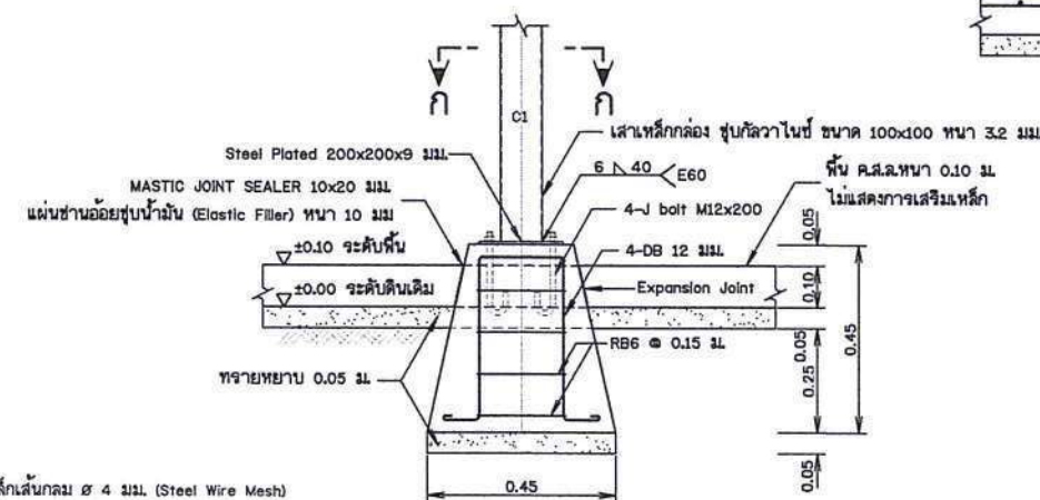
รูปขยายฐานรากโครงสร้างรับแผง F1 (ต่อม่อ คสล. หล่อสำเร็จรูปพร้อมติดตั้ง)
