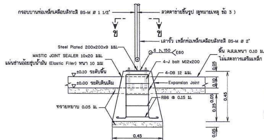
รูปขยายฐานรากโครงสร้างรับแผง F1 (คอม่อ คสล. หล่อสำเร็จรูปพร้อมติดตั้ง) ไม่แสดงมาตราส่วน
