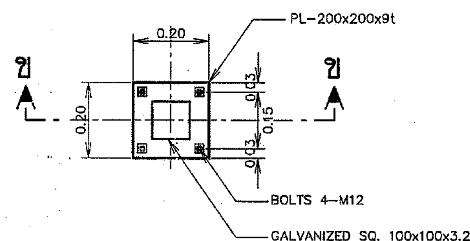
แบบขยายเสา
