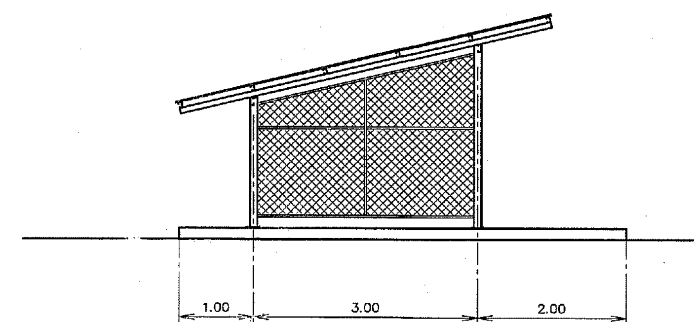
รูปด้านข้างอาคาร
