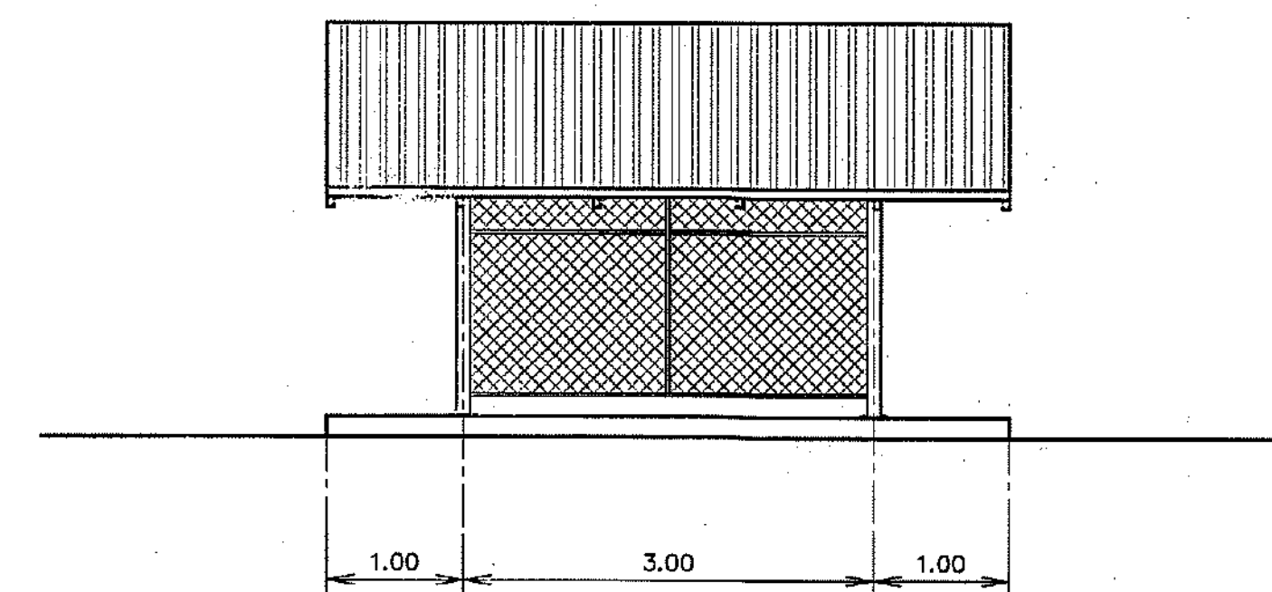
รูปด้านหลังอาคาร
