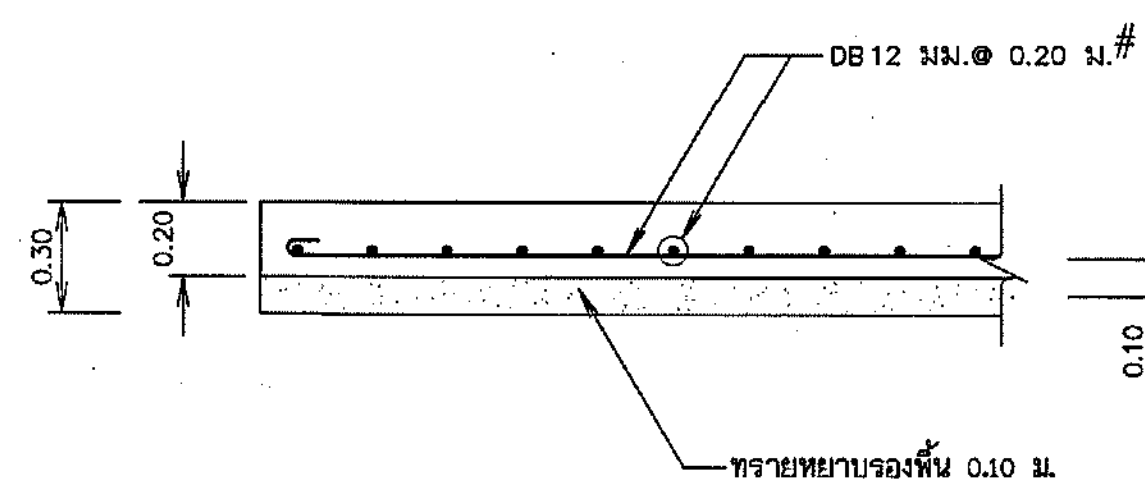
ขยายพื้น
