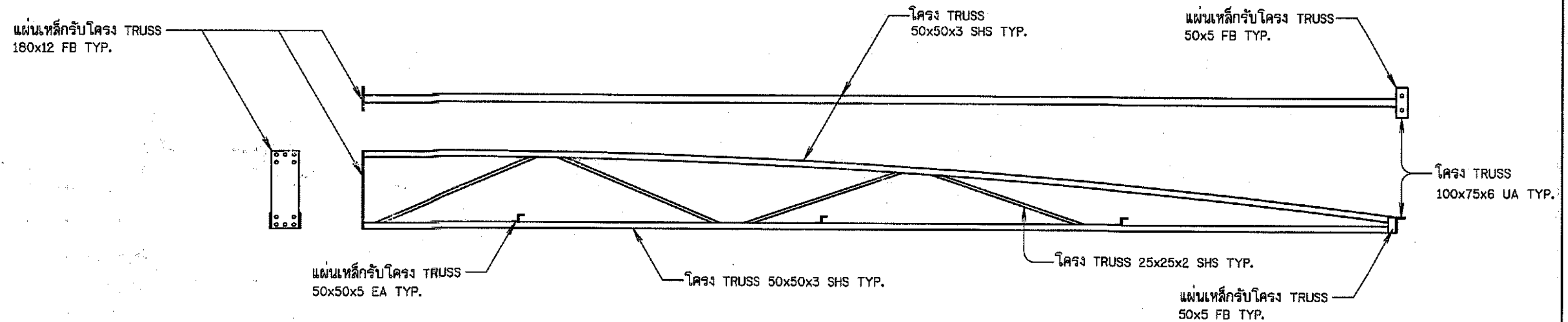
แบบขยาย 5 รูปตัดโครงเหล็กหลักทั่วไป
