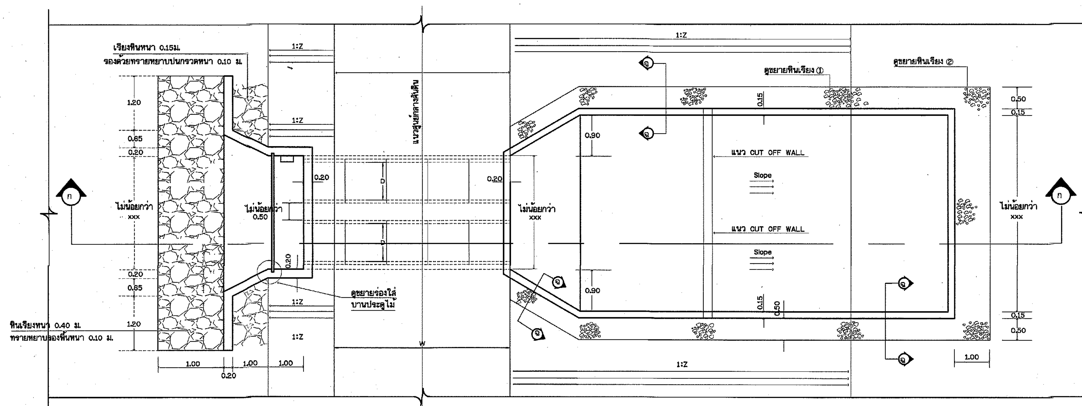
แปลนอาคารทางน้ำเข้า ไม่แสดงขนาดจาล้วน
