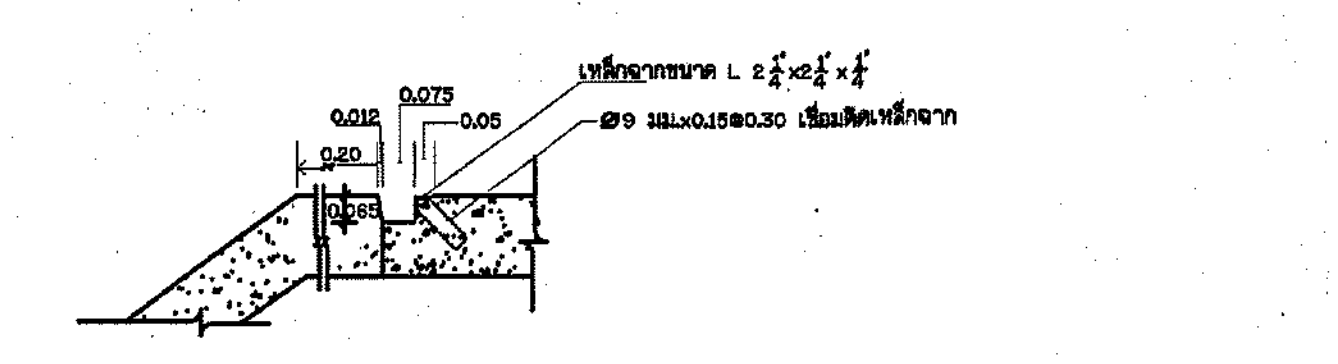
ขยายร่องใส่บานประตูไม้ ไม่แสดงขนาดจาล้วน
