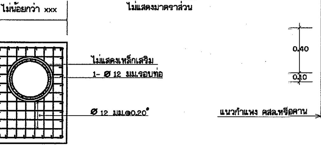
ขยายการเสริมเหล็กกำแพงปากท่อและท้ายท่อ (HEAD WALLS) ไม่แสดงขนาดจาล้วน
