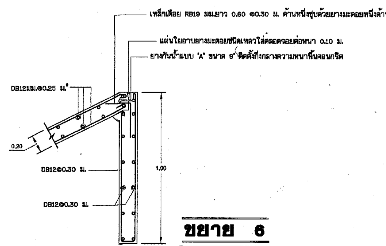
รูปขยายระบายน้ำกำแพงลาดเอียง ไม่ปรับไปตามขนาดจริง
