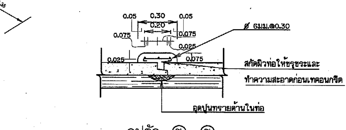
รูปตัด ข-ข ไม่แสดงขนาดจาล้วน
