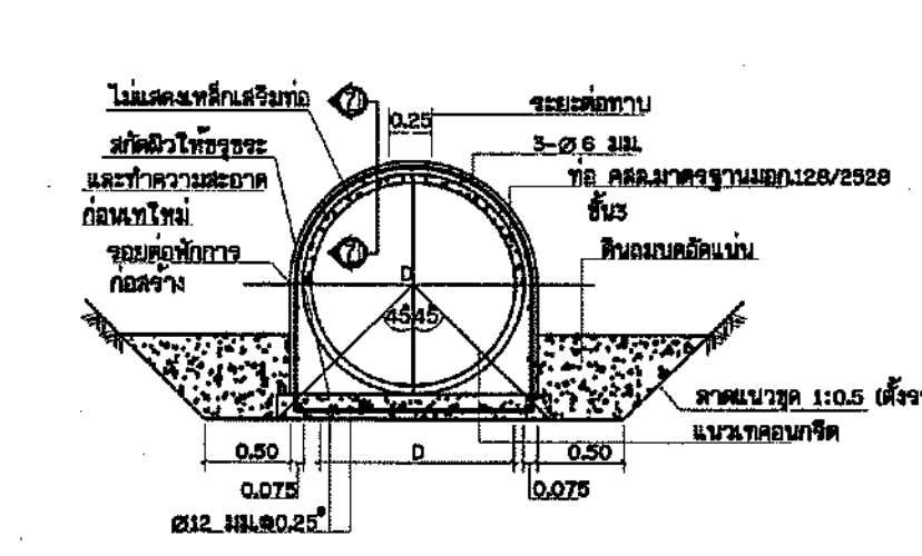
รูปตัดการวางท่อ คสล. ไม่แสดงขนาดจาล้วน
