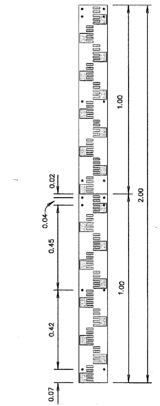
แผนเหล็กบอกระดับน้ำ มาตรฐาน 1:100
