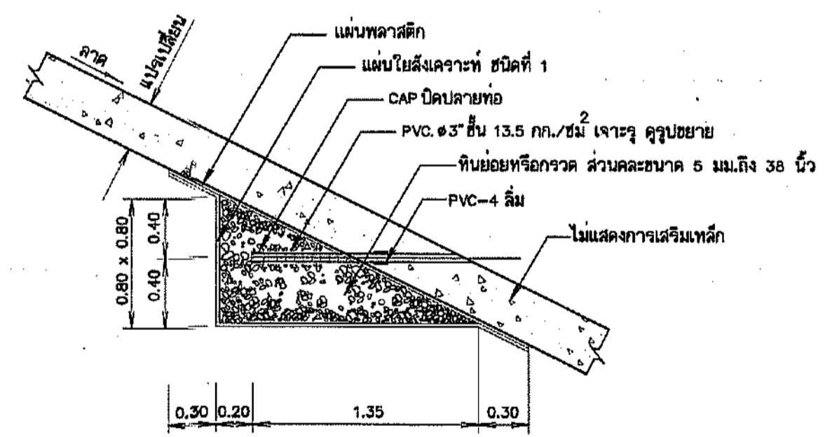
รูปขยายระบายน้ำกำแพงลาดเอียง ไม่ปรับไปตามขนาดจริง
