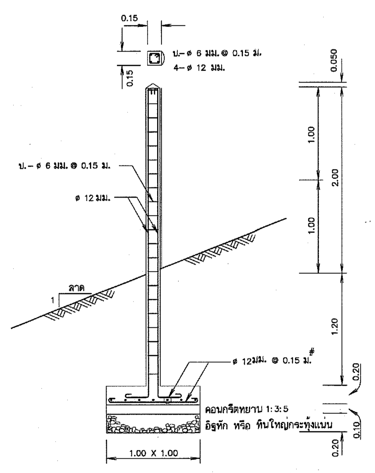
ขยายหลัก คสล.บอกระดับน้ำ มาตรฐาน 1:25
