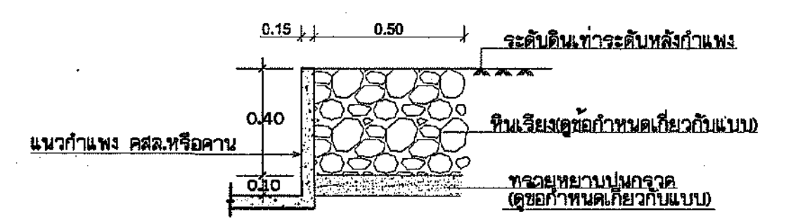
ขยายหินเรียง 1 ไม่แสดงขนาดจาล้วน
