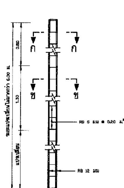
รายละเอียดเส้าท้าย คสล.
