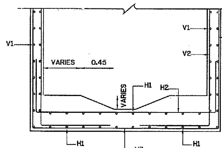
รูปตัด (ค) NOT TO SCALE
