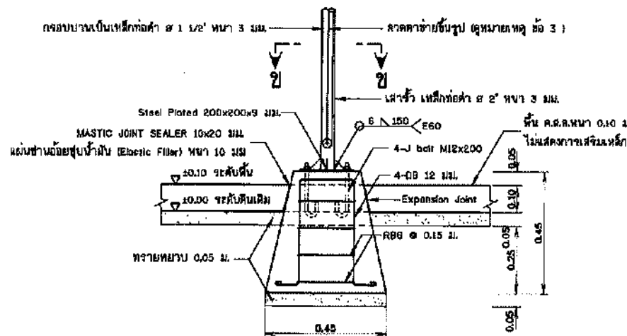
รูปขยายฐานรากโครงสร้างรับแผง F1 คคคค คคค, หลอดน้ำแรงดันพร้อมติดตั้ง ไม่แสดงขนาดบางส่วน
