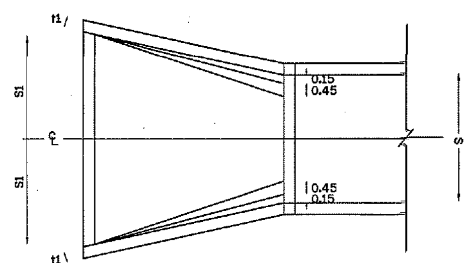
รูปตัด (ก) NOT TO SCALE
