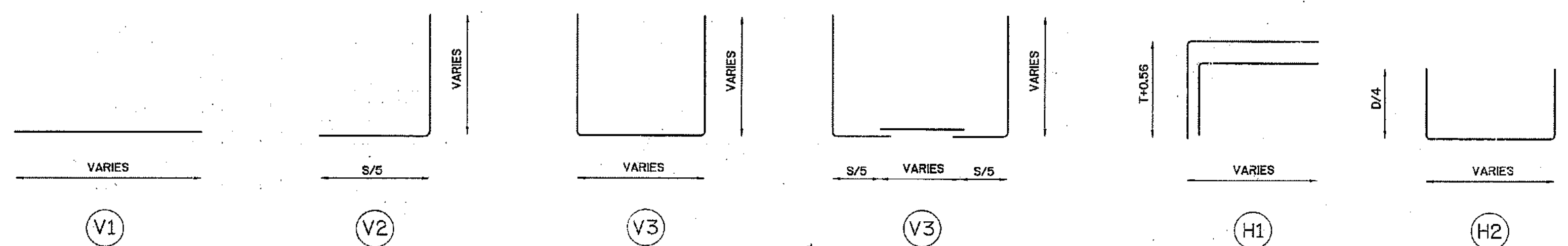
รายละเอียดเหล็กเสริม NOT TO SCALE
