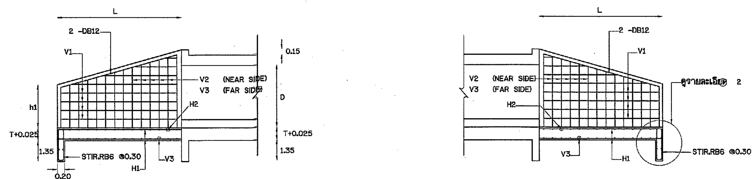
รูปตัด (ก) NOT TO SCALE
