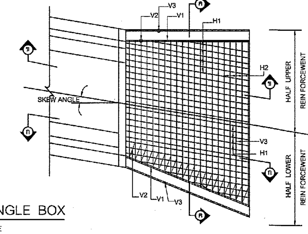
รูปตัด ⑥ NOT TO SCALE
