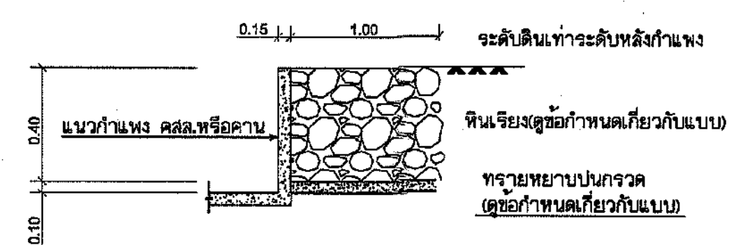
ขยายพื้นเรียบ 1 ไม่แสดงมาตราส่วน
