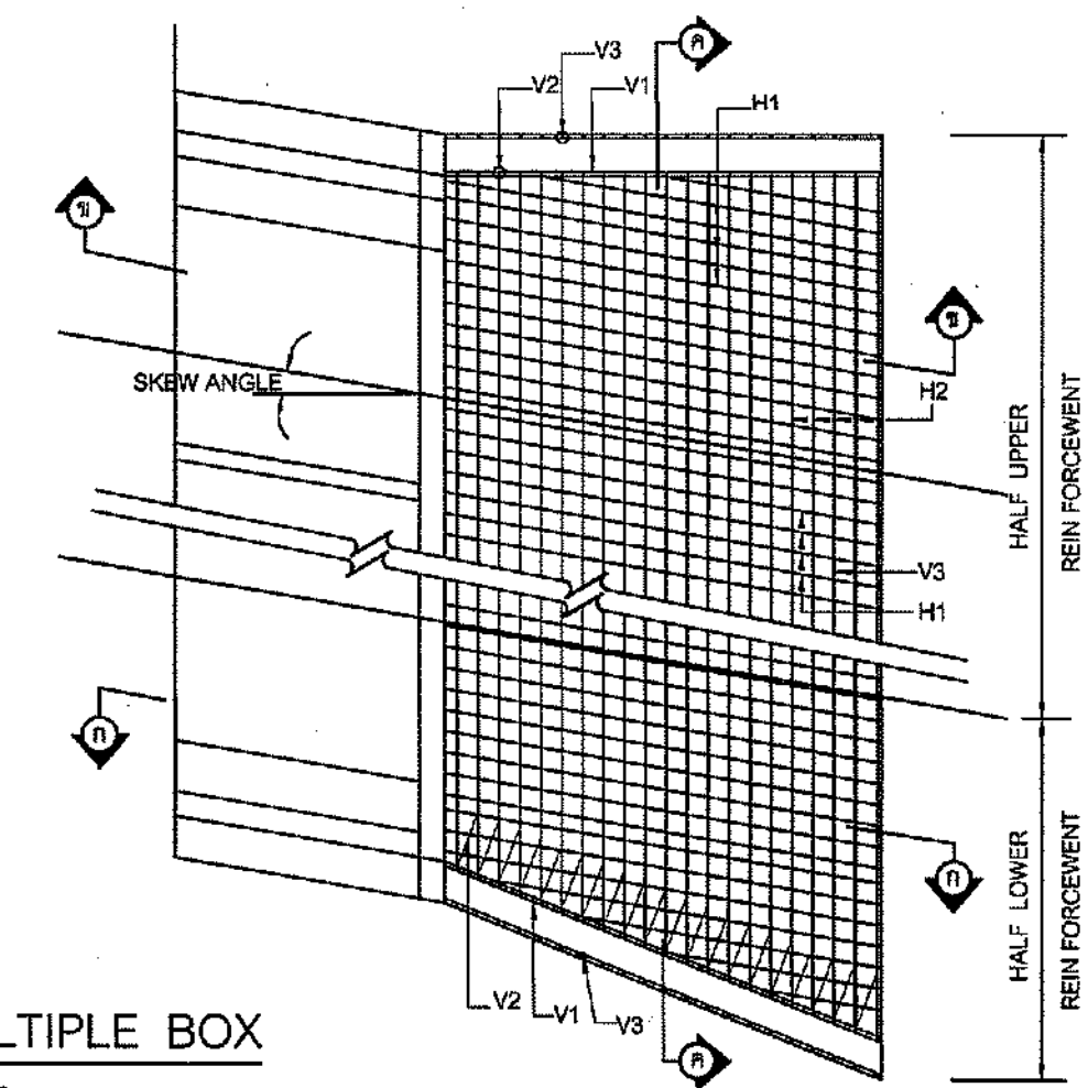
รูปตัด ⑧ NOT TO SCALE
