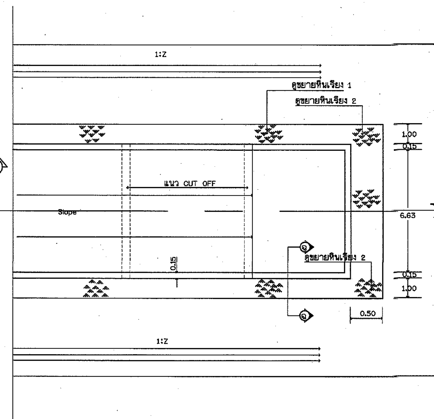
แปลนอาคารวาง Chute (กรณีไม่มีชานพัก) ไม่แสดงมาตราส่วน
