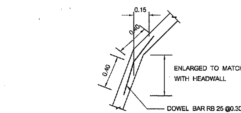
รูปตัด ① NOT TO SCALE
