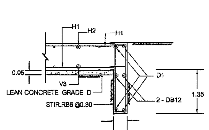
รูปตัด ② NOT TO SCALE
