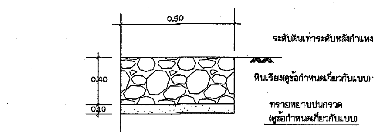
ขยายพื้นเรียบ 2 ไม่แสดงมาตราส่วน
