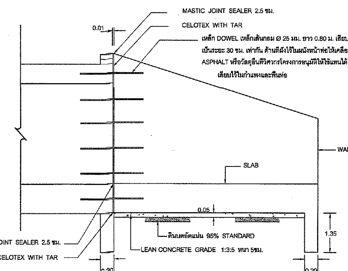
รูปตัด ⑤ NOT TO SCALE
