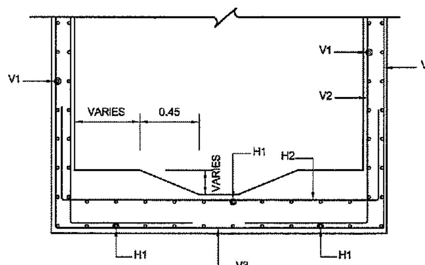
รูปตัด ④ NOT TO SCALE
