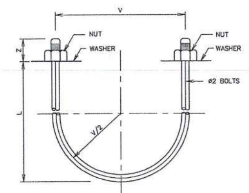
มาตรฐานการงอ U - BOLT ไม่แสดงมาตราส่วน
