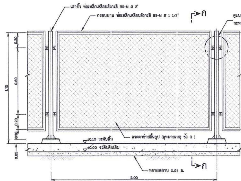
แบบขยาย ๕ รวดตาข่าย
