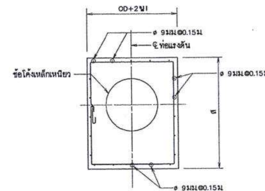
รูปตัด ช-ช ไม่แสดงมาตราส่วน
