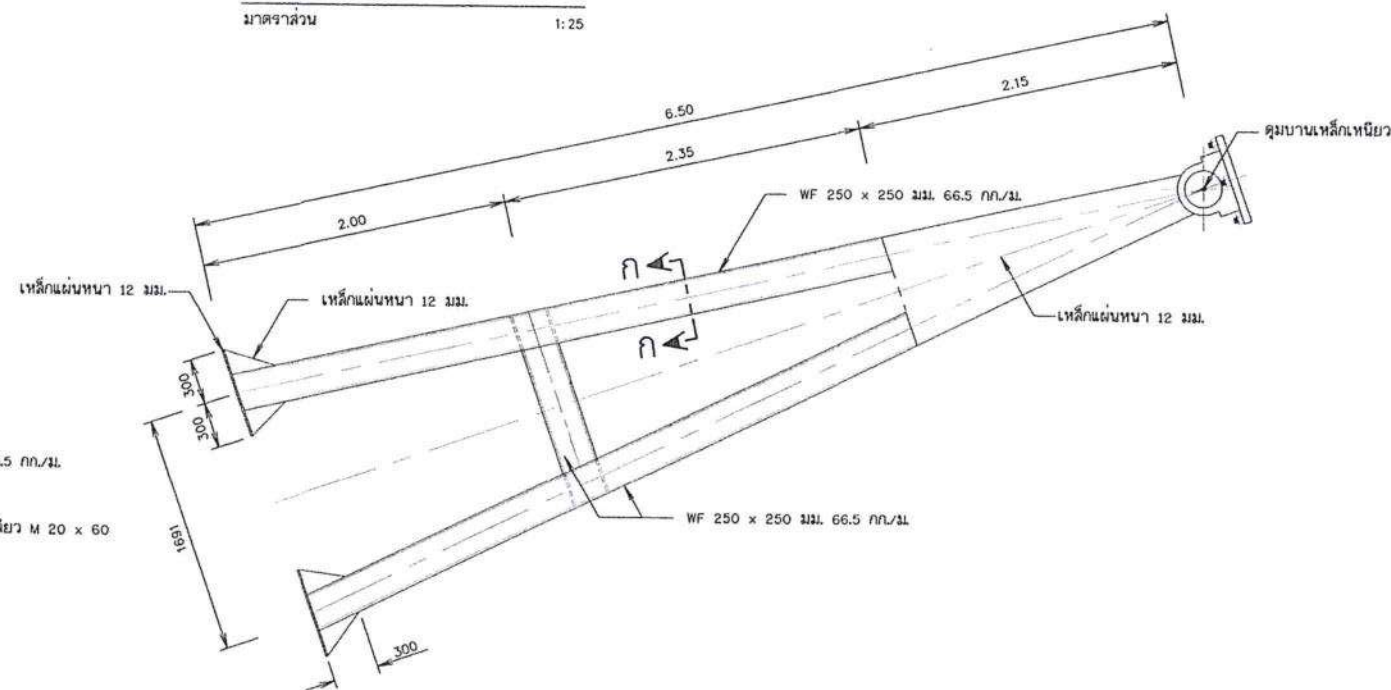
แปลนแขนบาน
