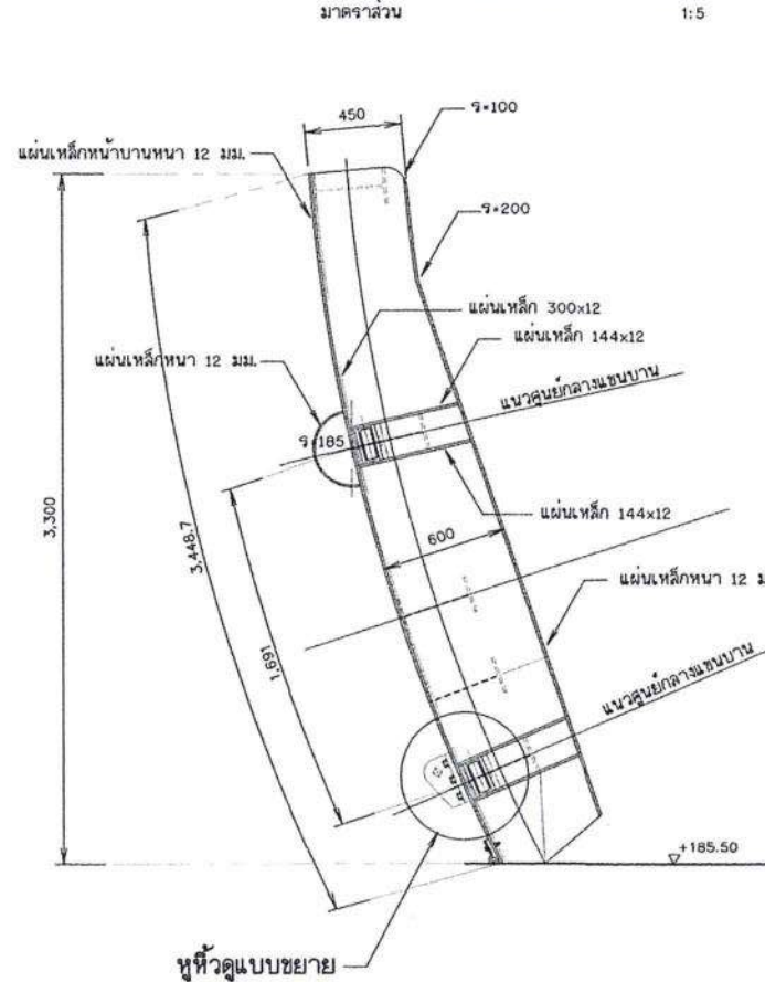
รูปตัด SIDE BEAM
