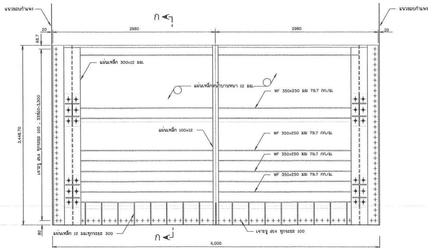
รูปบานประตูด้านท้ายน้ำ
