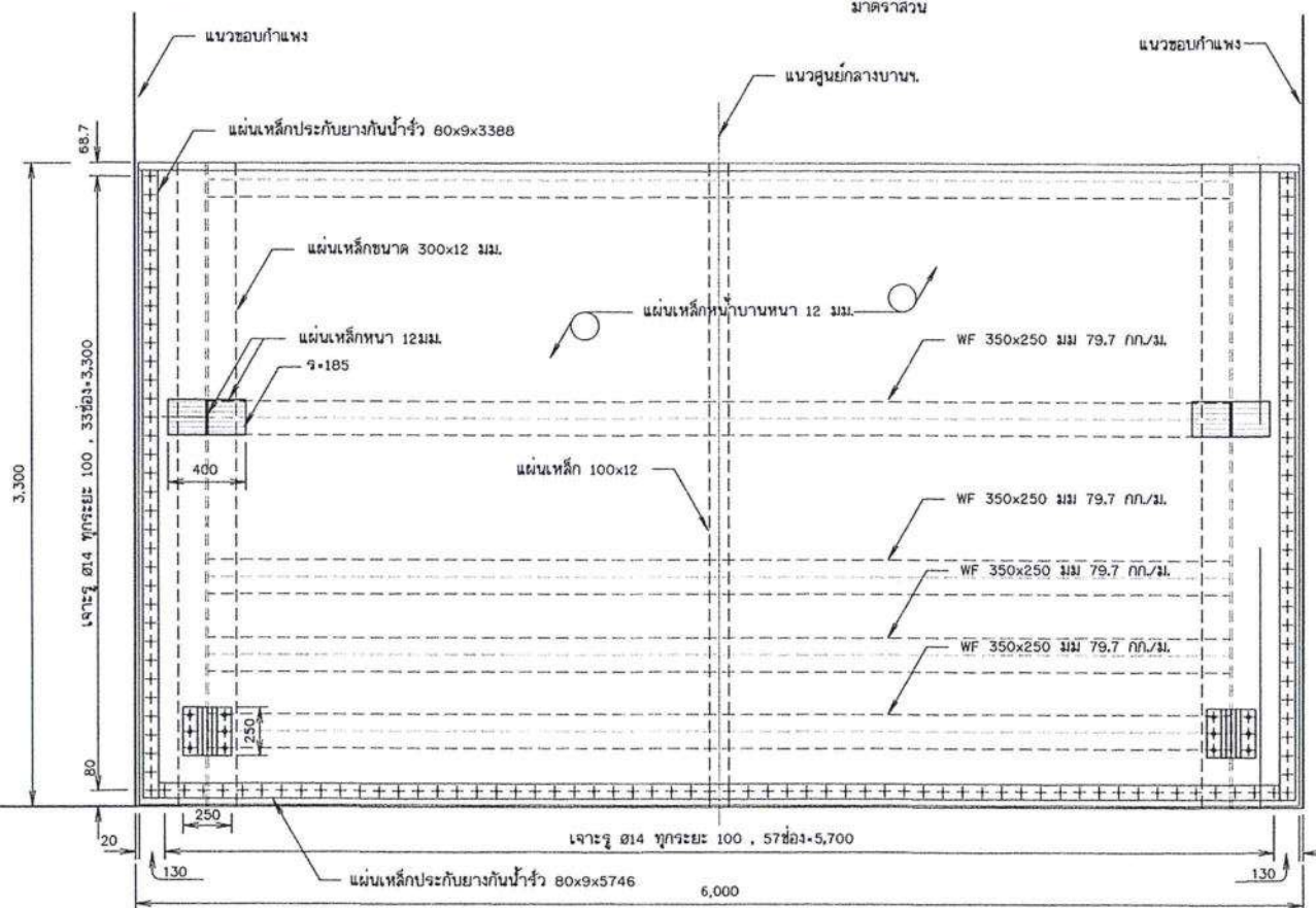
การติดตั้งยางกันน้ำรูด้านข้างและ SIDE ROLLER
