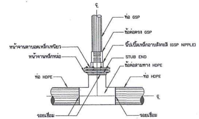
การบรรจุท่อสามทาง HDPE กับท่อ GSP แบบข้อต่อ (สำหรับอาคารจุดปล่อยน้ำ อาคารประจวบฯ อาคารท่อระบายอากาศ กรณีท่อส่งน้ำขนาดเส้นผ่าศูนย์กลางมากกว่า 315 มม.)
