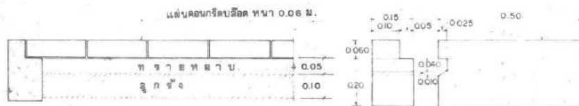
ขยายคันท่อนกริด 1810
