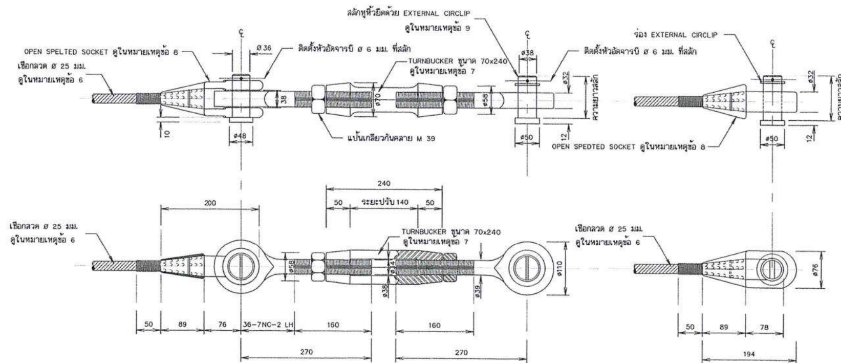
แบบแสดงรายละเอียด TURNBUCKLE กับหูหิ้ว
