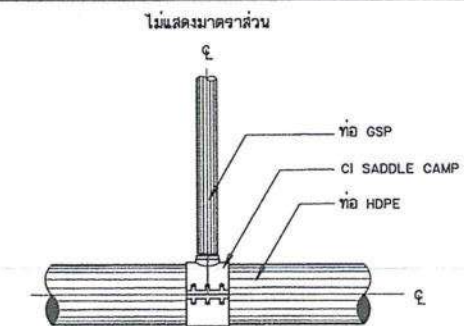
การบรรจุท่อสามทาง HDPE กับท่อ GSP แบบ CI SADDLE CLAMP (สำหรับอาคารจุดปล่อยน้ำ อาคารประจวบฯ อาคารท่อระบายอากาศ กรณีท่อส่งน้ำขนาดเส้นผ่าศูนย์กลางน้อยกว่าหรือเท่ากับ 315 มม.)
