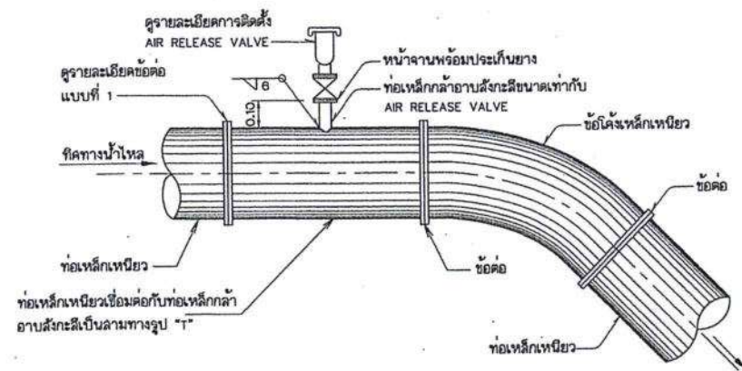
AIR RELEASE VALVE บนท่อลงน้ำขามห้วย ไม่แสดงมาตราส่วน
