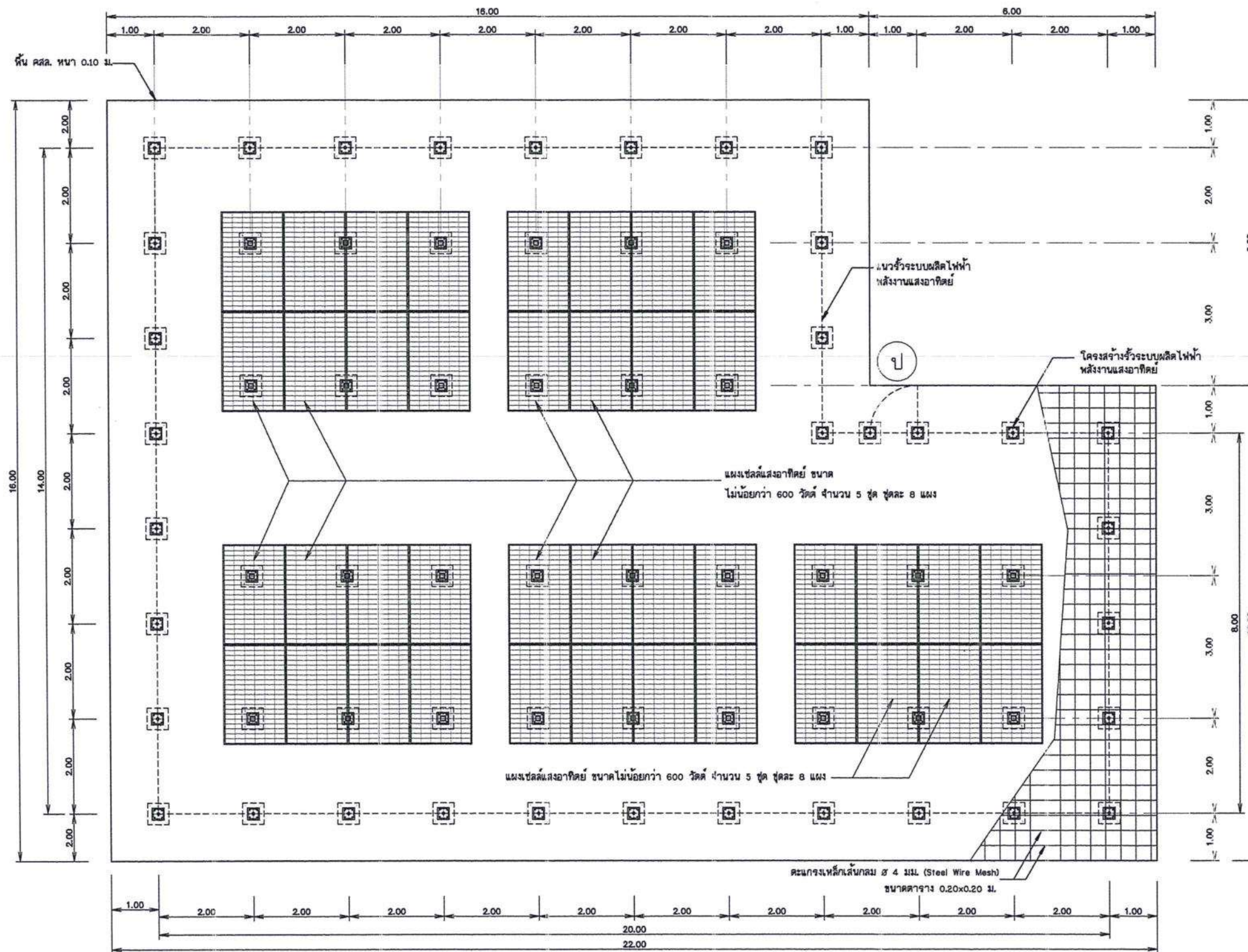
แปลนการติดตั้งแผงเซลล์แสงอาทิตย์ พร้อมรั้ว รูปขายพื้นคอนกรีต ไม่มีภาคส่วน
