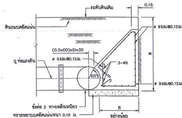
รูปตัด ข-ข ไม่แสดงขนาดบางส่วน
