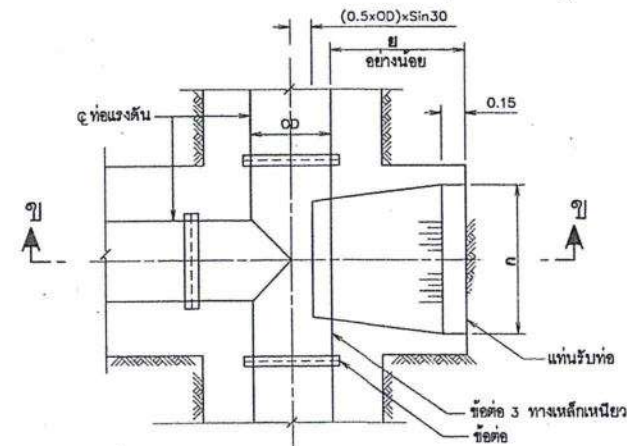
แบบแปลน ไม่แสดงขนาดบางส่วน
