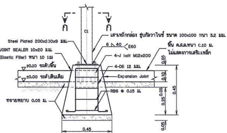
(ต่อม่อ คสล. หล่อสำเร็จรูปพร้อมติดตั้ง)
