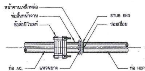
การบรรจุท่อ AC กับท่อ HDPE ไม่แสดงขนาดบางส่วน
