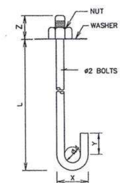
มาตรฐานการงอ HOOKED BOLT ไม่แสดงมาตราส่วน
