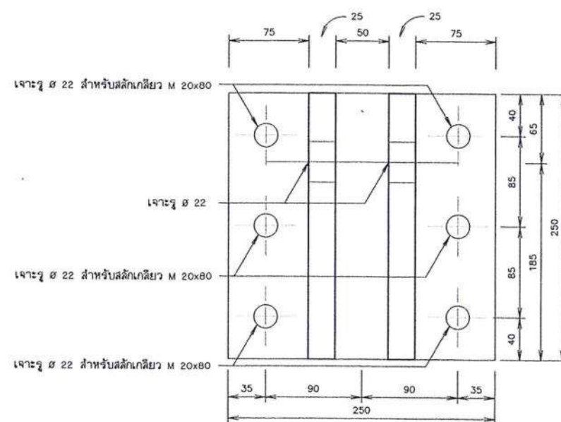
แบบแสดงรายละเอียด TURNBUCKLE กับหูหิ้ว
