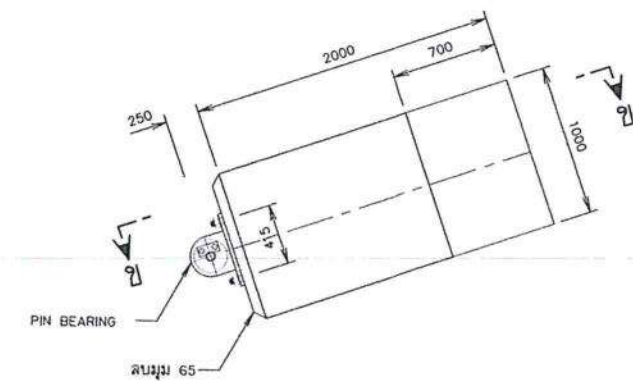
แท่น ค.ส.ล.รับ PIN BEARING
