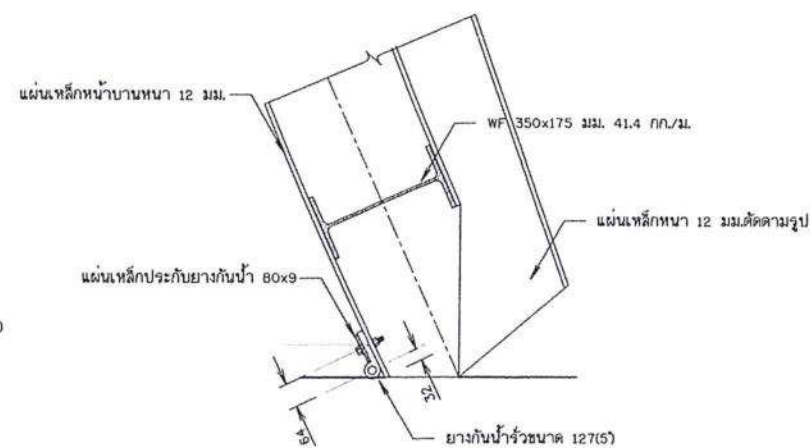
แบบขยายยางกันน้ำใต้บาน
