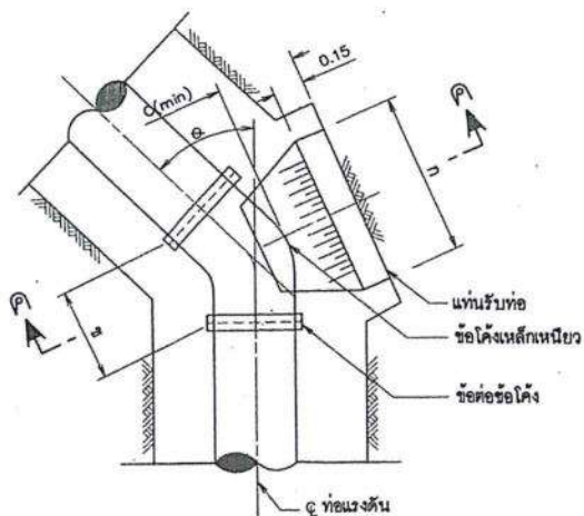
แบบแปลน ไม่แสดงขนาดบางส่วน
