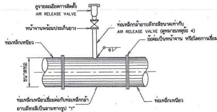
รายละเอียดข้อต่อแบบที่ 1 (กรณีท่อลงน้ำเป็นท่อเหล็กเหนียว) ไม่แสดงมาตราส่วน
