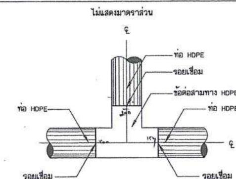
การบรรจุท่อสามทาง HDPE กับท่อ HDPE ไม่แสดงขนาดบางส่วน
