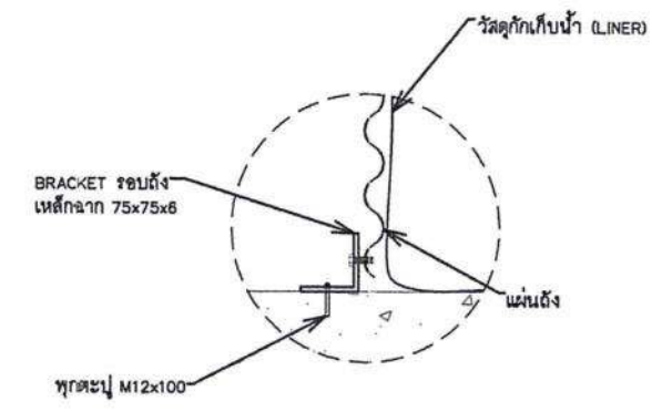
แบบขยาย 10 ติดตั้งผนังกับฐานราก Scale NTC
