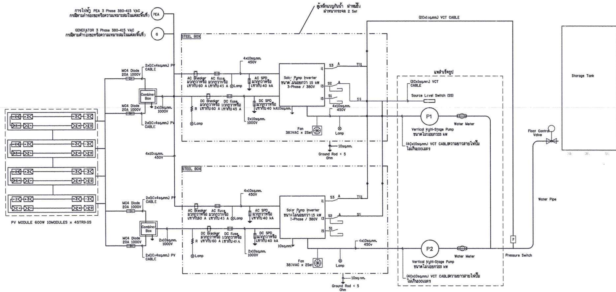
แผนผังระบบไฟฟ้า และไดอะแกรมไฟฟ้า ระบบกระจายน้ำด้วยพลังงานแสงอาทิตย์ ขนาด 13 กิโลวัตต์
