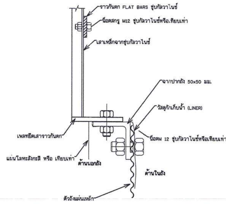
แบบขยาย 8 Scale NTC
