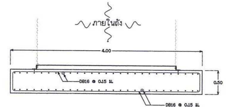
แบบขยาย ฐานจาก ขนาด 4.00x4.00x0.50 ม. Scale NTC
