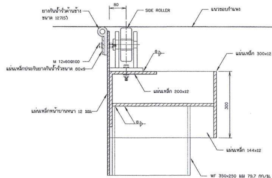
การติดตั้งยางกันน้ำรูด้านข้างและ SIDE ROLLER
