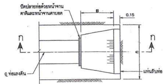
แบบแปลน ไม่แสดงขนาดบางส่วน
