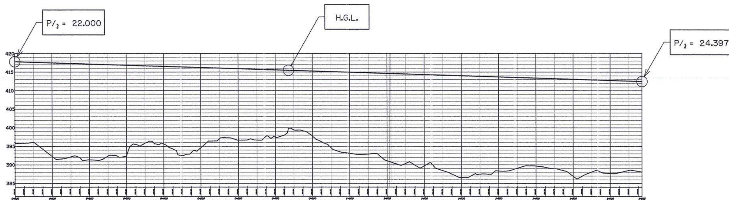
รูปตัดตามแนวยาวแสดง H.G.L. สาย RMP STA. 0+000 - 1+685 ไม่แสดงมาตราส่วน
