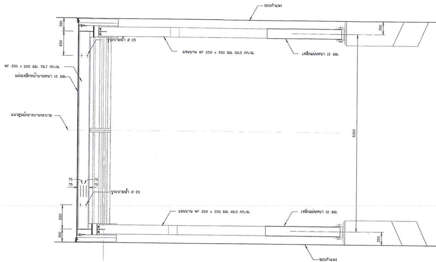
แปลนแขนบาน
