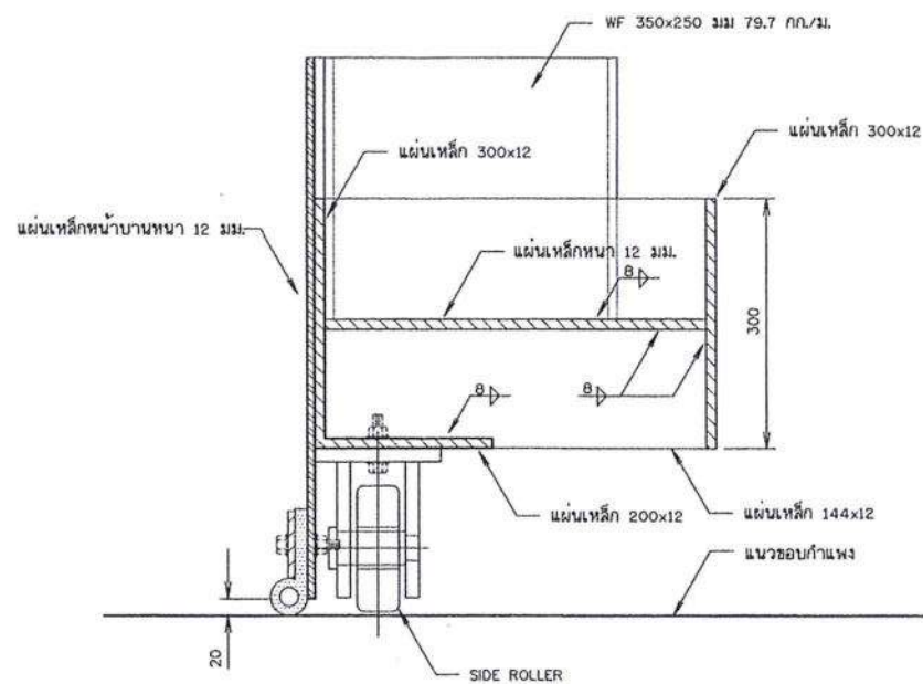
รูปตัด SIDE BEAM
