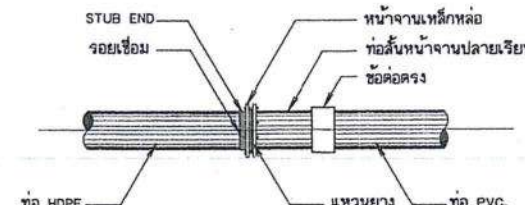
การบรรจุท่อ HDPE กับท่อ PVC. ไม่แสดงขนาดบางส่วน
