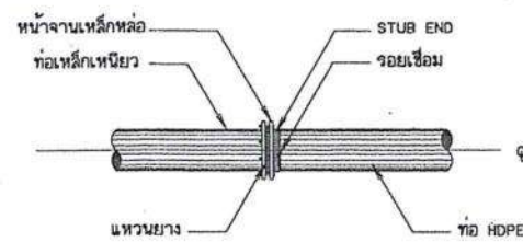
การบรรจุท่อเหล็กเหนียวกับท่อ HDPE ไม่แสดงขนาดบางส่วน
