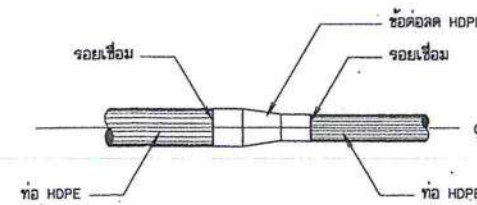
การบรรจุท่อ HDPE กับข้อต่อท่อ HDPE ไม่แสดงขนาดบางส่วน
