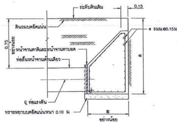
รูปตัด ก-ก ไม่แสดงขนาดบางส่วน
